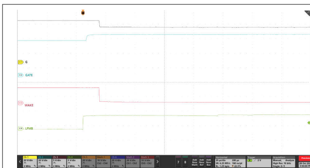
图 9-6. 从 LPM 到工作模式的状态转换 (LPM = 低电平到高电平, VIN = 48V, 无负载)
