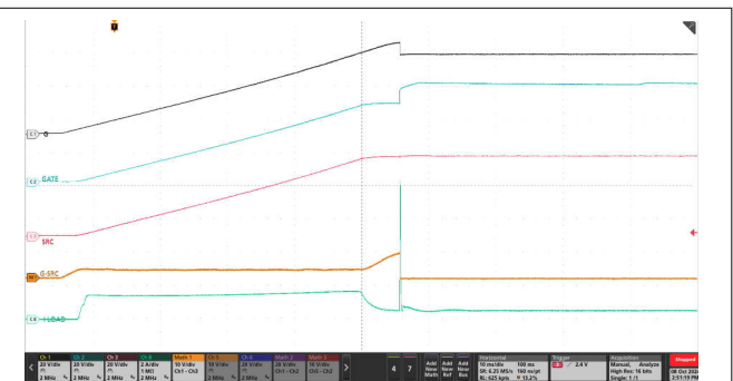
图 9-18. 输出端为 1000\mu F 且负载为 0.5A 时的浪涌电流曲线 (LPM = 低电平)
