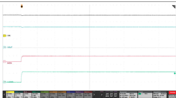
图 9-13. TPS4812-Q1 电流监测输出 (IMON) 瞬态响应
