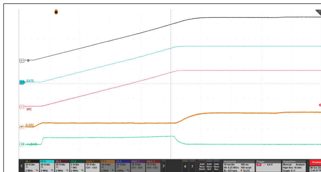
图 9-17. 输出端为 1000\mu F 时的浪涌电流曲线 (LPM = 低电平)
