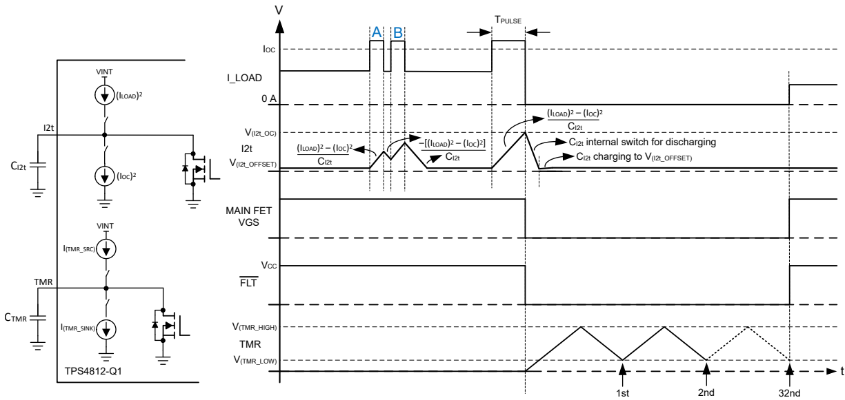
图 8-9. 具有自动重试功能的 I^2t 过流保护
