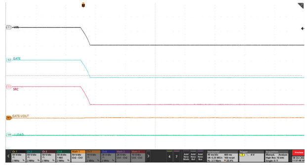
图 9-15. 输入电池反向故障下的 GATE 关断
