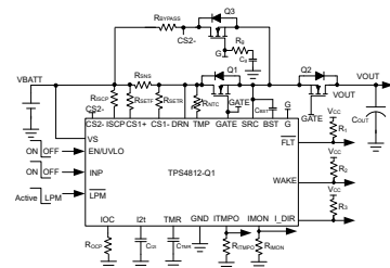
驱动 PAAT 负载、具有负载唤醒和大容量电容器充电功能的 TPS4812-Q1 应用电路
