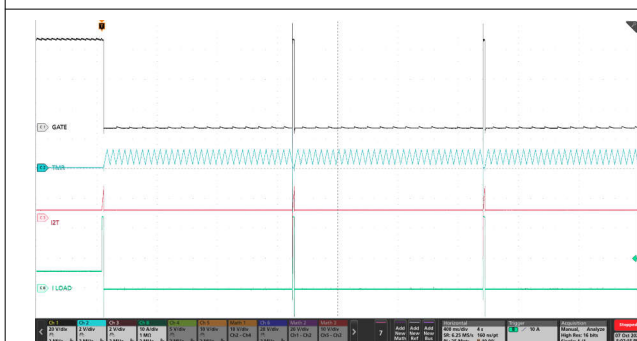
图 9-10. TPS4812-Q1 在 I 2 t 过流故障下的自动重试响应
