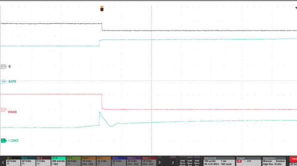
图 9-4. 从 LPM 到工作模式的状态转换放大视图 ( \overline{LPM} = 低电平， V_{IN} = 48V ， EN/UVLO = 高电平)
