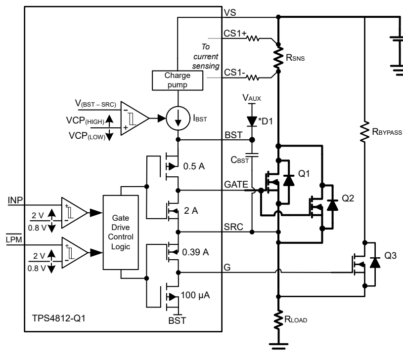
图 8-1. 栅极驱动器
