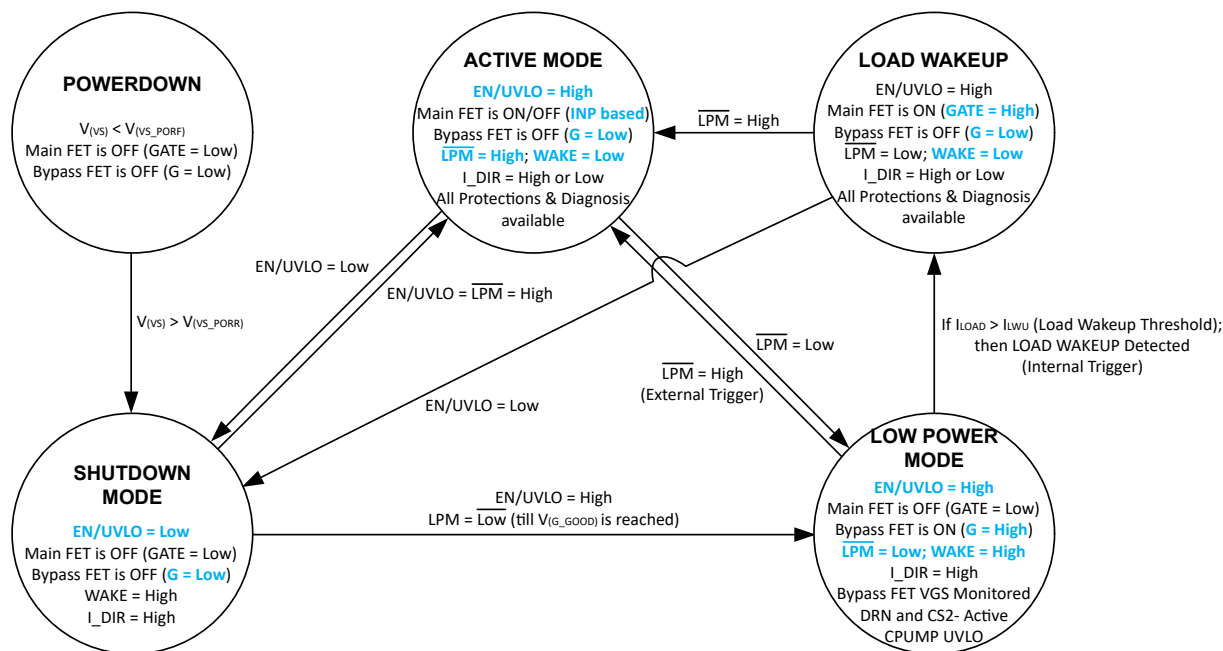
图 8-14. 状态图
