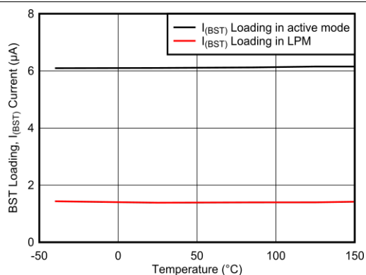
图 6-5. 电荷泵电流与温度间的关系
