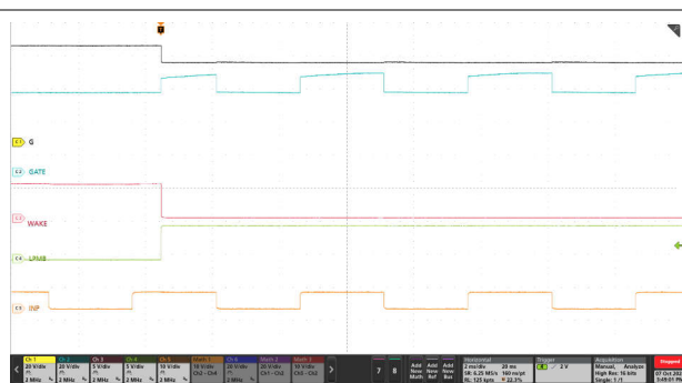
图 9-7. 当 LPM = 低电平到高电平时, INP 获得对 GATE 的控制 (VIN = 48V, 无负载)
