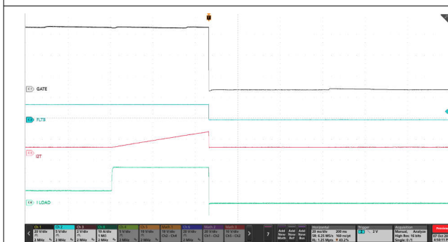
图 9-8. 6A 至 16A 负载阶跃下 TPS4812-Q1 EVM 基于 I 2 T 的过流响应
