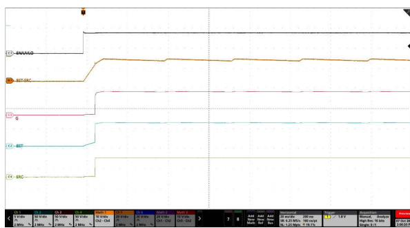
图 9-2. 低功耗路径的启动曲线 ( \overline{LPM} = 低电平， V_{IN} = 48V ，无负载， C_{BST} = 470nF )
