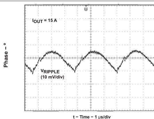
图 8-6. Output Voltage Ripple
