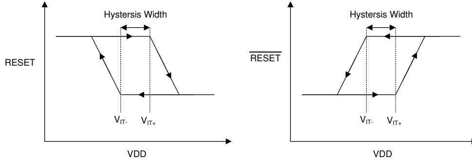
图 6-1. Hysteresis Diagram
