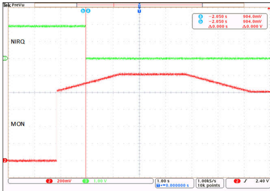
图 8-2. 发生过压故障后触发 NIRQ
