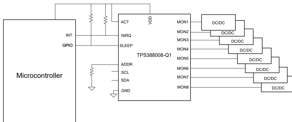
TPS38800 典型电路
