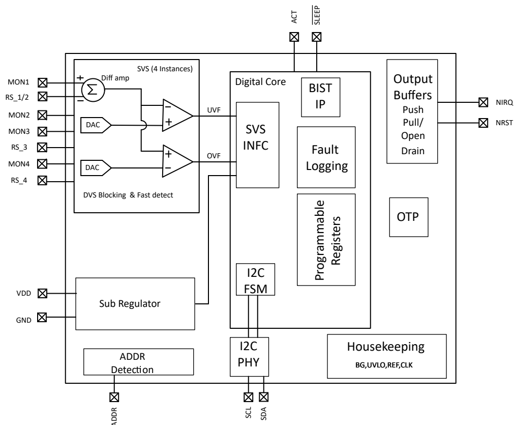
图 7-2. TPS388R04 方框图
