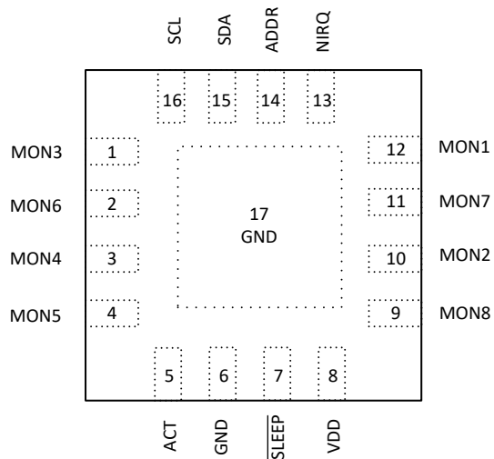
图 5-1. RTE 封装 16 引脚 WQFN TPS388008 顶视图
