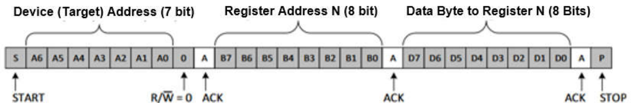
图 7-4. I 2 C 写入协议
