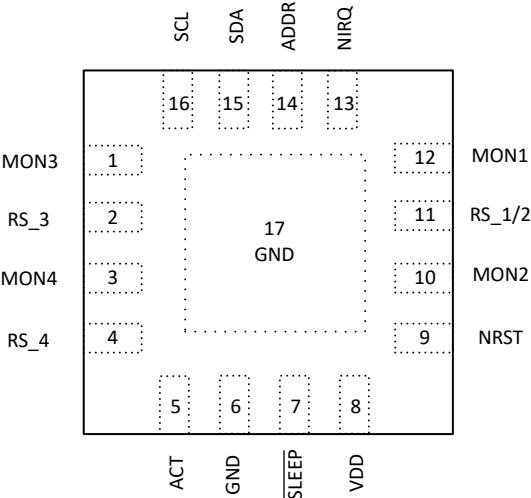
图 5-3. RTE 封装 16 引脚 WQFN TPS388R04 顶视图
