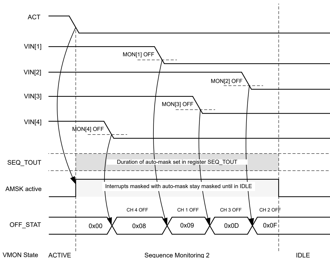
图 7-16. ACT 1→0 转换
