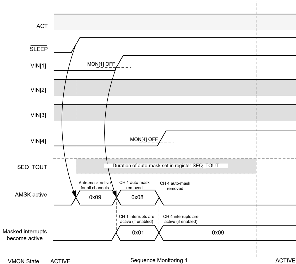
图 7-15. SLEEP 0→1 转换
