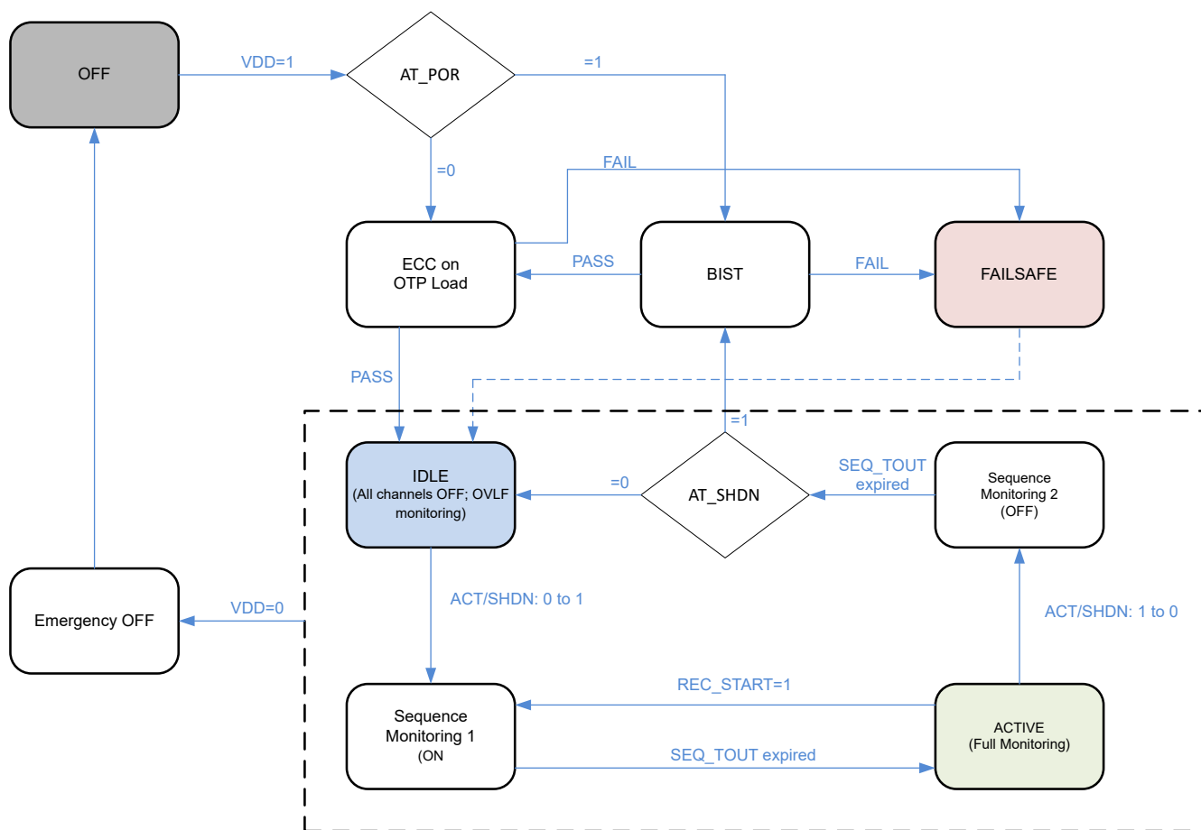
图 7-11. TPS38800/TPS388R0 状态图
