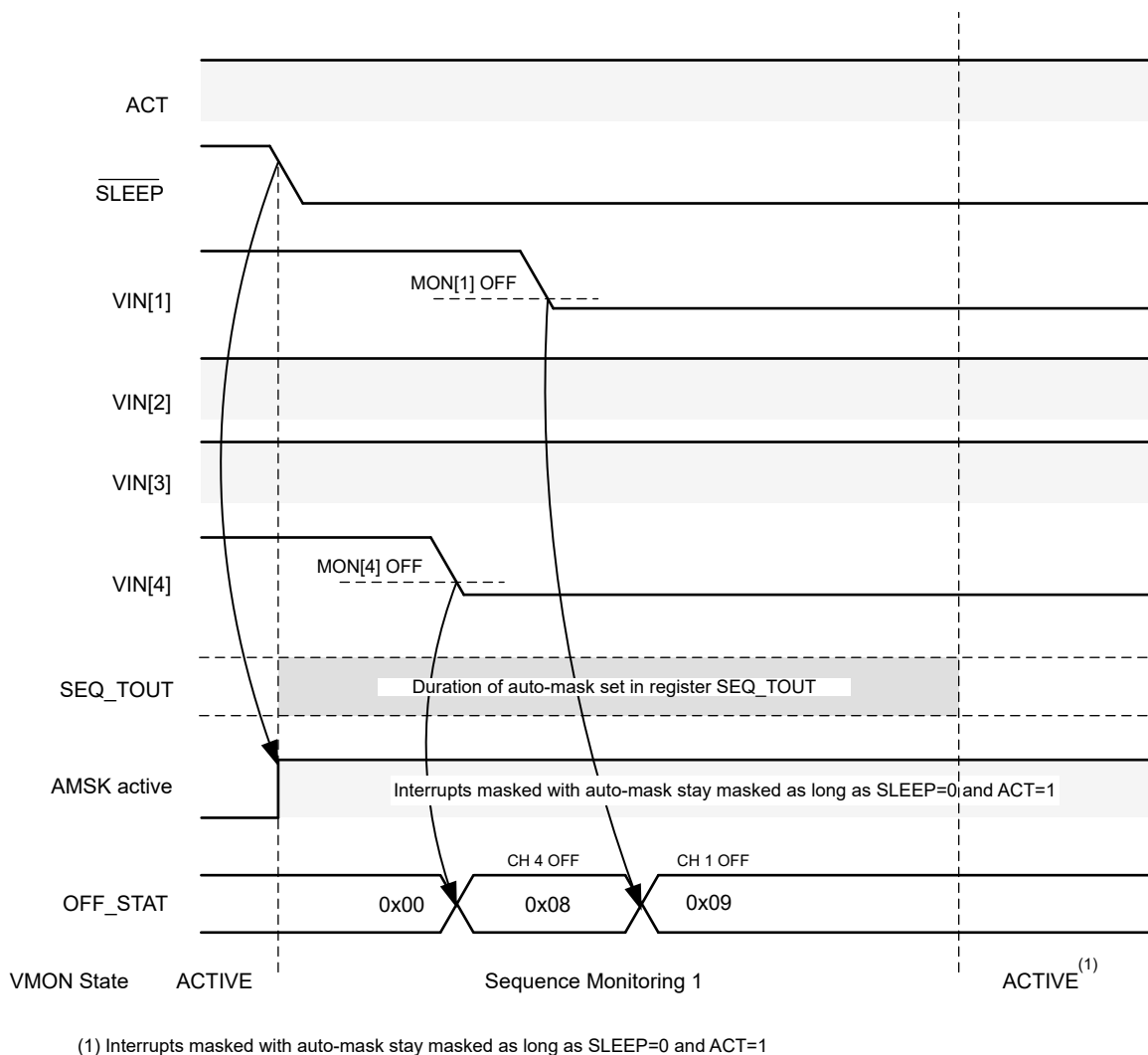
图 7-14. SLEEP 1→0 转换
