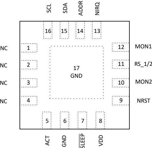
图 5-4. RTE 封装 16 引脚 WQFN TPS388R02 顶视图
