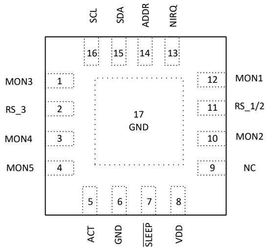
图 5-2. RTE 封装 16 引脚 WQFN TPS388005 顶视图
