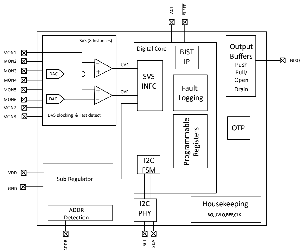
图 7-1. TPS388008 方框图
