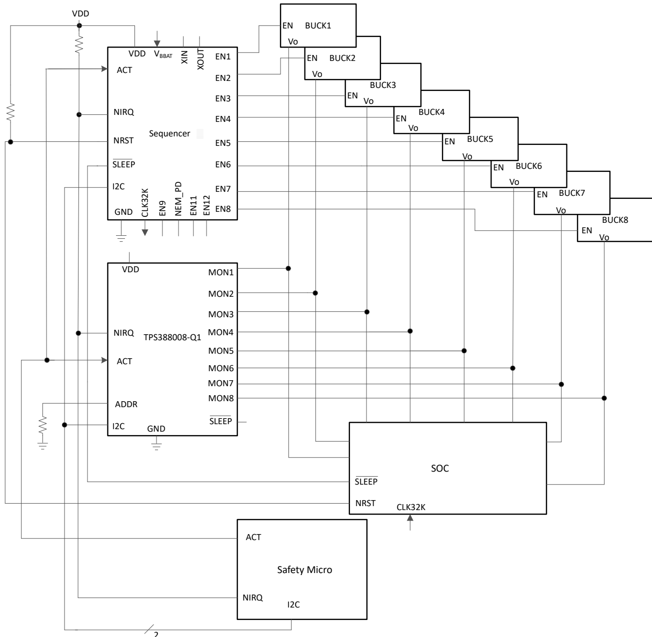
图 8-1. TPS38800 电压监控器设计方框图
