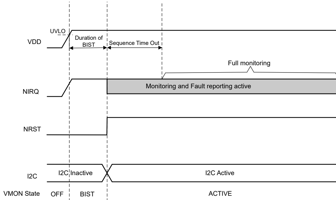
图 7-12. TPS38800/TPS388R0 上电信令和内部状态
