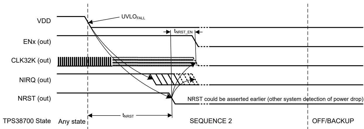
图 7-7. 紧急断电
