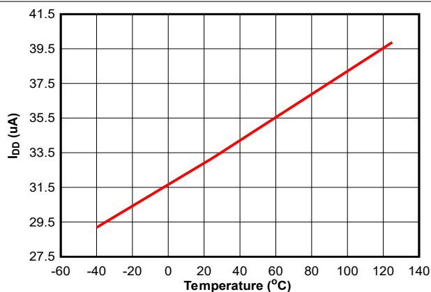
图 6-4. I_{DD} 关断电流与温度间的关系
