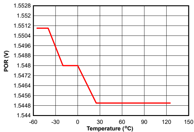
图 6-5. V_{POR} 与温度间的关系
