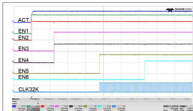
图 8-2. 上电序列
