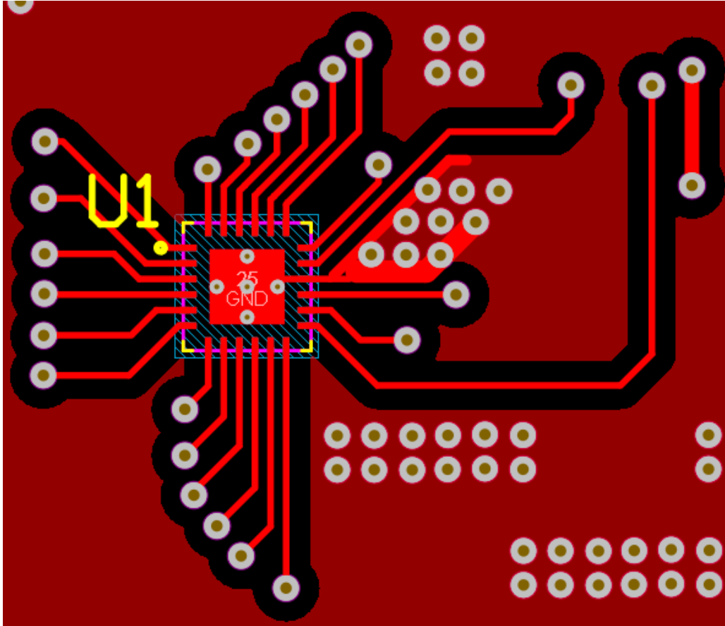
图 8-7. 建议布局
