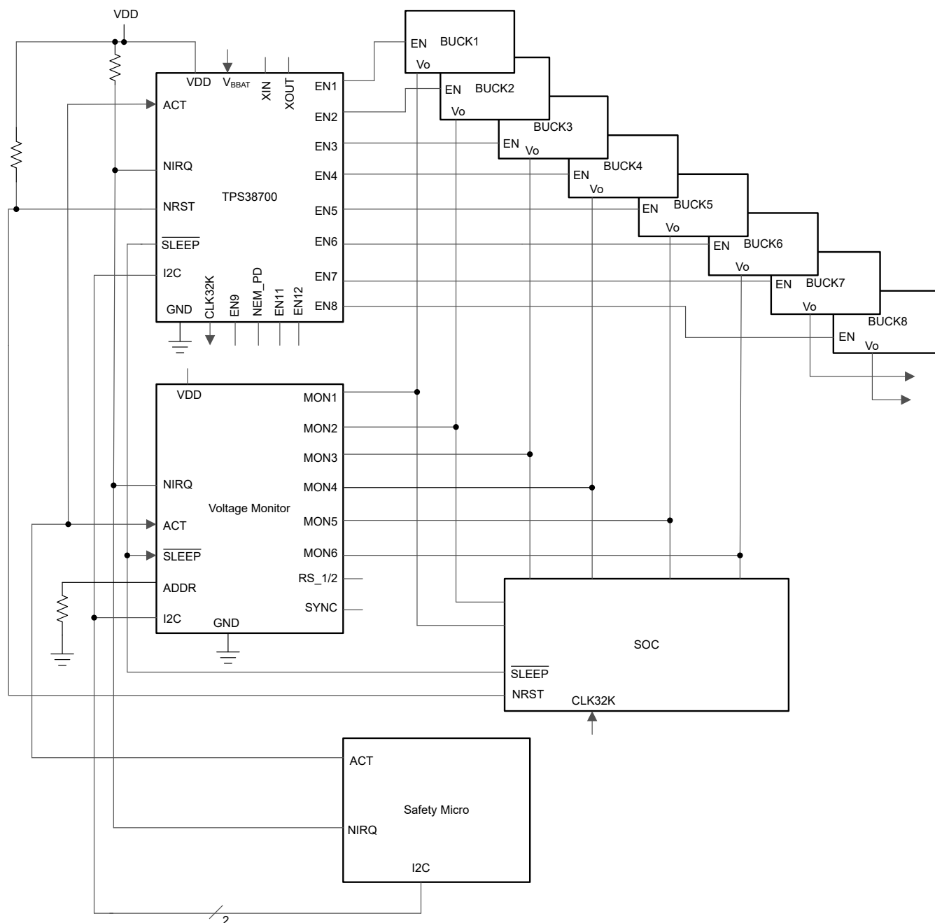
图 8-1. TPS38700-Q1 电压序列发生器设计方框图
