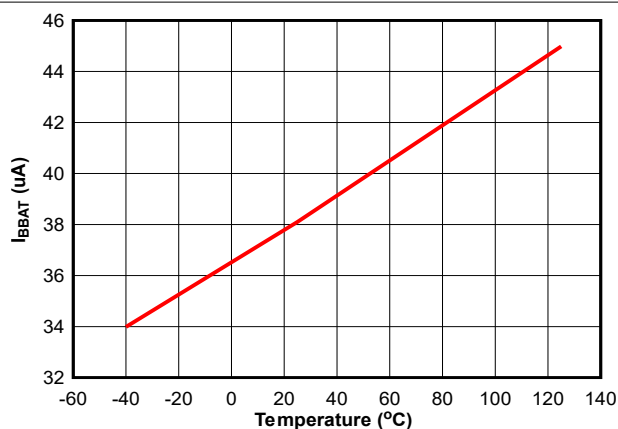
图 6-3. I_{BAT} 与温度间的关系
