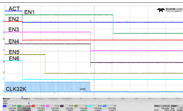
图 8-3. 断电序列
