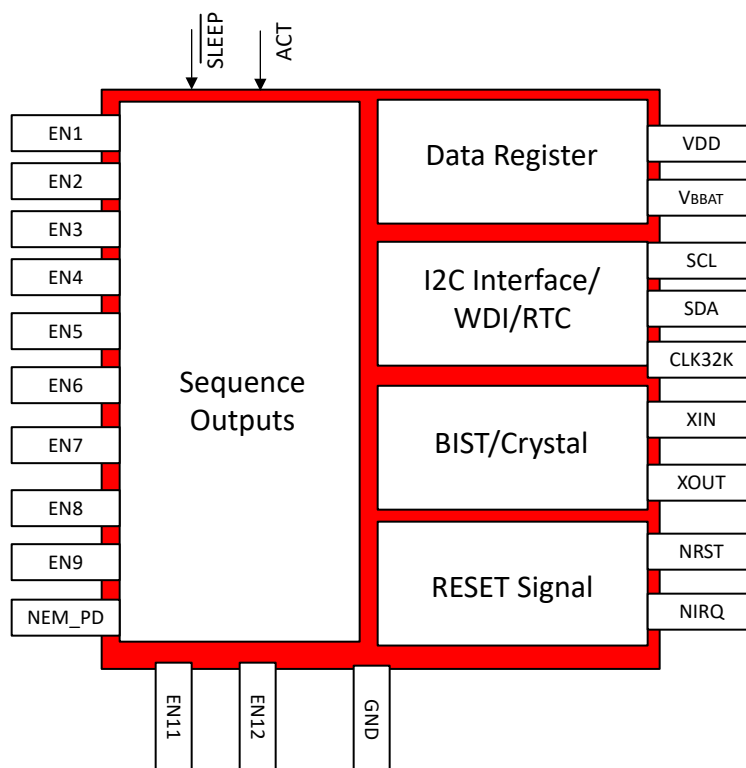
图 7-1. TPS38700 方框图
