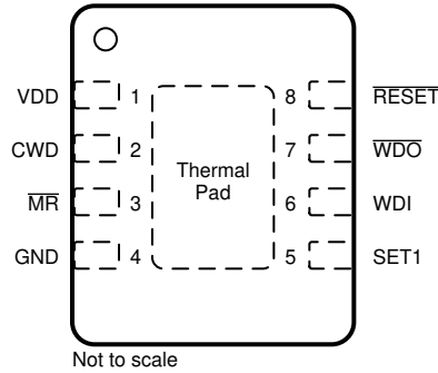
图 4-1. DRB 封装：TPS3851 3mm × 3mm VSON-8 顶视图
