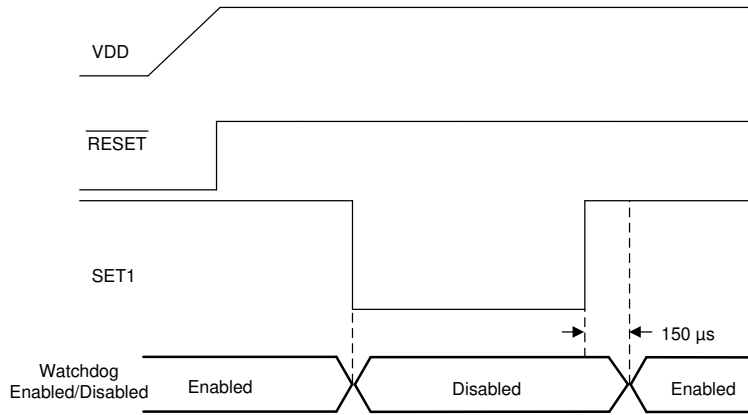
图 6-3. 启用和禁用看门狗
