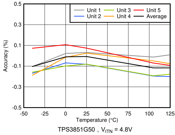
图 5-9. V_{ITN} 精度与温度间的关系
