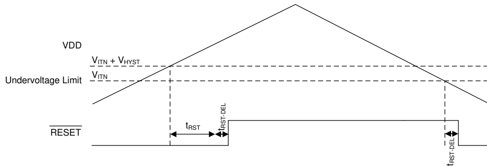
图 6-1. 欠压检测
