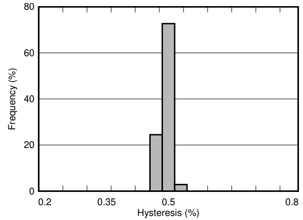
图 5-10. V_{ITN} + V_{HYST} 精度直方图
