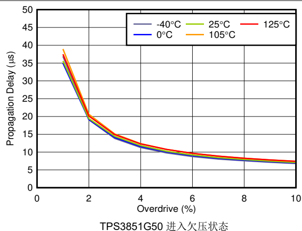
图 5-16. 传播延迟与过驱间的关系
