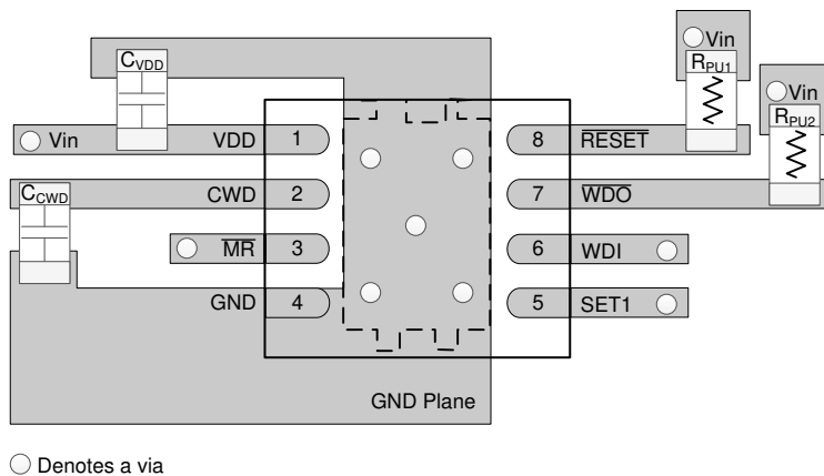
图 7-9. TPS3851 建议布局
