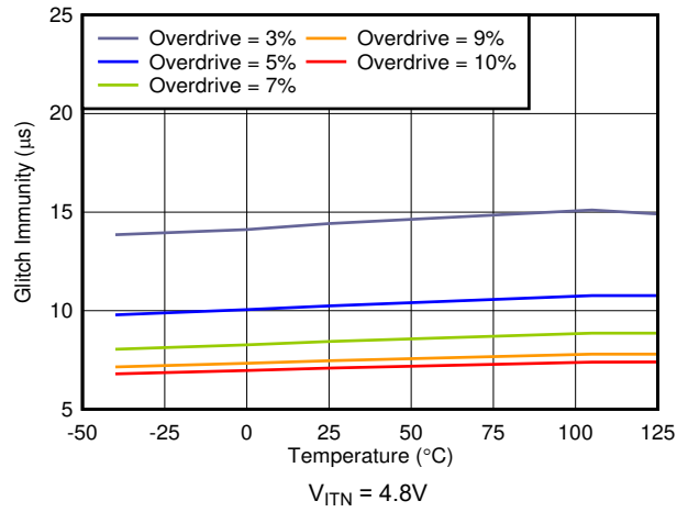
图 5-20. 高到低电平毛刺抑制与温度间的关系
