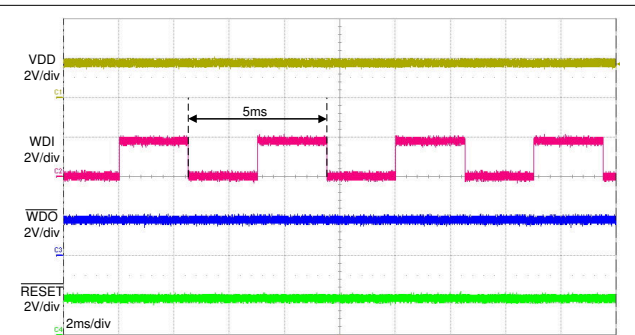
图 7-6. 典型 WDI 信号
