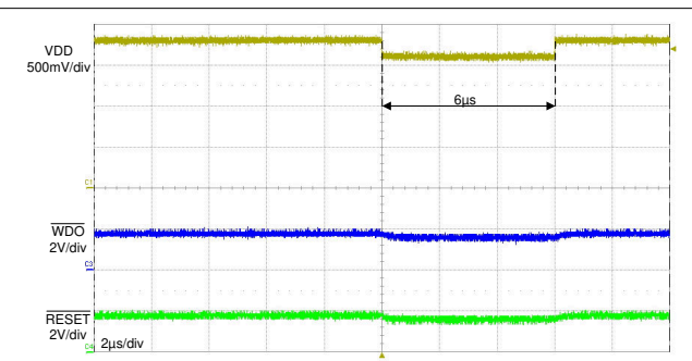
图 7-8. 高到低电平毛刺抑制
