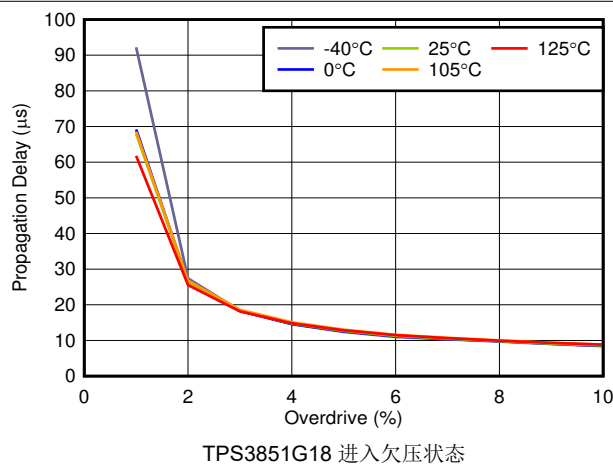
图 5-15. 传播延迟与过驱间的关系
