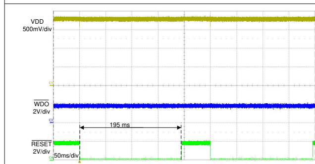
图 7-7. 典型 RESET 延迟
