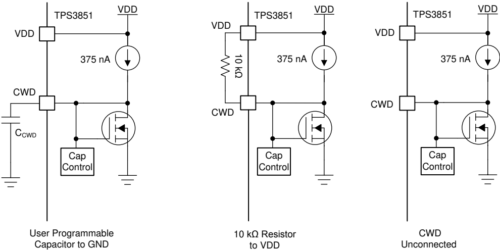
图 7-1. CWD 充电电路
