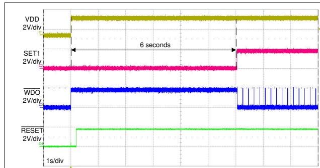
图 7-5. 无 WDI 信号的启动
