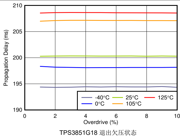
图 5-17. 传播延迟时间 ( t_{\text{RST}} ) 与过驱间的关系
