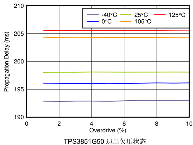
图 5-18. 传播延迟时间 ( t_{\text{RST}} ) 与过驱间的关系
