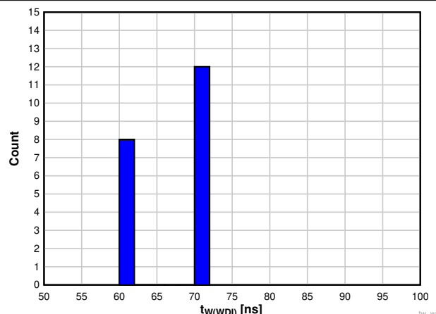
图 6-24. TPS3823A-33 器件在 -40°C 时的 WDI 脉宽直方图 (单位数 = 20)
