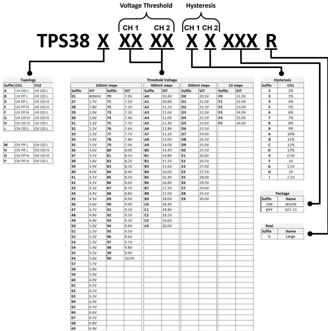
图 5-1. Device Nomenclature
