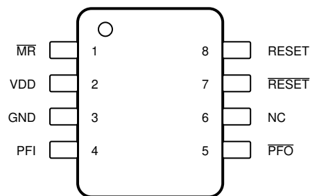
图 6-2. TPS3707-xx D Package 8-Pin SOIC Top View
