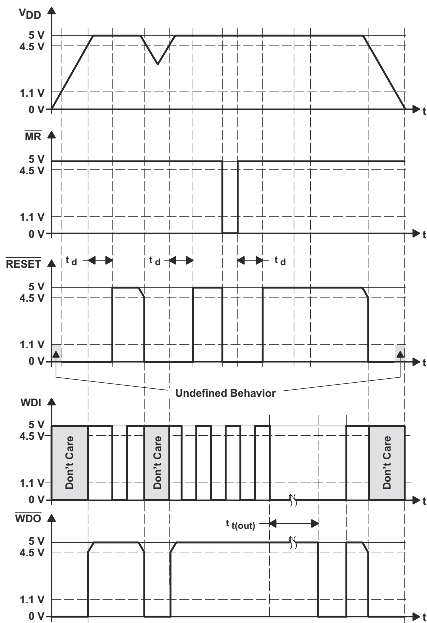
图 7-1. Timing Diagrams
