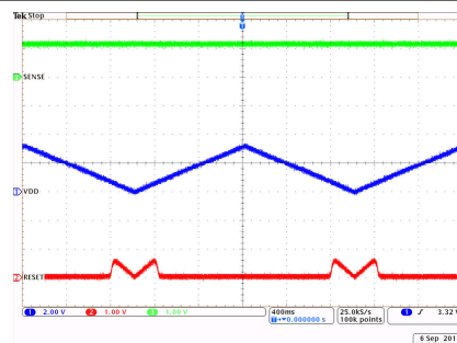
图 9-13. TPS3703-Q1 CT Bias Unlatch Function
