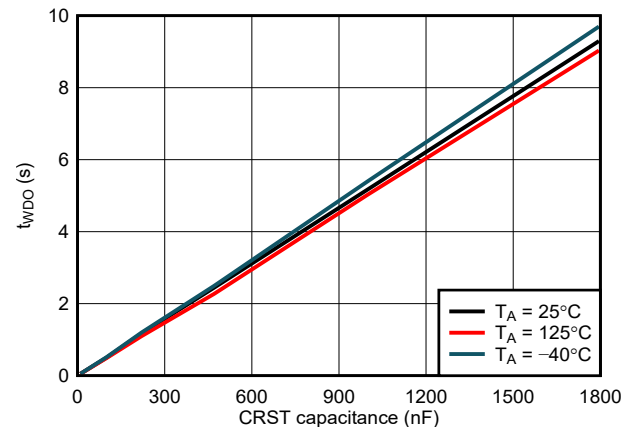
图 7-5. t_{WDO} 与电容间的关系
