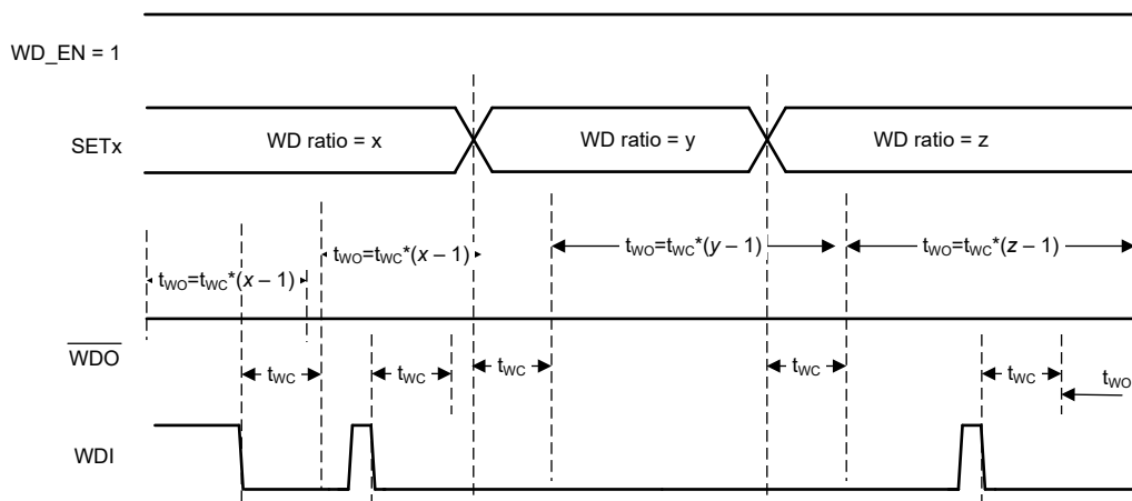
图 8-7. 具有 SETx 引脚状态的看门狗行为
