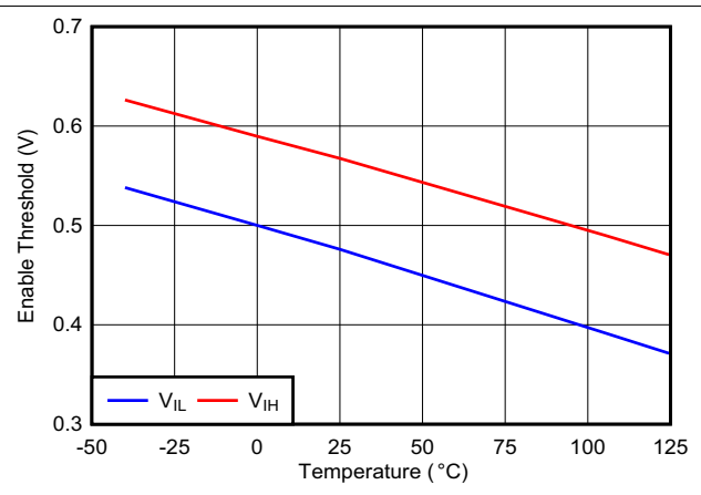
图 6-4. EN Threshold vs Temperature V_{DD} = 1.8\text{ V}
