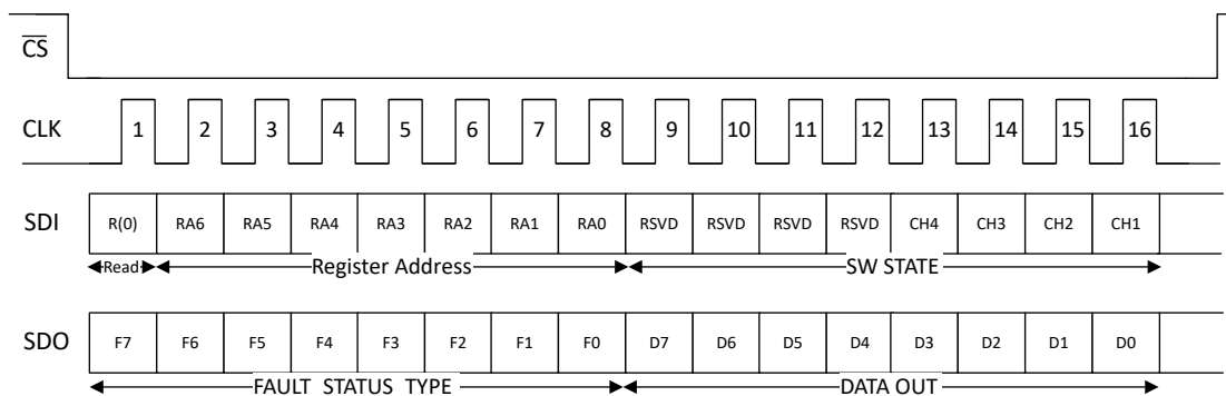
图 8-11. 16-bit Read, DSPI=1, D24BIT=0, CRC_EN=0
