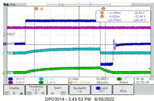
图 8-26. TPS274C65 Inductive Discharge (100mH + 48 \Omega )
