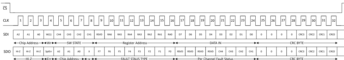
图 8-10. 32-bit Write, DSPI=0, D24BIT=x, CRC_EN=1
