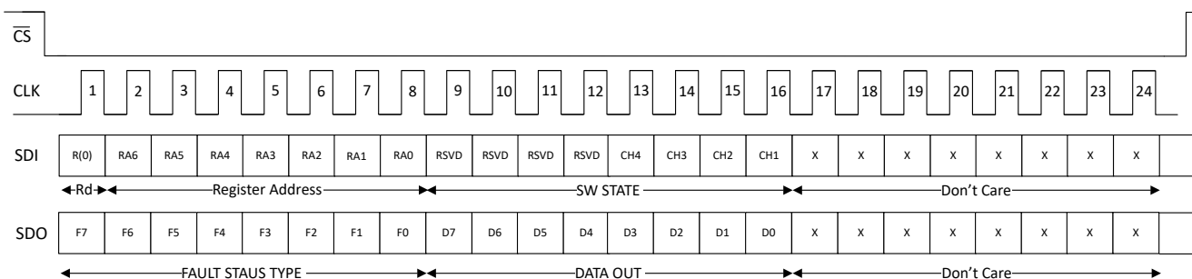
图 8-13. 24-bit Read, DSPI=1, D24BIT=1, CRC_EN=0
