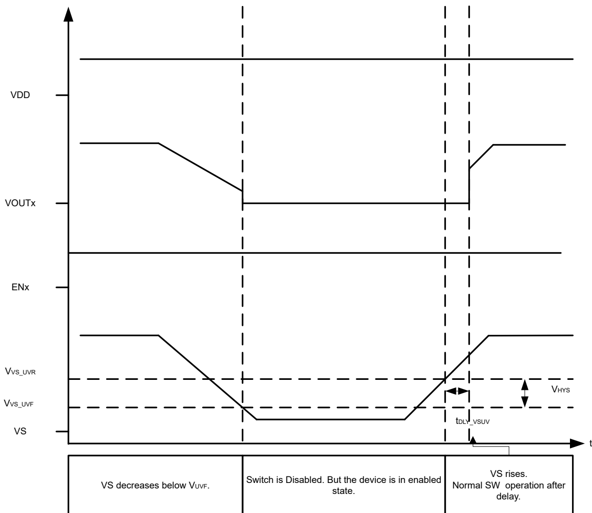
图 8-28. VS UVP
