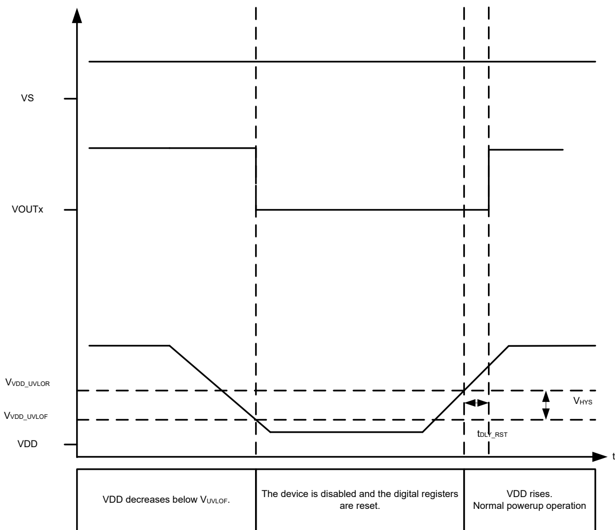
图 8-29. VDD UVLO
