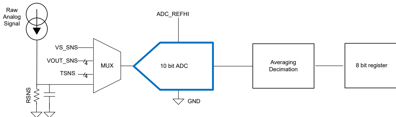
图 8-39. ADC Block Diagram
