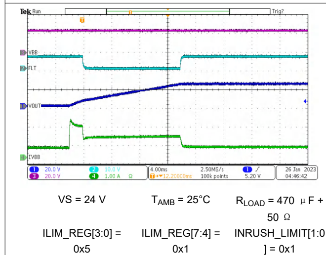
图 6-3. Charging a 470-μF Capacitor
