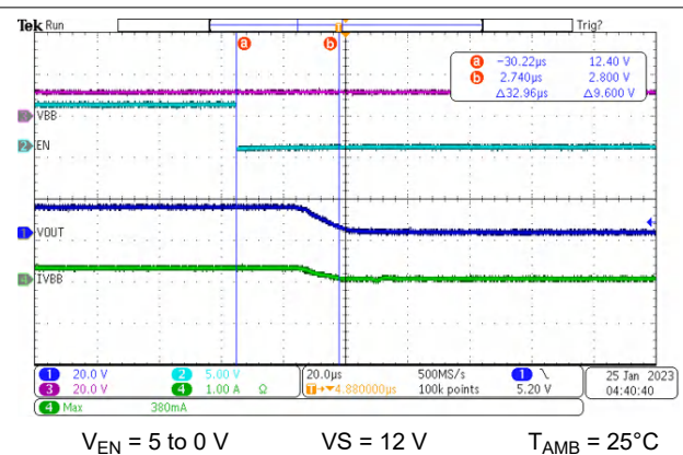
图 6-2. Turn-off Time (tOFF)
