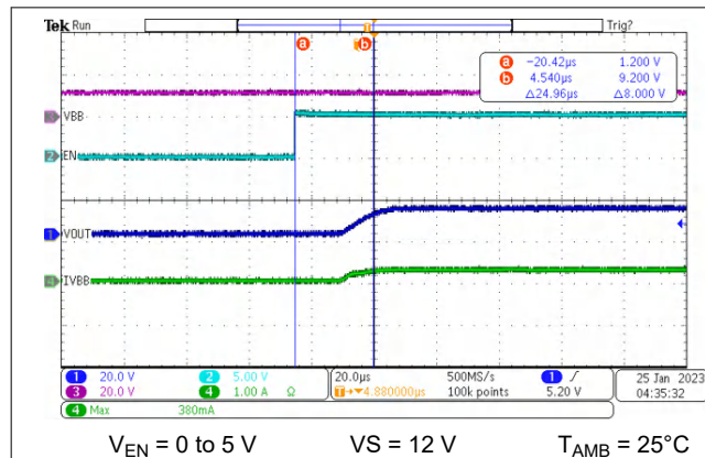
图 6-1. Turn-on Time (tON)
