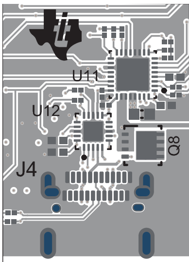
图 8-12. PCB 布局 — 顶部复合图
