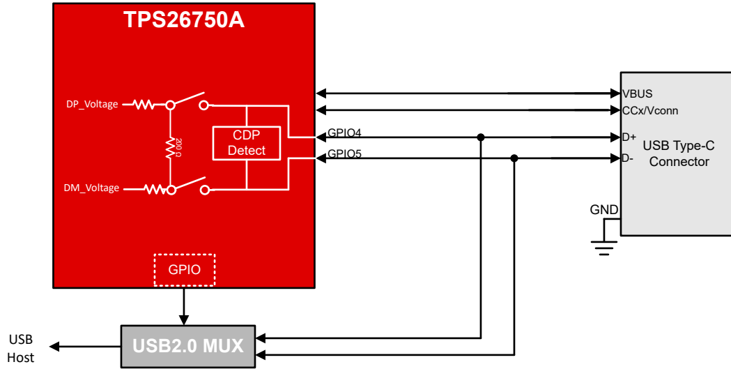
图 8-6. BC1.2 应用方框图
