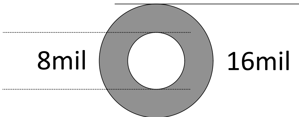
图 8-10. 建议的最小过孔尺寸
