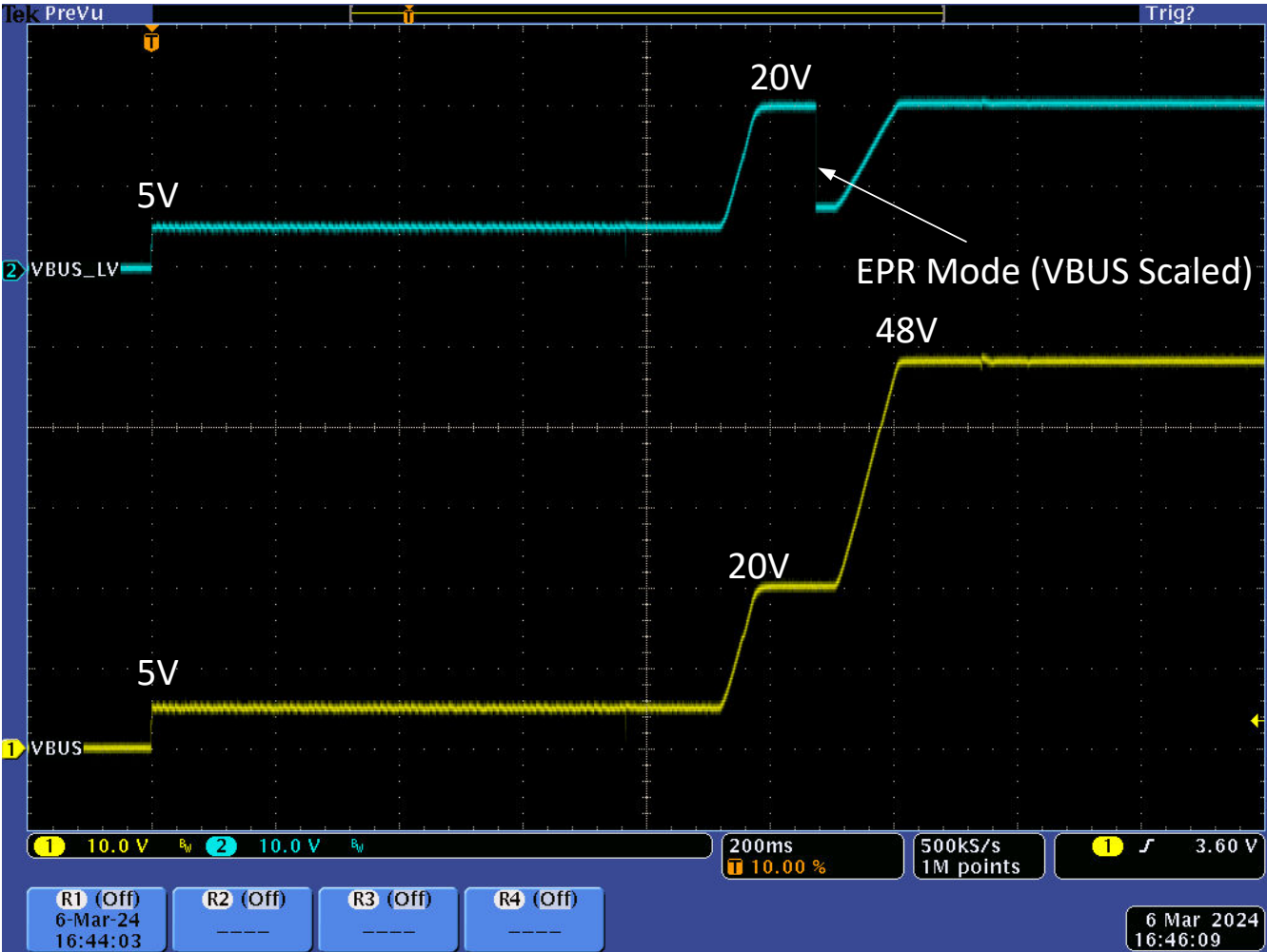
图 8-9. 48V EPR 合约协商 VBUS 和 VBUS LV
