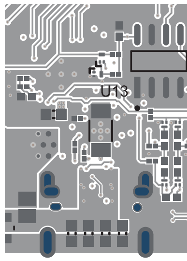
图 8-13. PCB 布局 — 底部复合图
