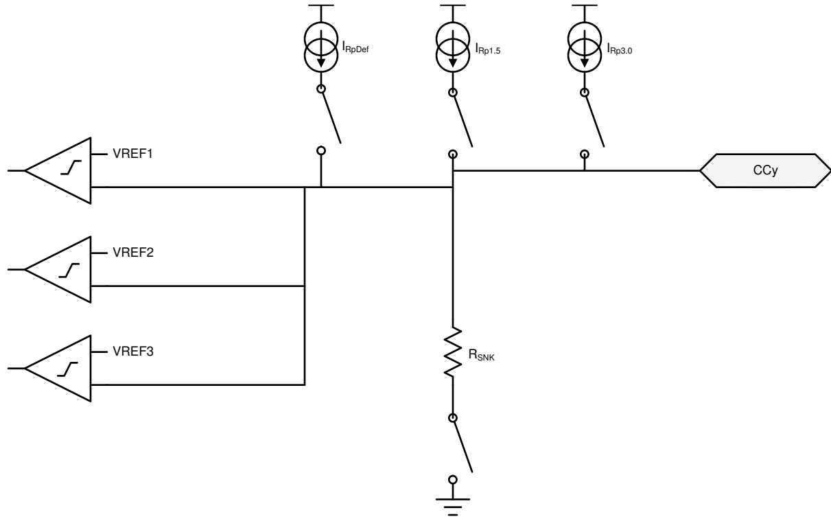
图 7-12. 插头和方向检测块
