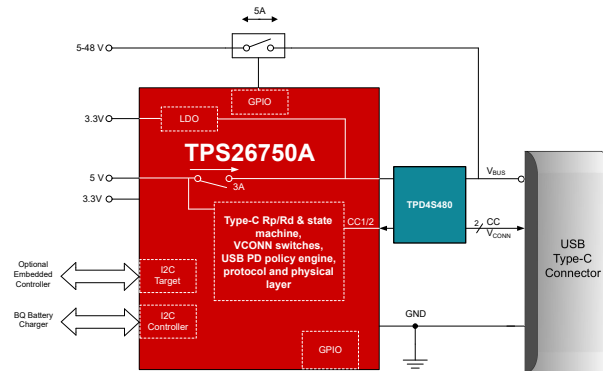
TPS26750A 原理图
