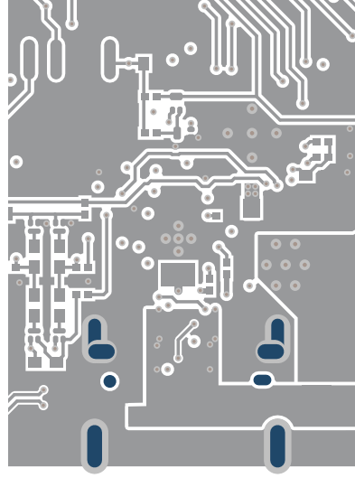
图 8-19. PCB 布局 — 底层 6
