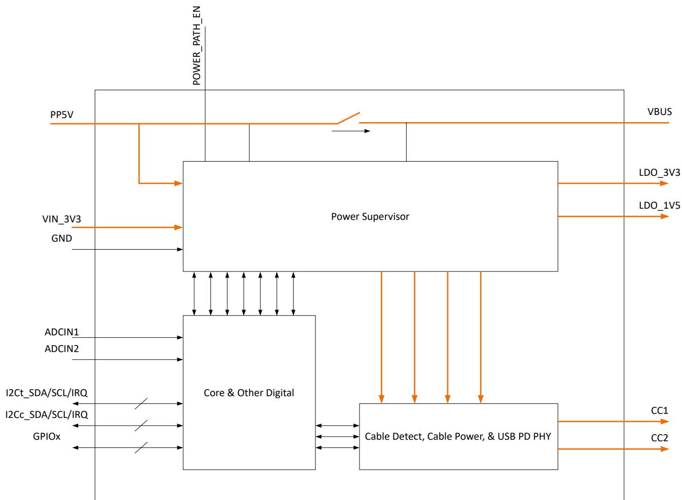
图 7-1. TPS26750A
