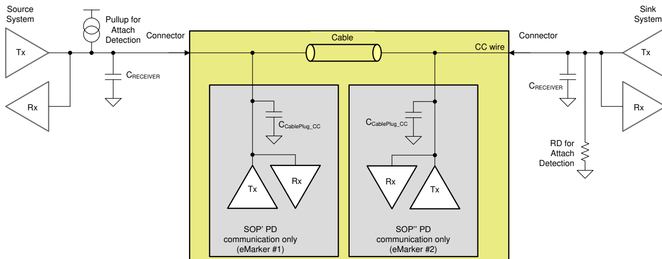
图 7-9. USB-PD 多点配置示例
