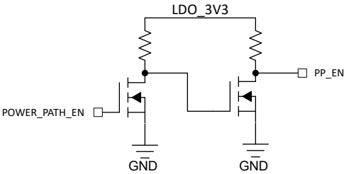
图 8-3. POWER_PATH_EN 缓冲器
