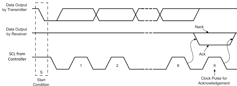
图 7-20. I²C 确认
