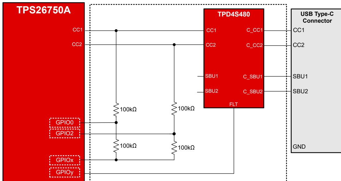
图 8-4. TPS26750A 液体检测方框图 — CC1 和 CC2 监测引脚
