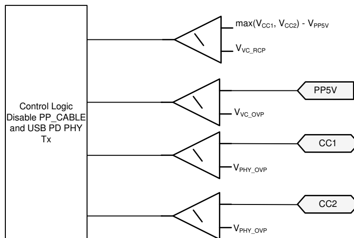
图 7-13. CC1 和 CC2 的过压和反向电流保护
