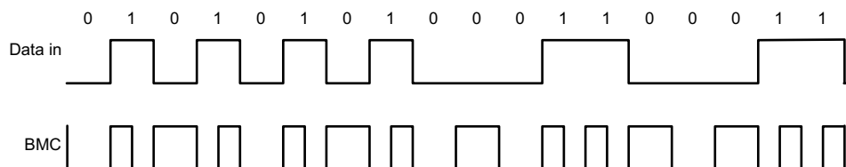
图 7-5. 双相标记编码示例
