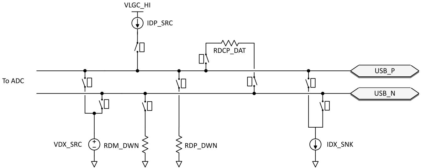
图 7-16. BC1.2 硬件元件
