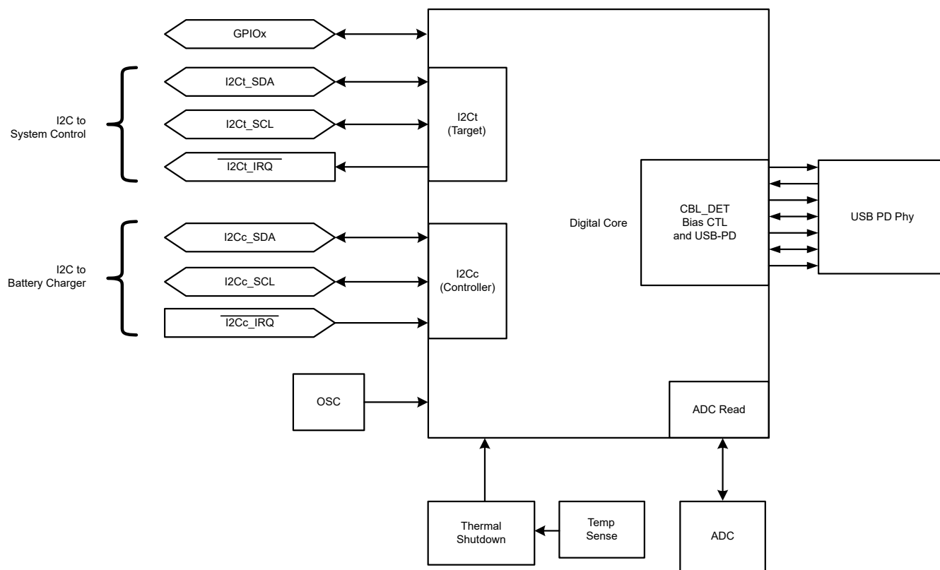
图 7-24. 数字内核方框图
