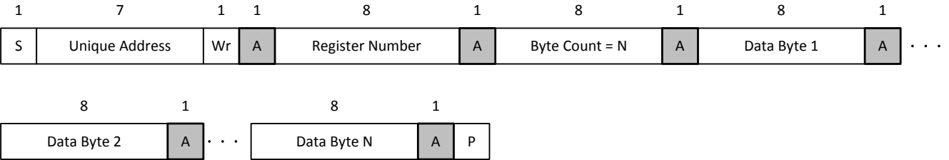
图 7-21. I 2 C 唯一地址写入寄存器协议
