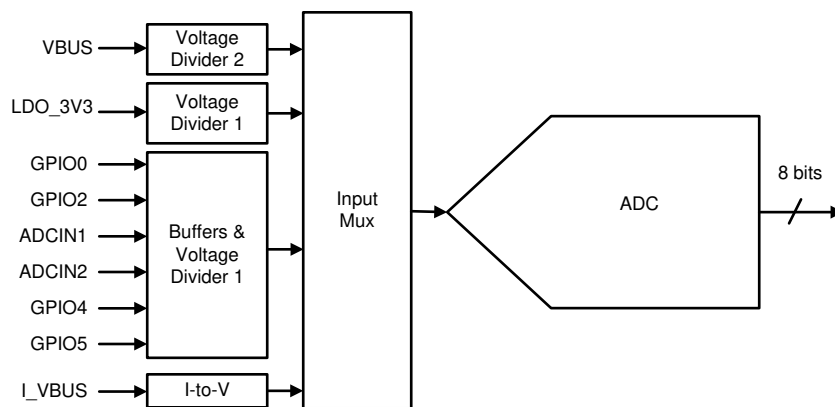
图 7-15. SAR ADC
