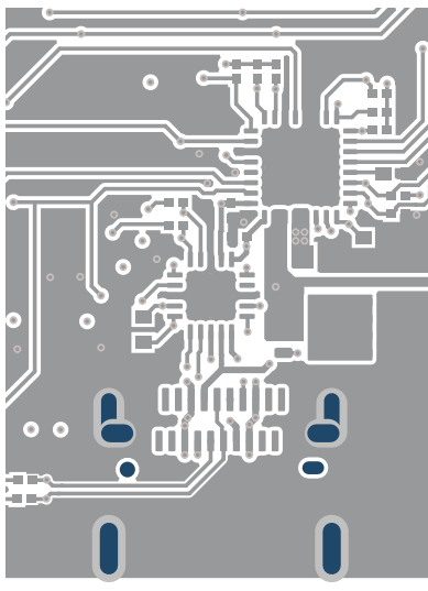
图 8-14. PCB 布局 — 顶层 1
