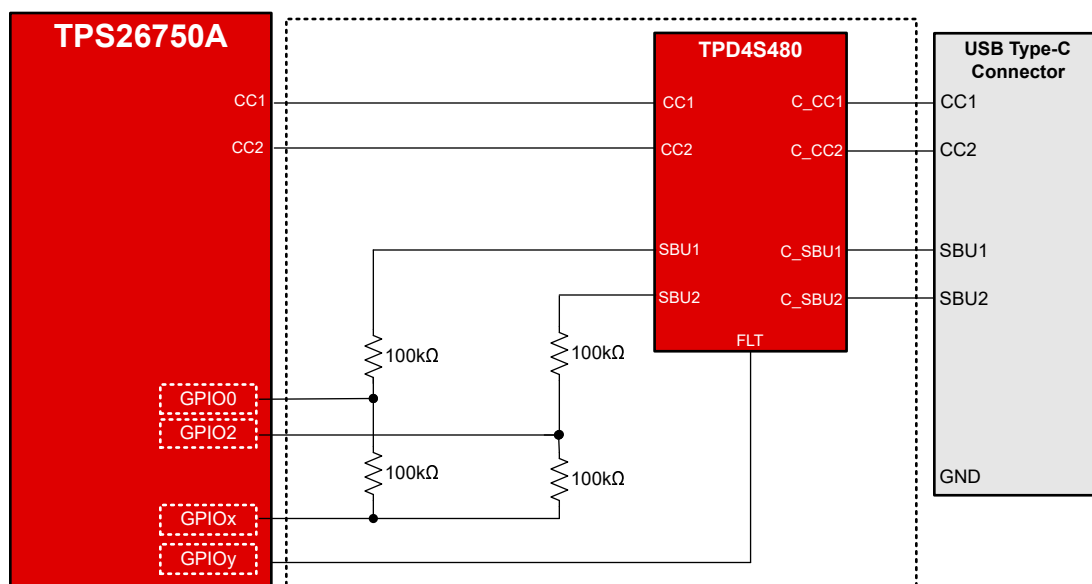
图 8-5. TPS26750A 液体检测方框图 — SBU1 和 SBU2 监测引脚
