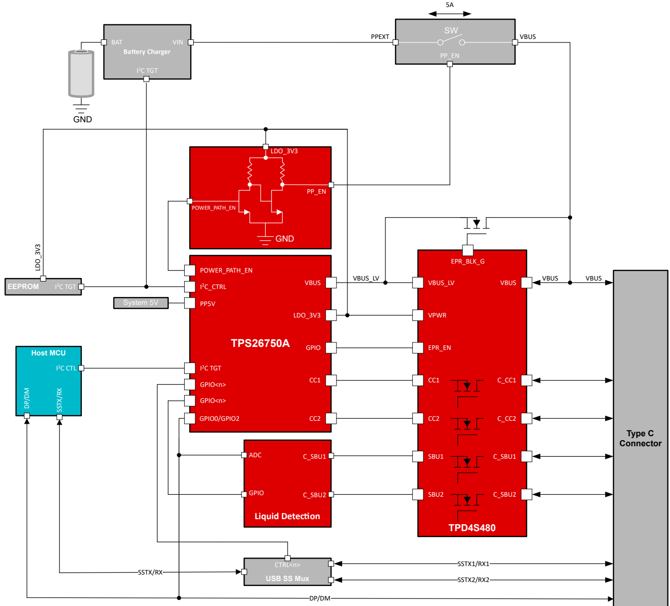
图 8-1. TPS26750A 电池充电器和完整系统方框图
