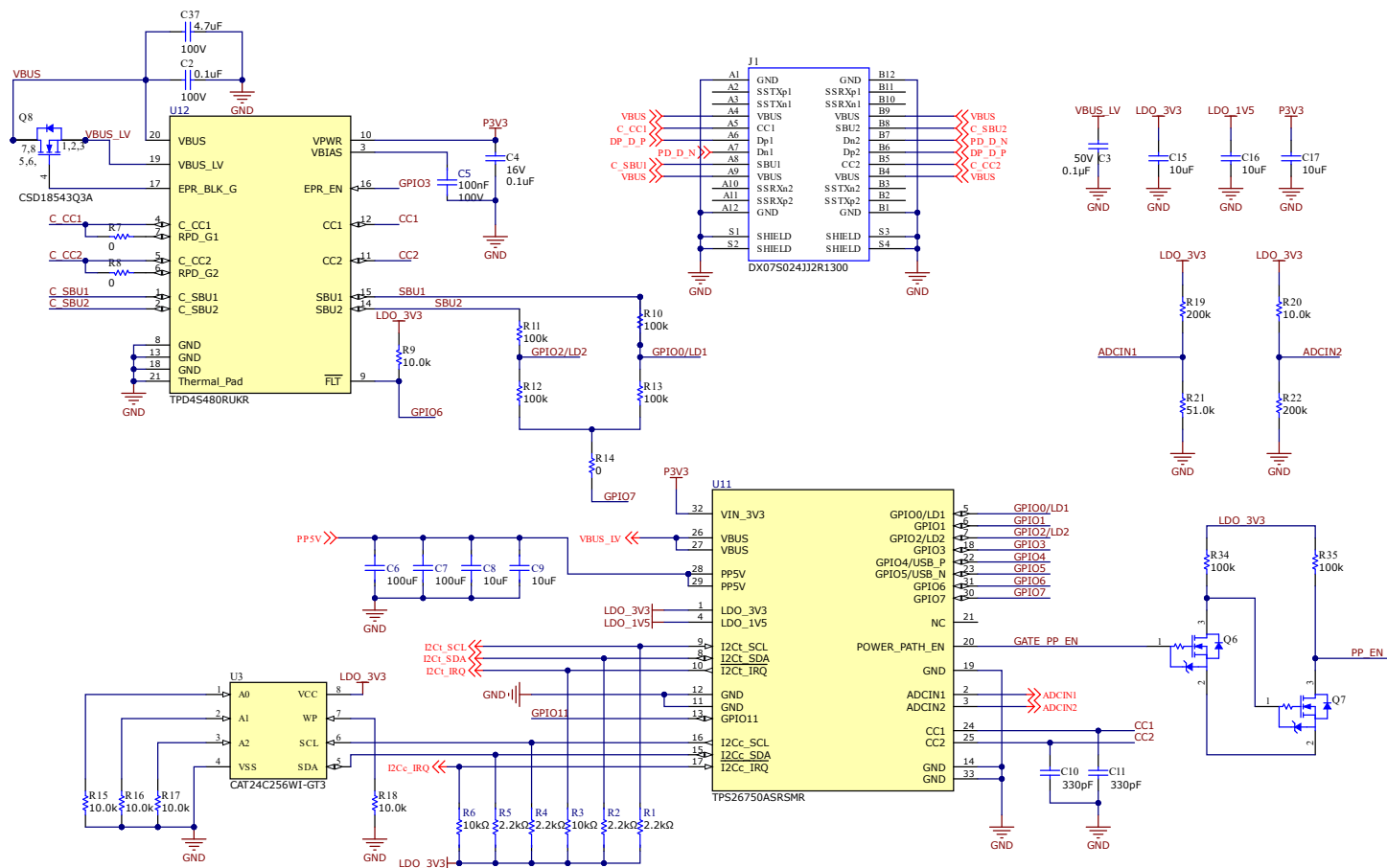
图 8-11. 示例原理图
