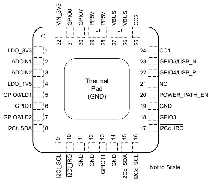
图 4-1. TPS26750A QFN 封装，32 引脚（顶视图）
