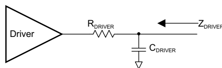
图 7-8. ZDRIVER 电路
