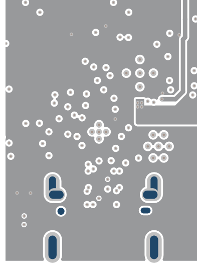
图 8-17. PCB 布局 — 信号层 4
