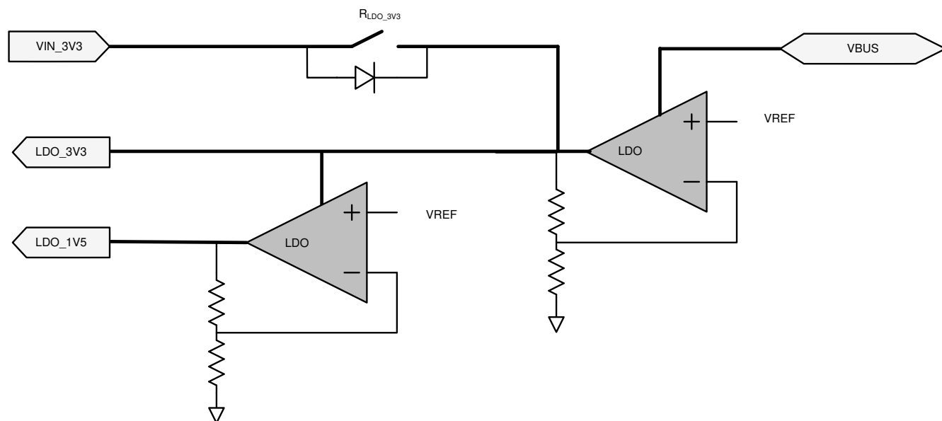
图 7-10. 电源
