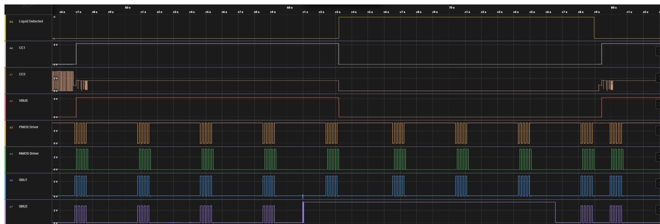
图 8-8. 液体检测行为 - 腐蚀缓解
