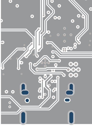
图 8-16. PCB 布局 — 信号层 3
