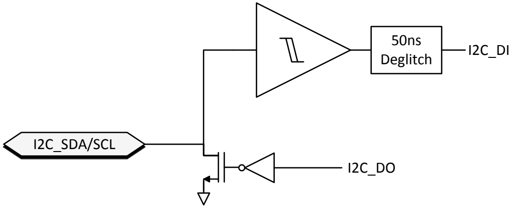
图 7-17. I 2 C 缓冲器
