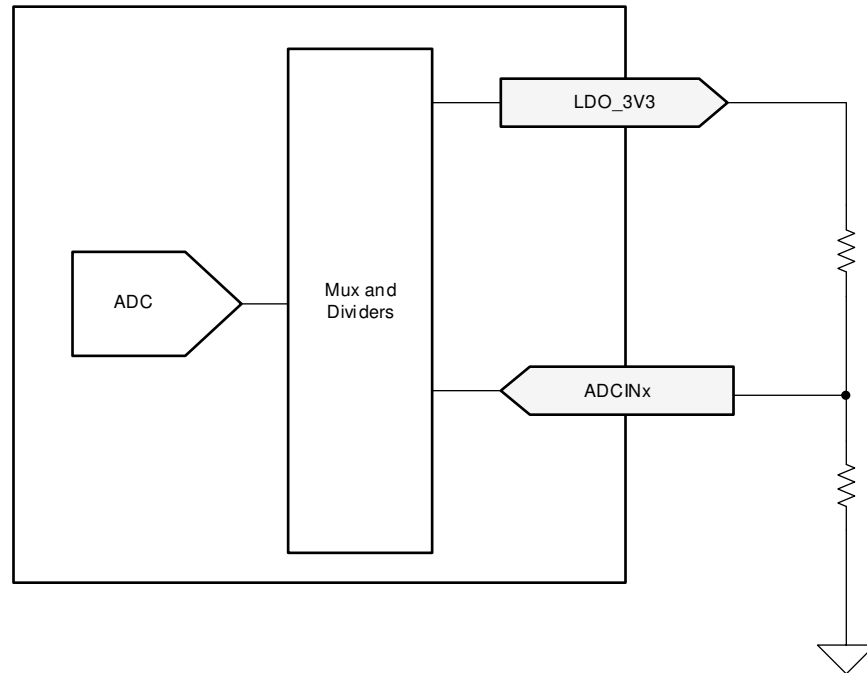
图 7-14. ADCINx 电阻分压器
