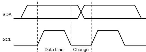
图 7-19. I²C 位传输
