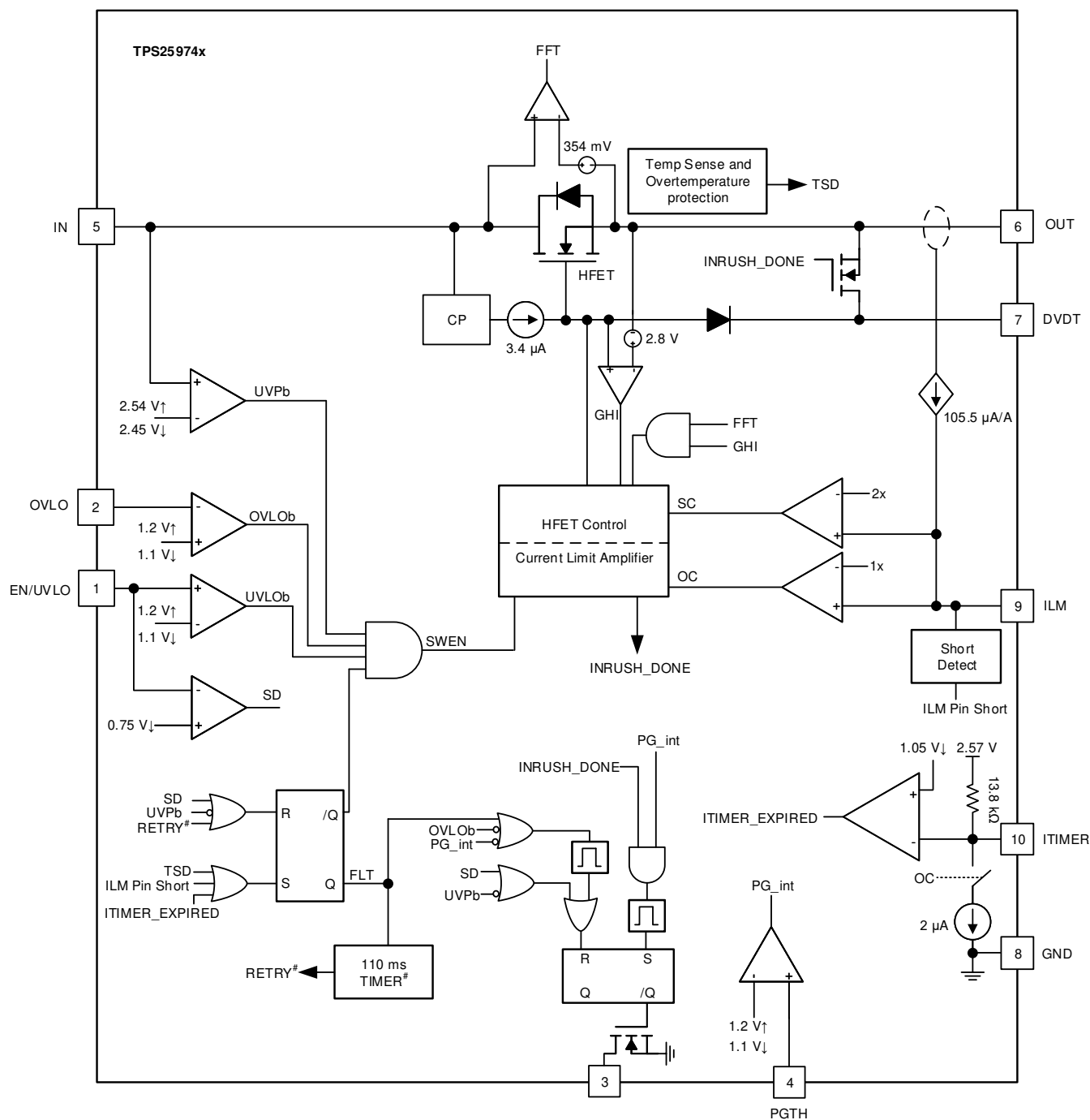
图 7-3. TPS25974x Block Diagram
