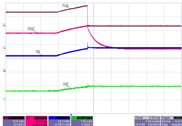
图 10-9. Overvoltage Shutdown
