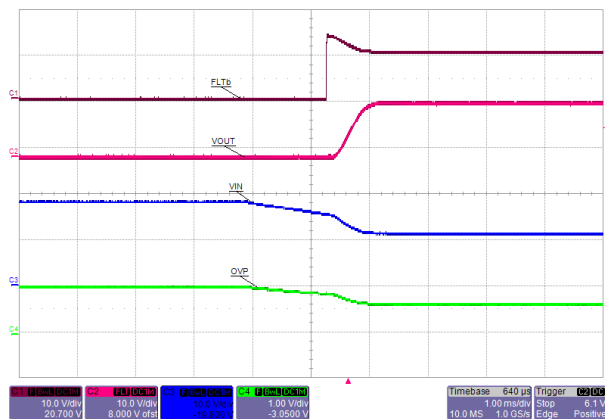
图 10-10. Overvoltage Recovery
