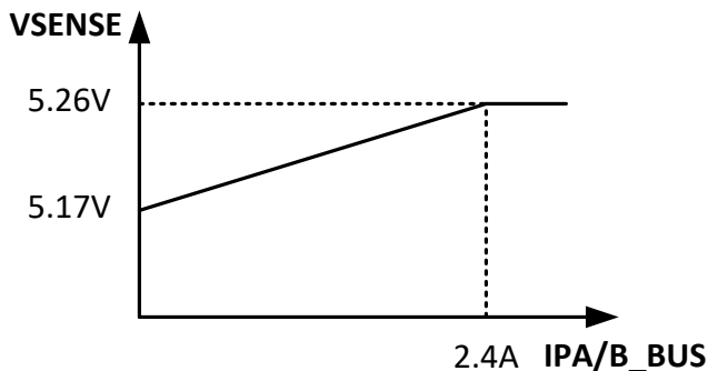
图 10-9. Dual Ports Cable Compensation
