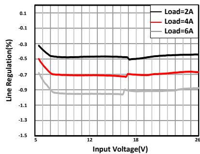
图 11-6. Line Regulation
