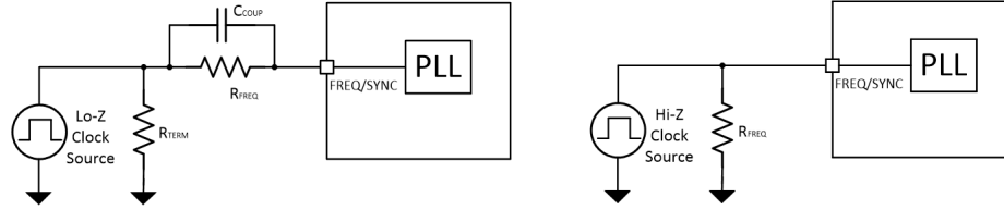
图 10-4. Synchronize to External Clock
