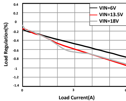
图 11-6. Load Regulation
