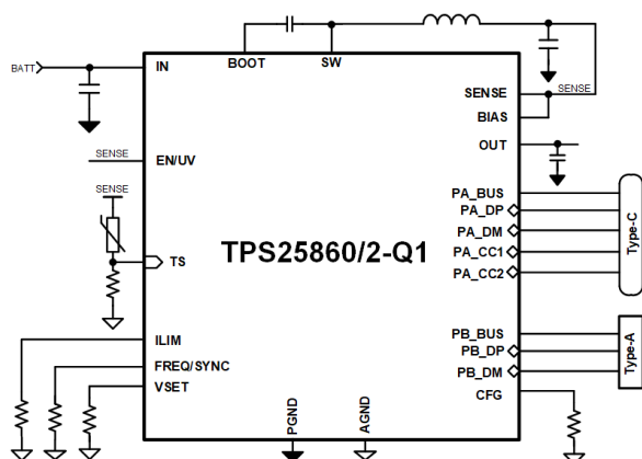
简化版原理图：TPS2586x-Q1
