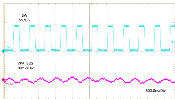
图 11-15. 100-mA Output Ripple
