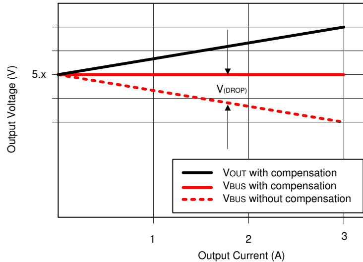
图 10-14. Voltage Drop
