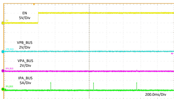
图 11-21. Rd Assert
