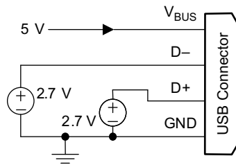
图 10-23. Divider 3 Mode
