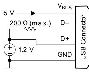
图 10-24. 1.2-V Mode
