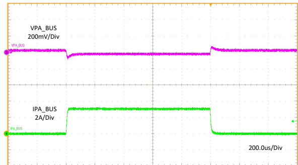
图 11-6. Load Regulation
