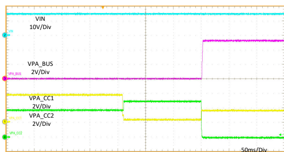
图 11-21. Rd Assert
