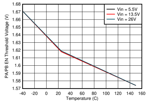
图 8-4. Precision USB PA/PB Enable Threshold
