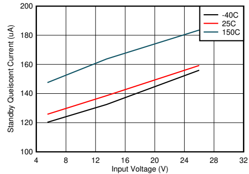
图 8-2. Standby Quiescent Current
