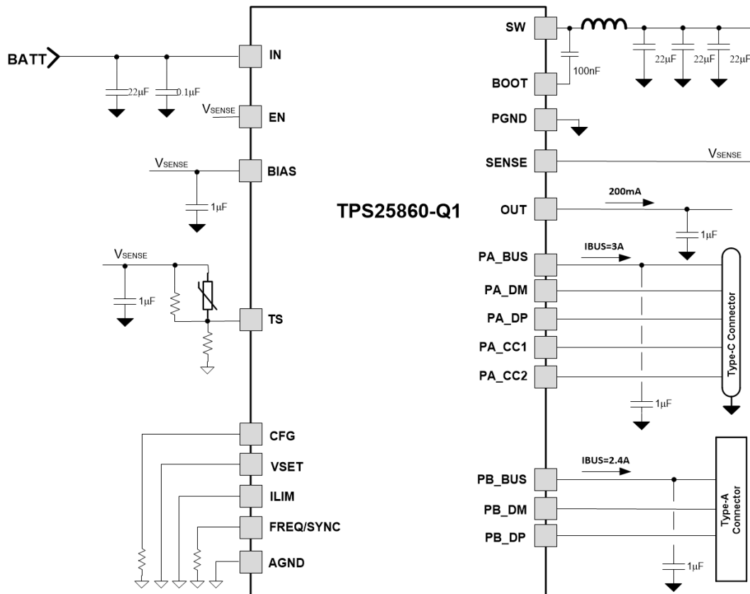
图 11-1. TPS25860-Q1 Typical Application Circuit for 2.1-MHz f_{sw}
