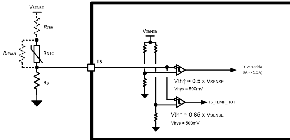
图 10-16. TS Input
