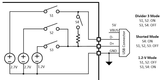
图 10-25. DCP Auto Mode
