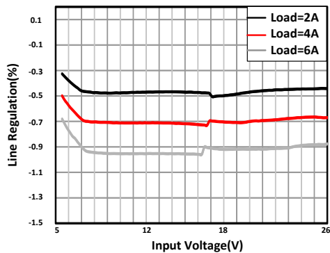
图 11-7. Line Regulation
