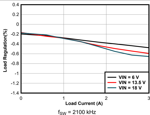
图 11-6. Load Regulation
