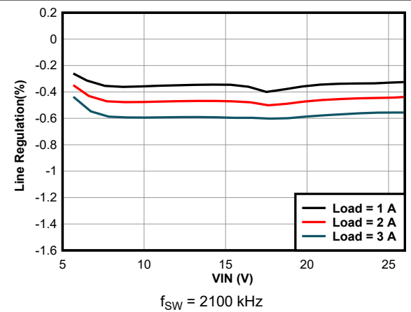
图 11-7. Line Regulation
