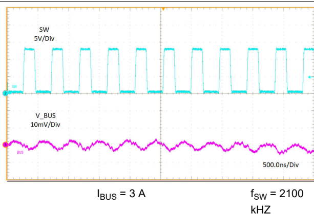
图 11-13. 6-A Output Ripple
