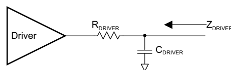
图 8-25. ZDRIVER 电路
