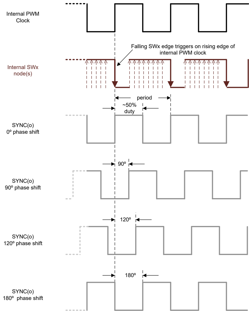
图 8-15. SYNC(o) 相移
