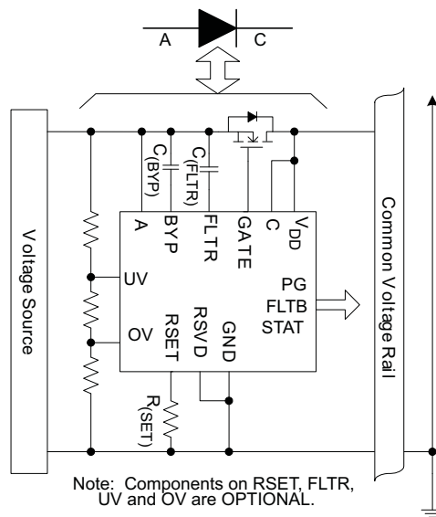
典型应用图
