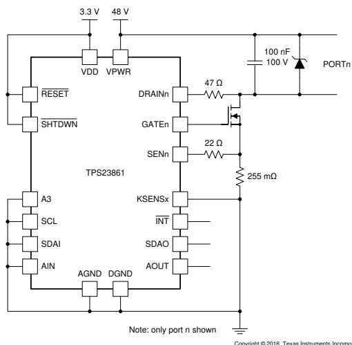
简化原理图
