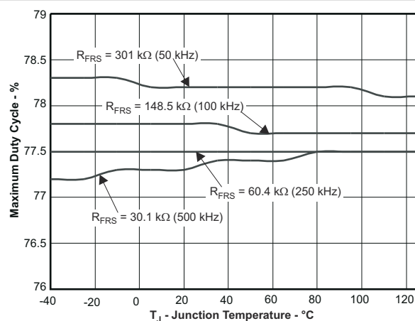
图 7-9. Maximum Duty Cycle vs Temperature
