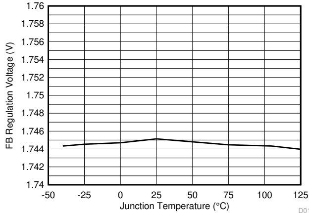
图 7-13. 反馈调节电压与温度间的关系
