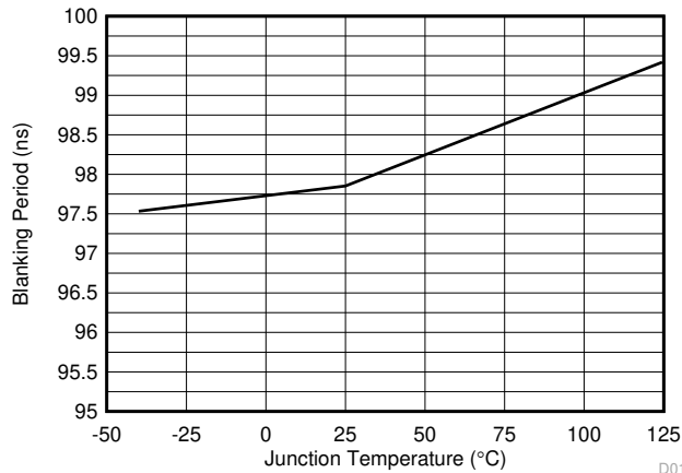
图 7-15. 消隐周期与温度间的关系
