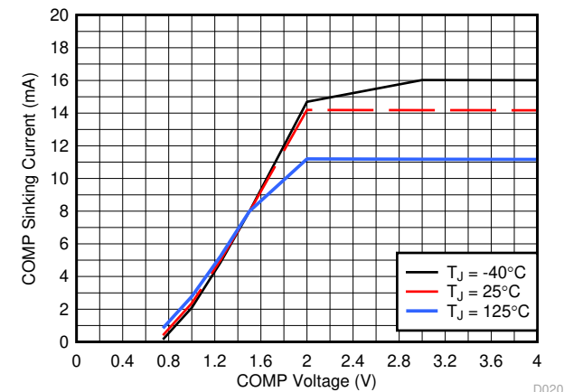
图 7-17. 误差放大器灌电流
