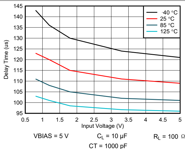
图 6-5. Delay Time vs Input Voltage
