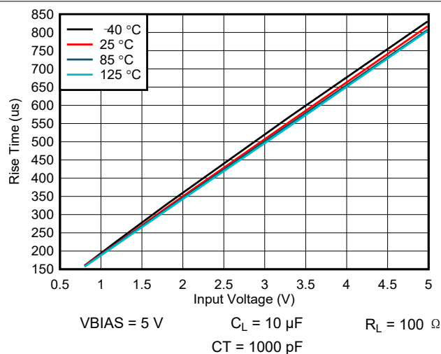
图 6-6. Rise Time vs Input Voltage
