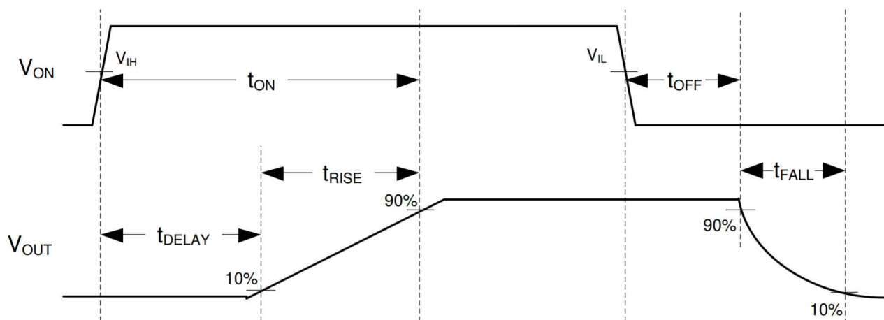
图 7-1. TPS22997 Timing Diagram
