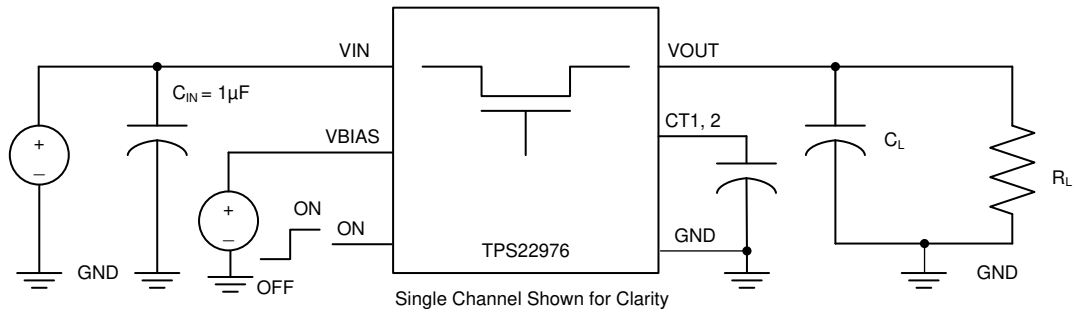
图 7-1. Test Circuit
