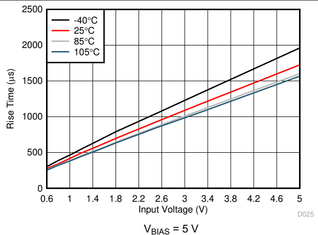
图 6-30. Rise Time vs Input Voltage
