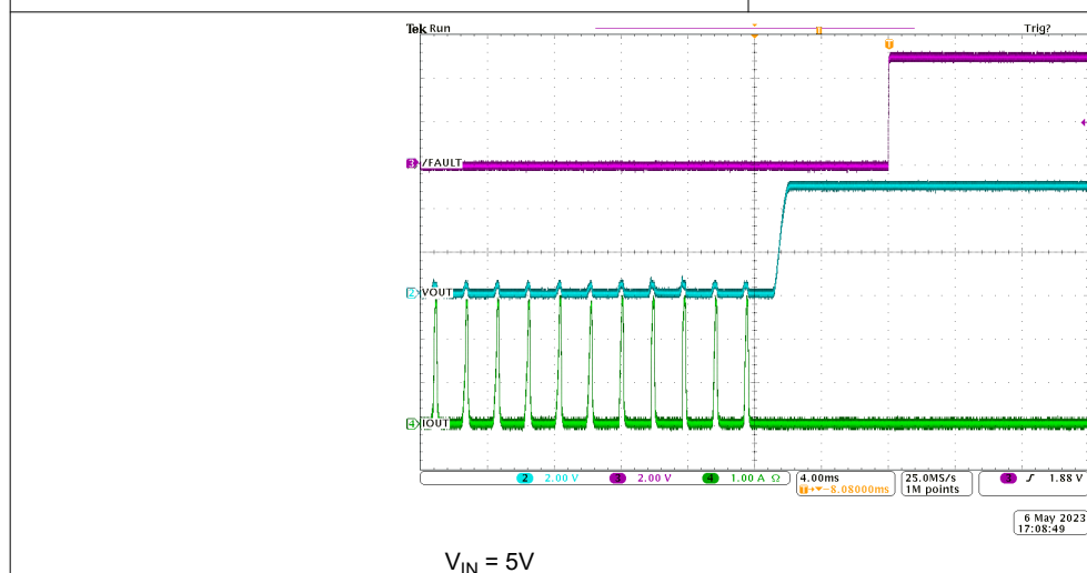
图 8-8. TPS2001E 输出至空载短路
