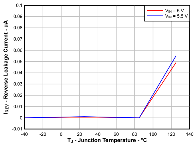
图 6-11. 反向漏电流 ( I_{REV} ) 与温度间的关系
