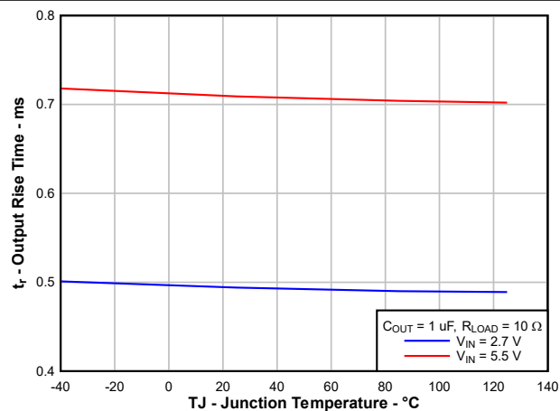
图 6-15. 输出上升时间 ( T_R ) 与温度间的关系
