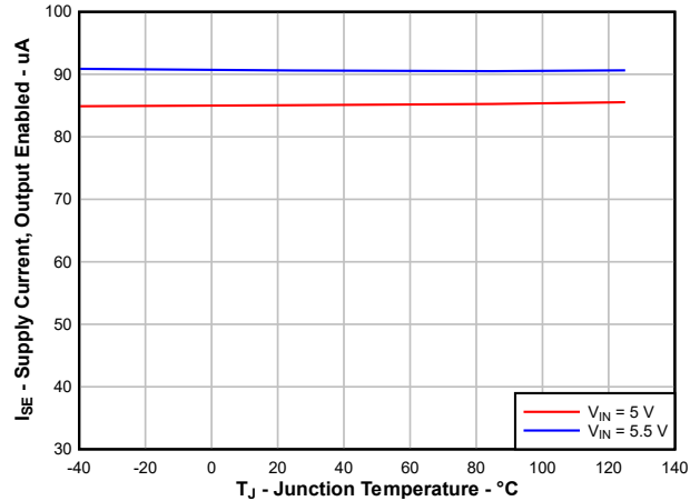
图 6-13. 启用电源电流 ( I_{SE} ) 与温度间的关系
