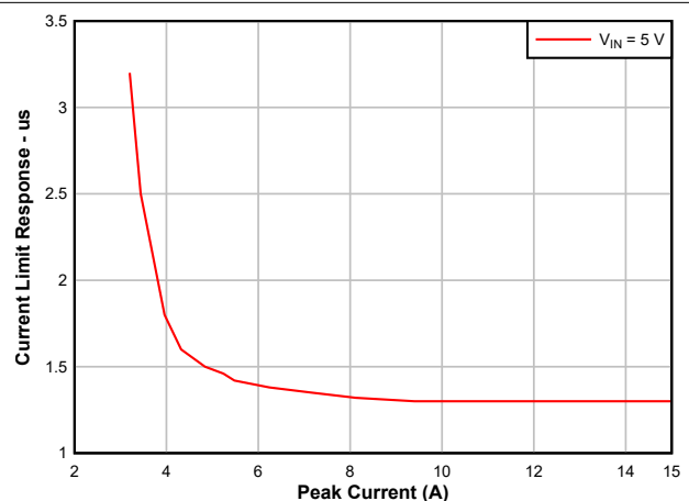
图 6-18. 电流限制响应 ( t_{IOS} ) 与峰值电流间的关系
