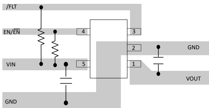
图 8-9. 建议布局 - DBV
