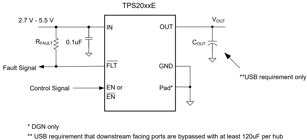
图 8-1. 典型应用原理图
