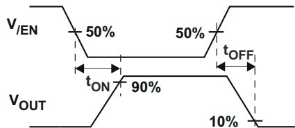
图 6-4. 使能时序，低电平有效使能
