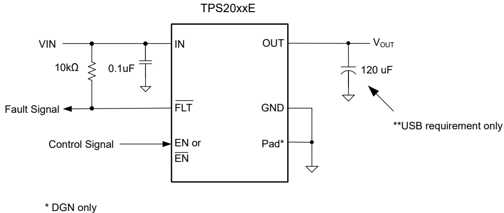
典型应用图
