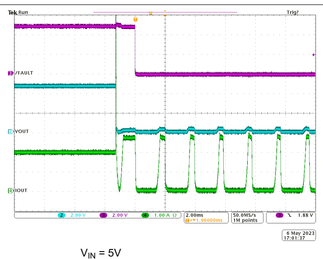
图 8-5. TPS2001E 满载至输出短路
