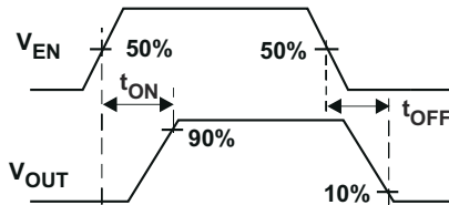
图 6-3. 使能时序，高电平有效使能
