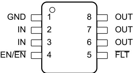
图 5-2. DGK 封装 8 引脚 VSSOP 顶视图
