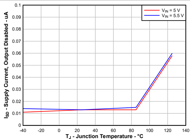
图 6-12. 禁用电源电流 ( I_{SD} ) 与温度间的关系
