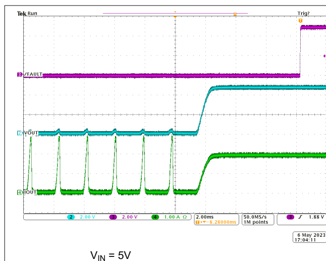
图 8-6. TPS2001E 输出对满载短路
