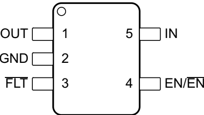
图 5-3. DBV 封装 5 引脚 SOT-23 顶视图
