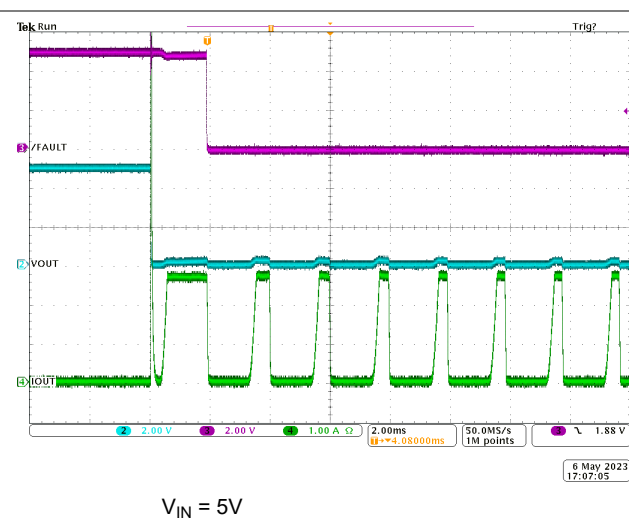
图 8-7. TPS2001E 空载至输出短路
