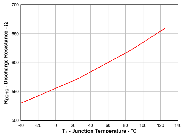
图 6-8. 输出放电电阻与温度之间的关系
