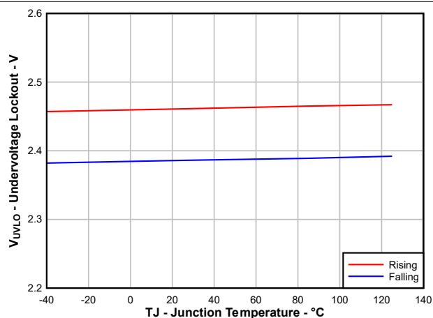
图 6-17. 欠压锁定与温度间的关系
