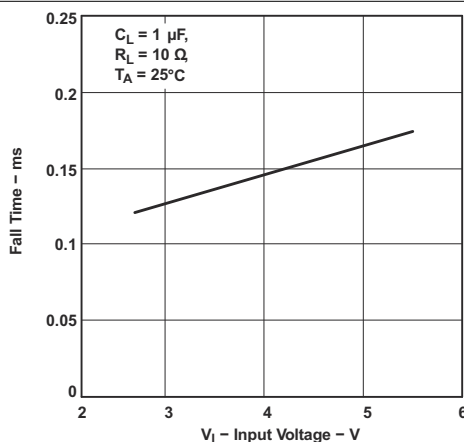
图 6-4. Fall Time vs Input Voltage
