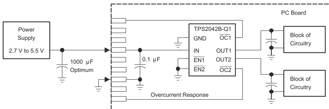
图 9-15. Example Hot-Plug Implementation (TPS2042B-Q1)
