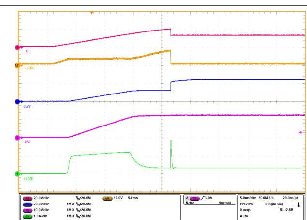
图 9-20. 输出端为 1000\mu\text{F} 且负载为 0.5\text{A} 时的浪涌电流曲线 (LPM = 低电平)
