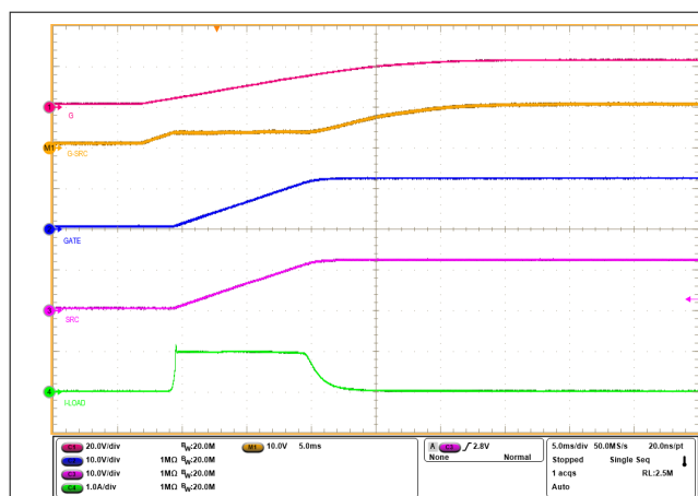
图 9-19. 输出端为 1000\mu\text{F} 时的浪涌电流曲线 ( \overline{\text{LPM}} = 低电平)
