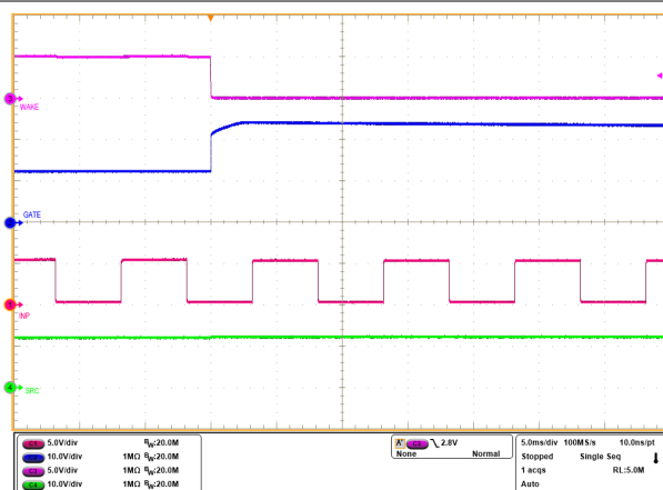
图 9-5. 当负载唤醒状态下 \overline{\text{LPM}} = 低电平时, INP 无法控制 GATE
