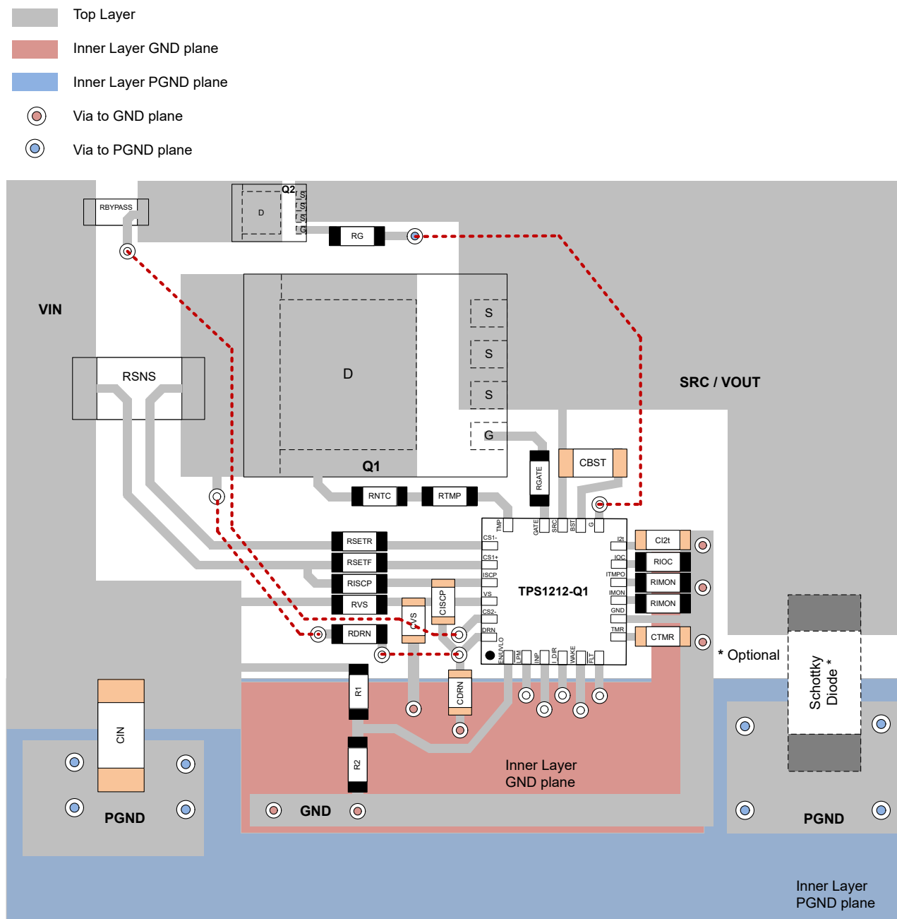
图 9-20. TPS1212-Q1 的典型 PCB 布局布线示例
