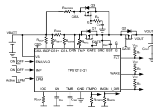
驱动 PAAT 负载、具有负载唤醒和大容量电容器充电功能的 TPS12120-Q1 应用电路
