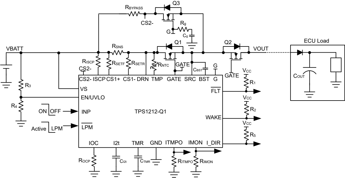
图 9-16. 使用自动负载唤醒和输出大容量电容器充电功能来驱动全时供电 (PAAT) 负载的 TPS1212-Q1 应用电路
