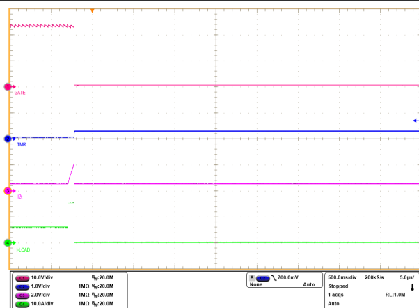
图 9-11. TPS1212-Q1 在 I^2t 过流故障下的闭锁响应
