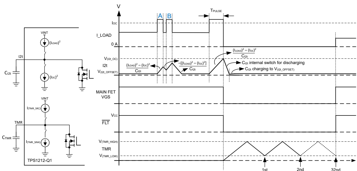
图 8-9. 具有自动重试功能的 I2t 过流保护
