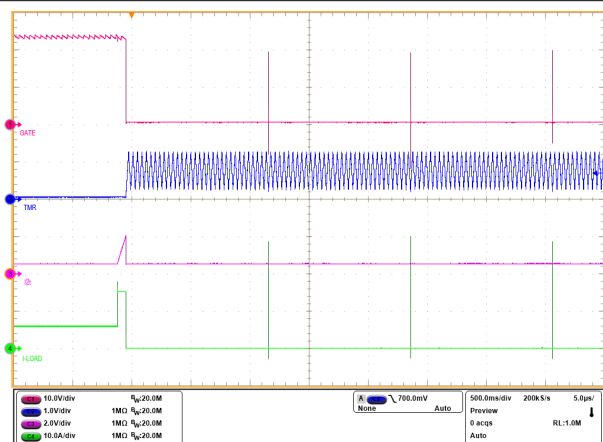
图 9-10. TPS1212-Q1 在 I^2t 过流故障下的自动重试响应
