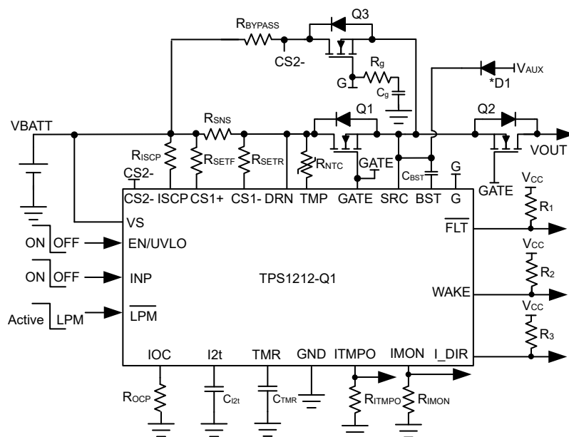
图 8-3. 采用 BST 外部供电的 TPS1212-Q1 应用电路
