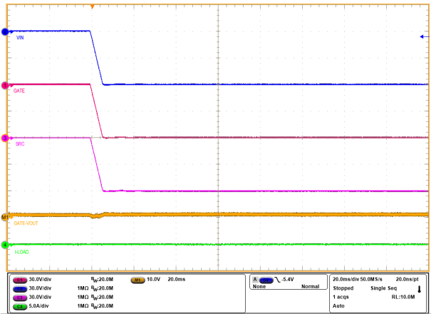
图 9-15. 输入电池反向故障下的 GATE 关断
