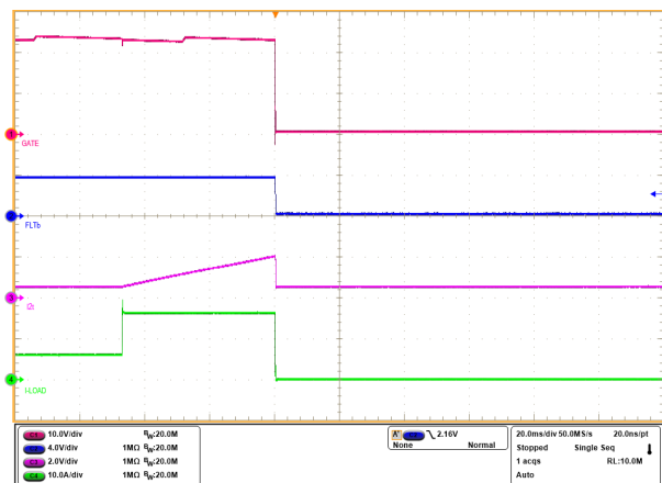
图 9-8. 6A 至 16A 负载阶跃下 TPS1212-Q1 EVM 基于 I^2t 的过流响应
