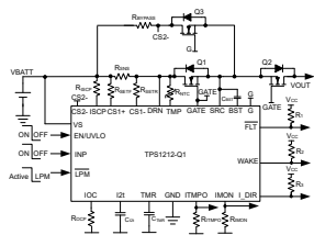
驱动 PAAT 负载、具有负载唤醒的 TPS12120-Q1 应用电路
