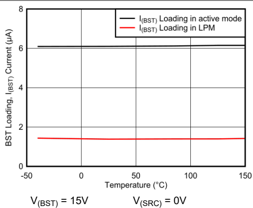
图 6-7. BST 负载电流 ( I_{BST} ) 与温度间的关系
