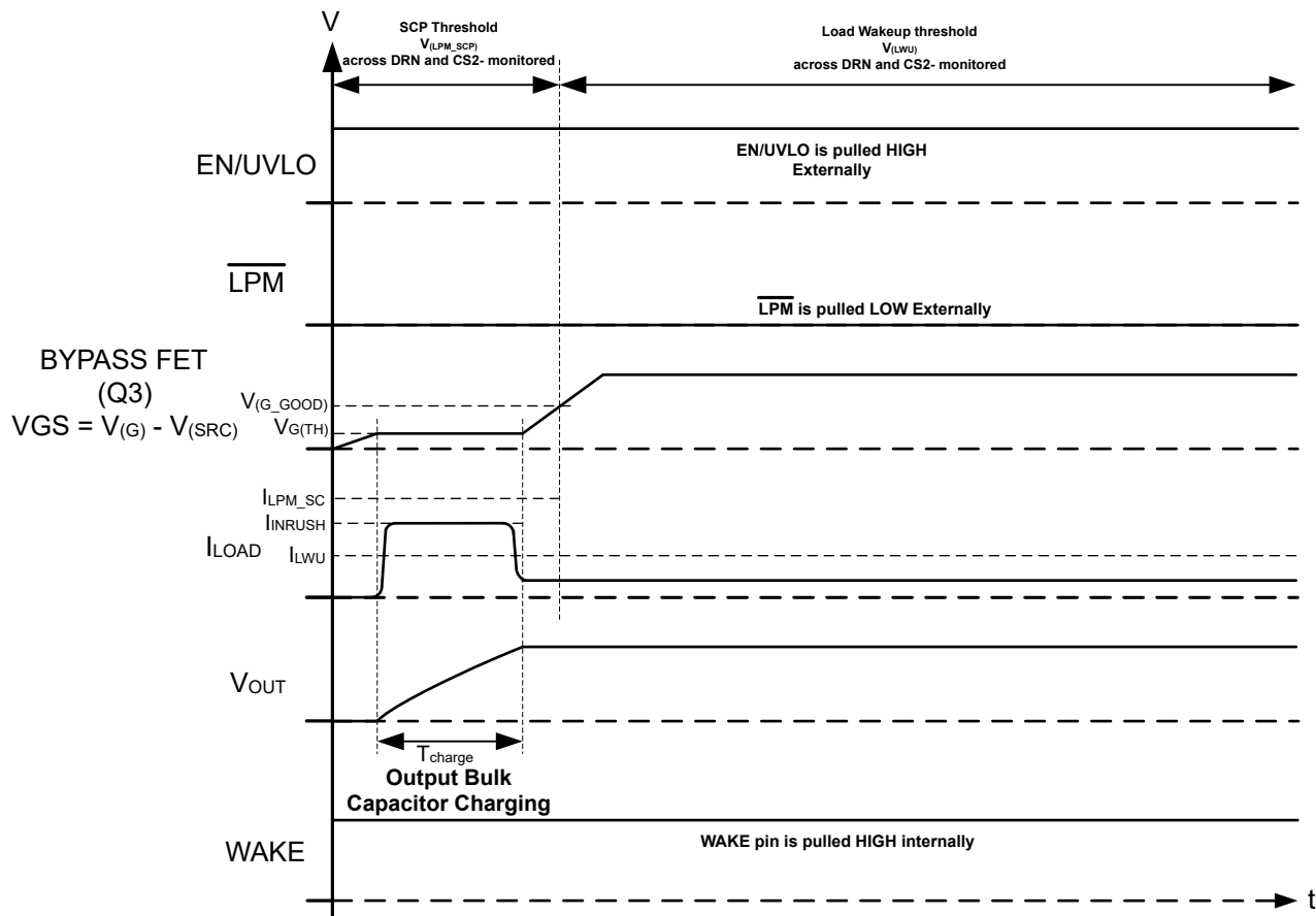
图 8-5. 使用旁路路径的大容量电容器充电的时序图
