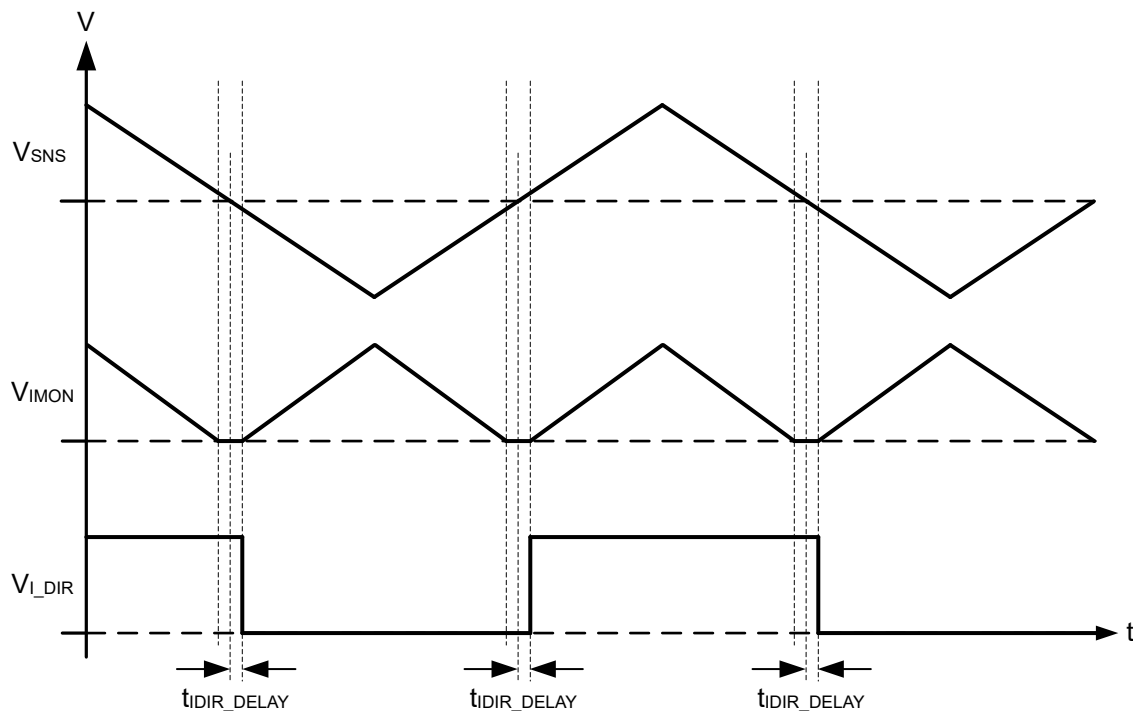
图 8-11. TPS1212-Q1 双向电流监测时序图
