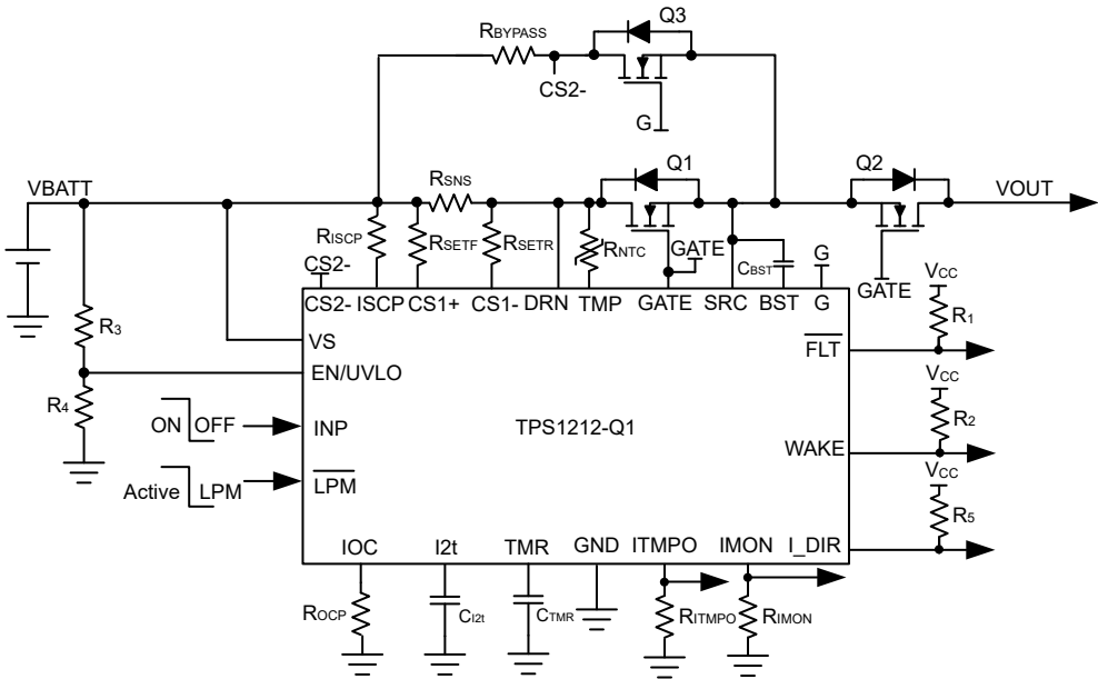
图 9-1. 使用自动负载唤醒功能来驱动全时供电 (PAAT) 负载的 TPS1212-Q1 应用电路
