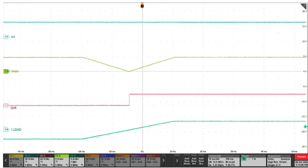
图 9-14. TPS1212-Q1 双向电流监测输出 ( IMON、 I_DIR ) 瞬态响应
