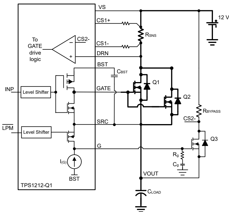
图 8-4. 使用低功耗旁路 FET 栅极 (G) 压摆率控制的电容器充电
