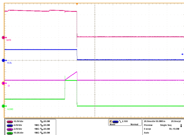
图 9-9. 6A 至 23A 负载阶跃下 TPS1212-Q1 EVM 基于 I^2t 的过流响应
