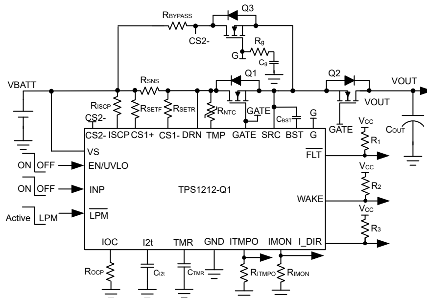
图 8-6. 使用低功耗旁路 FET (Q3) 和串联电阻器 ( R_{BYPASS} ) 的容性负载驱动 TPS1212-Q1 应用电路
