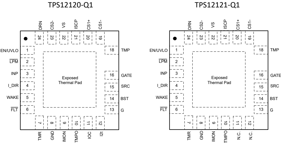
图 5-1. RGE 封装，23 引脚 VQFN (透明顶视图)
