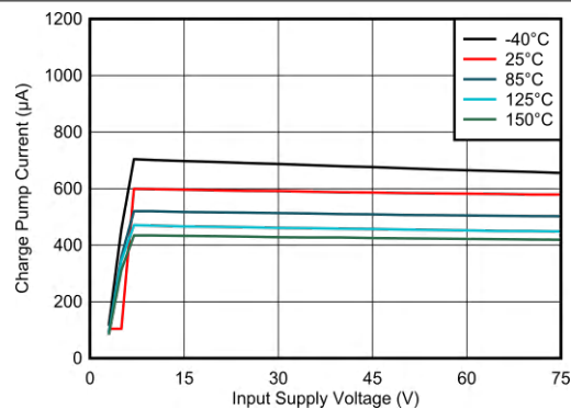
图 6-4. 电荷泵电流与电源电压间的关系
