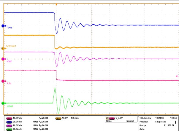
图 9-12. TPS1212-Q1 的输出短路响应
