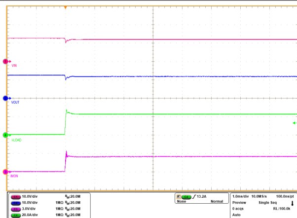
图 9-13. TPS1212-Q1 电流监测输出 (IMON) 瞬态响应
