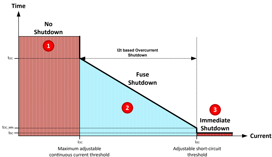
图 8-8. TPS1212-Q1 的可配置电流与时间特性曲线
