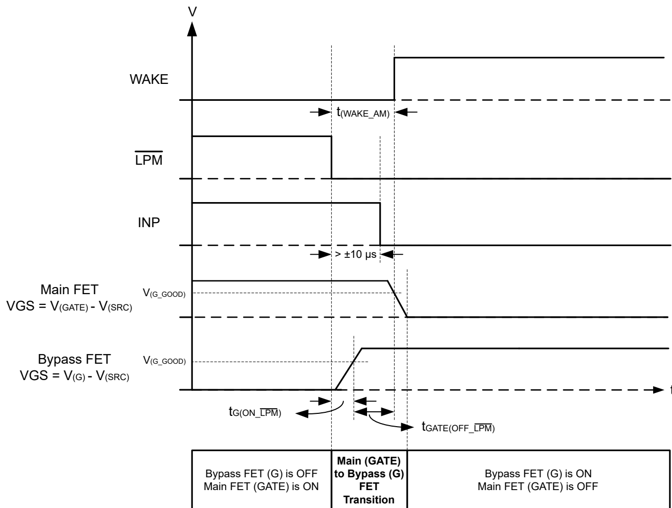
图 8-17. 从工作模式进入低功耗模式的 LPM 和 INP 信号时序控制注意事项
