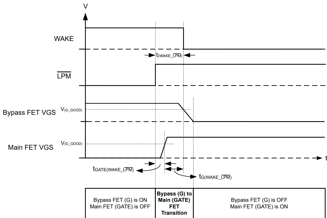
图 7-2. 通过 \overline{LPM} 外部触发器将系统从低功耗模式唤醒至工作模式
