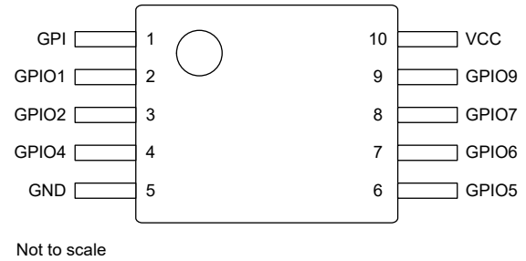
图 4-2. DGS 封装，10 引脚 VSSOP (俯视图)
