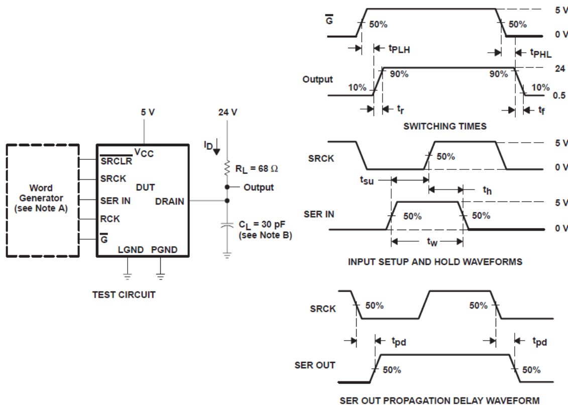
图 6-1. 电阻负载运行
