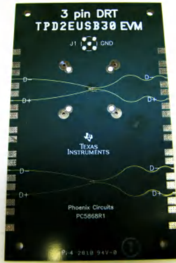
图 10-3. TPDxEUSB30/A EVM - TPD2EUSB30/A Side
