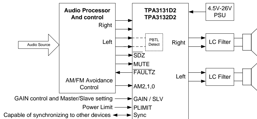
简化应用电路
