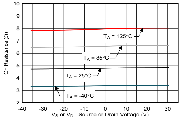
图 10-3. R_{ON} Flatness
