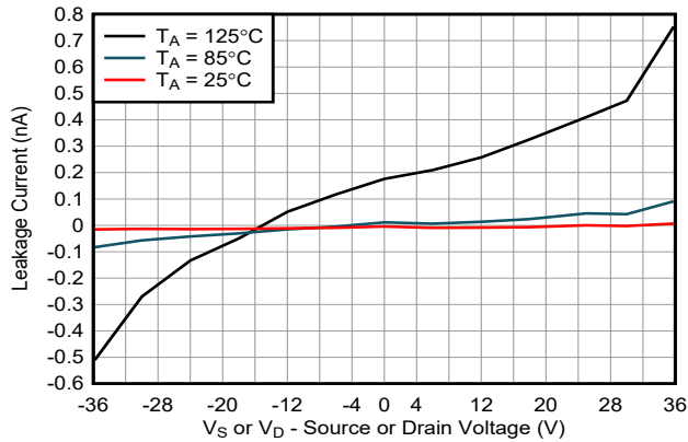
图 10-2. On-Leakage
