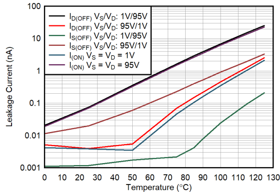
图 10-2. Leakage Current
