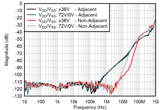
图 10-3. Crosstalk
