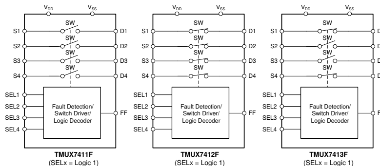
功能方框图
