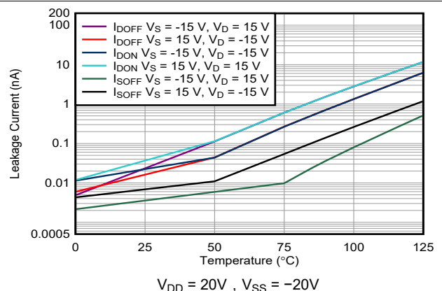
图 7-18. 泄漏电流与温度间的关系
