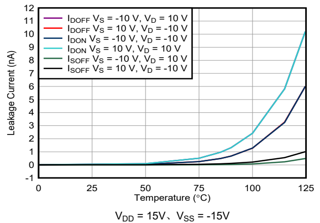
图 7-14. 泄漏电流与温度间的关系
