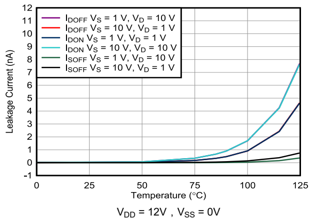
图 7-13. 泄漏电流与温度间的关系
