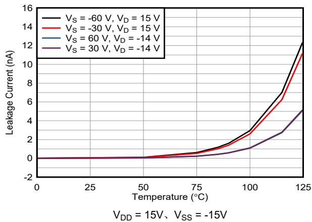
图 7-19. I_{D(FA)} 过压漏电流与温度的关系
