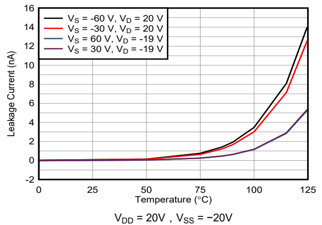
图 7-20. I_{D(FA)} 过压漏电流与温度的关系
