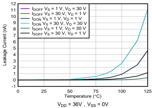
图 7-15. 泄漏电流与温度间的关系
