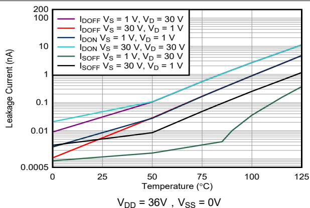
图 7-17. 泄漏电流与温度间的关系
