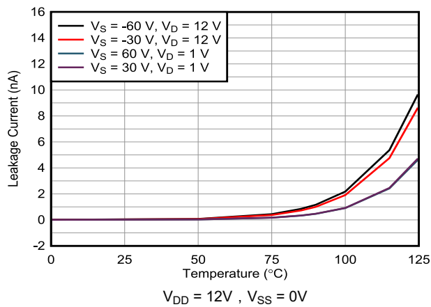
图 7-21. I_{D(FA)} 过压漏电流与温度的关系
