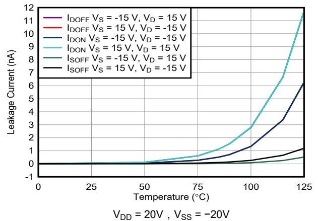
图 7-16. 泄漏电流与温度间的关系
