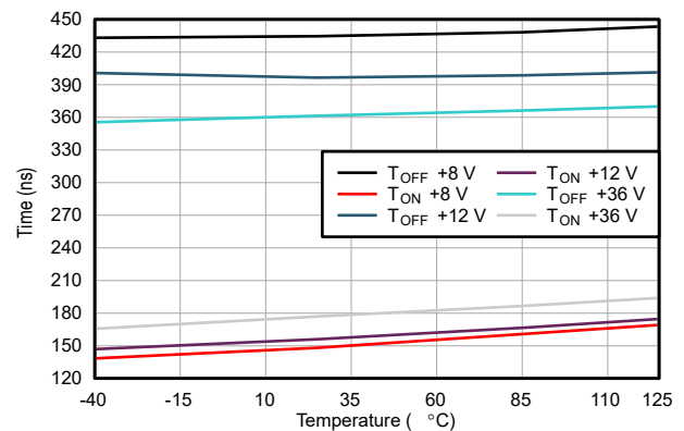
图 7-28. 转换时间与温度间的关系
