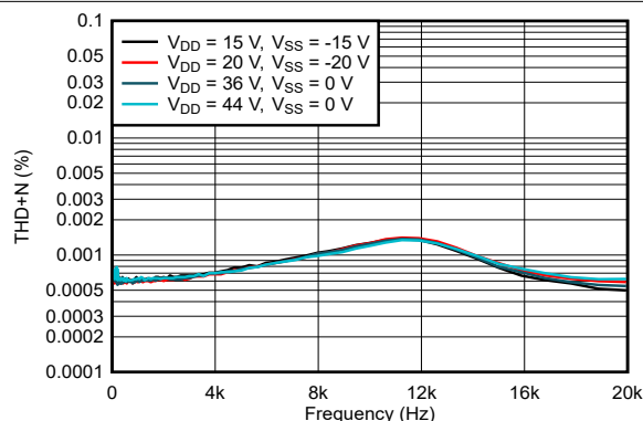
图 6-25. THD+N 与频率间的关系
