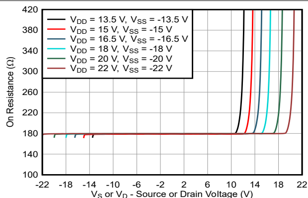
图 6-2. 导通电阻与源极或漏极电压之间的关系
