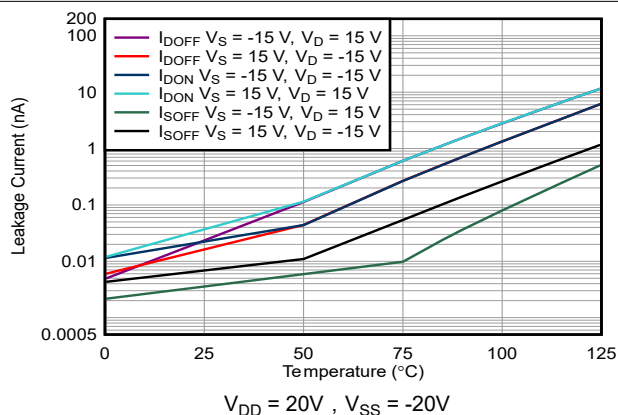
图 6-19. 漏电流与温度间的关系
