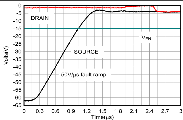
图 6-38. 漏极输出恢复 - 负过压
