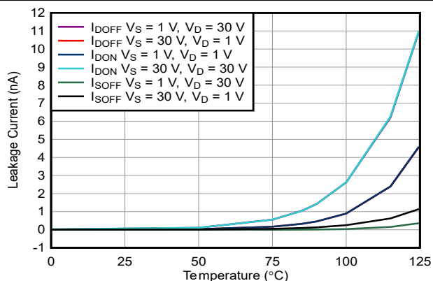
图 6-14. 漏电流与温度间的关系
