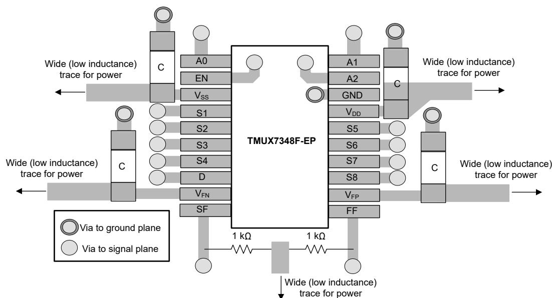
图 9-4. TMUX7348F-EP 布局示例
