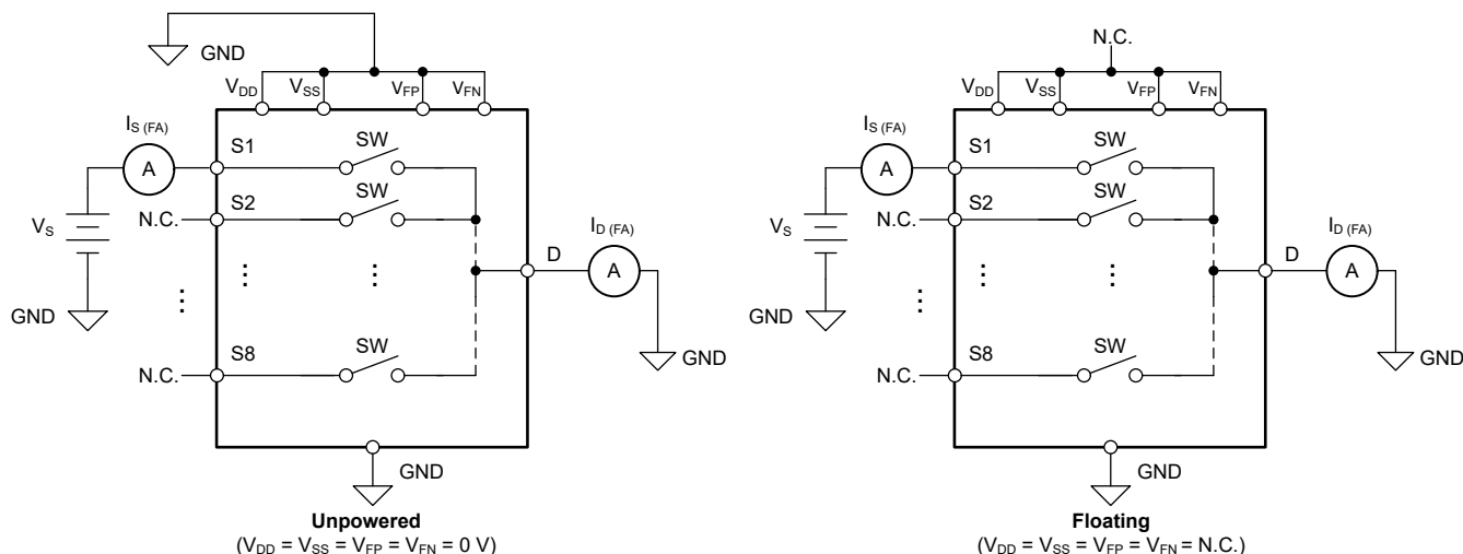
图 7-5. 无电源或浮动电源过压故障下输入和输出漏电流的测量设置
