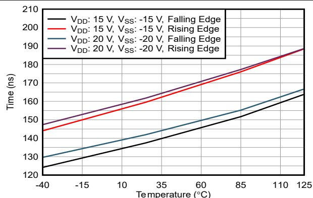
图 6-28. 转换时间与温度间的关系
