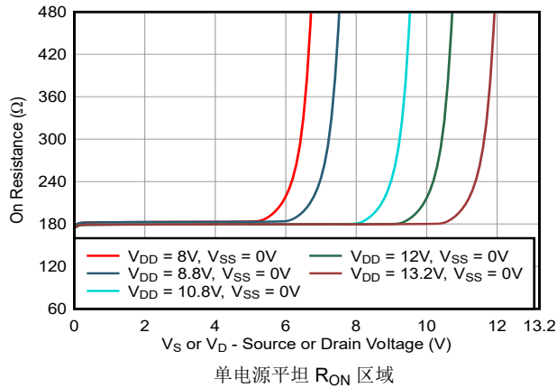
图 6-7. 导通电阻与源极或漏极电压之间的关系
