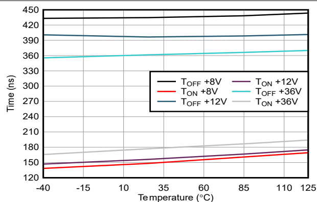
图 6-31. 开启和关闭时间与温度的关系
