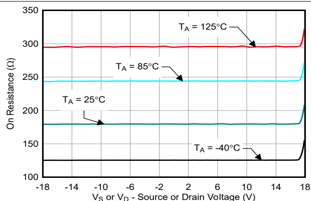
图 6-3. 导通电阻与源极或漏极电压之间的关系
