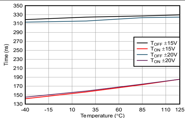
图 6-30. 开启和关闭时间与温度的关系
