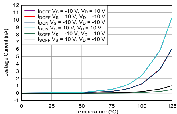
图 6-15. 漏电流与温度间的关系
