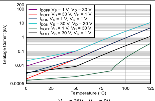
图 6-18. 漏电流与温度间的关系
