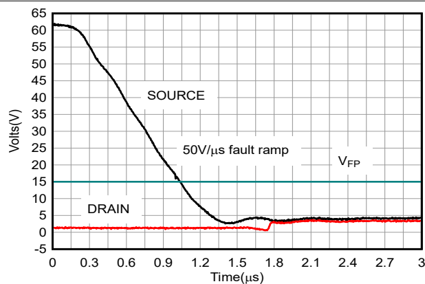
图 6-37. 漏极输出恢复 - 正过压
