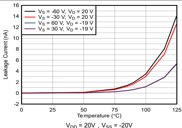
图 6-21. I_{D(FA)} 过压漏电流与温度的关系
