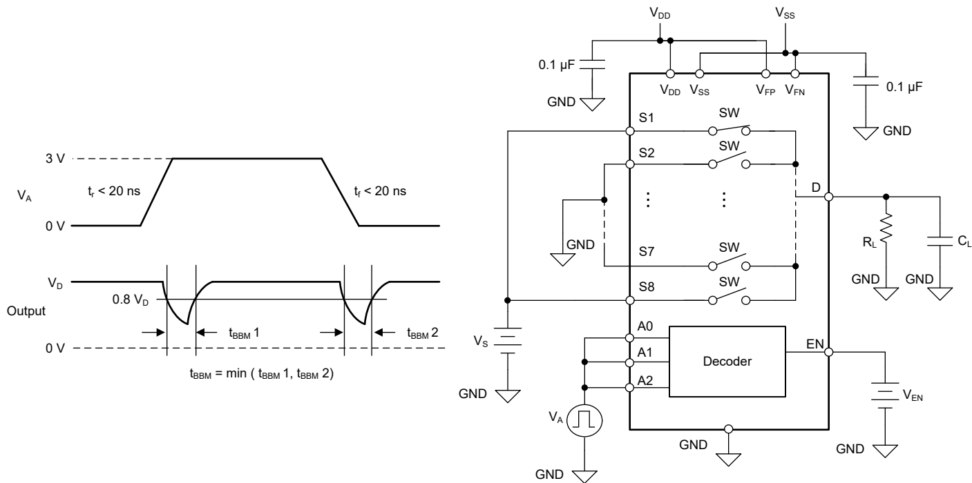
图 7-6. 先断后合延迟测量设置
