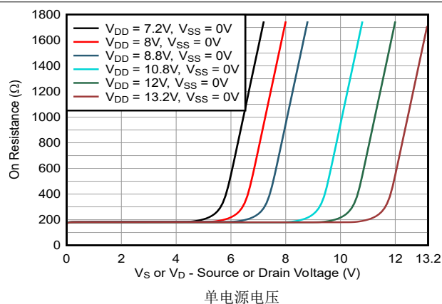
图 6-6. 导通电阻与源极或漏极电压之间的关系
