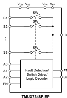
功能方框图
