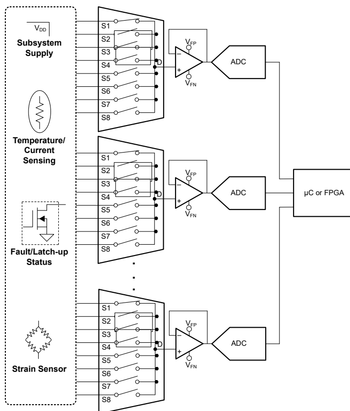
图 9-1. 典型应用
