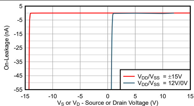
源极/漏极电压与导通漏电流间的关系
