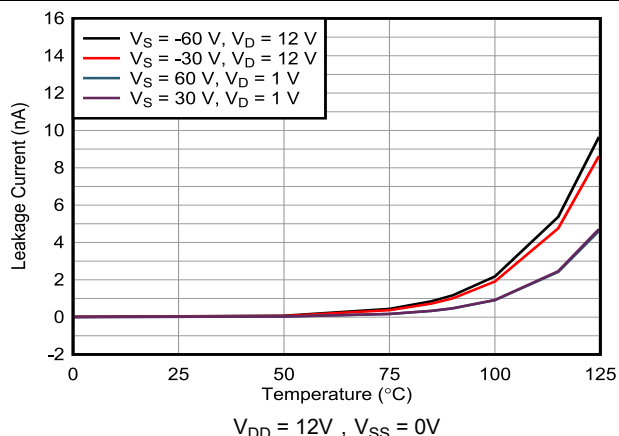
图 6-22. I_{D(FA)} 过压漏电流与温度的关系
