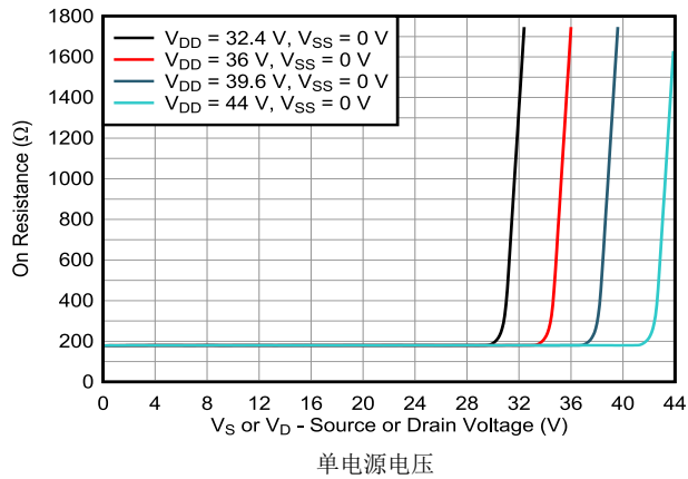
图 6-9. 导通电阻与源极或漏极电压之间的关系
