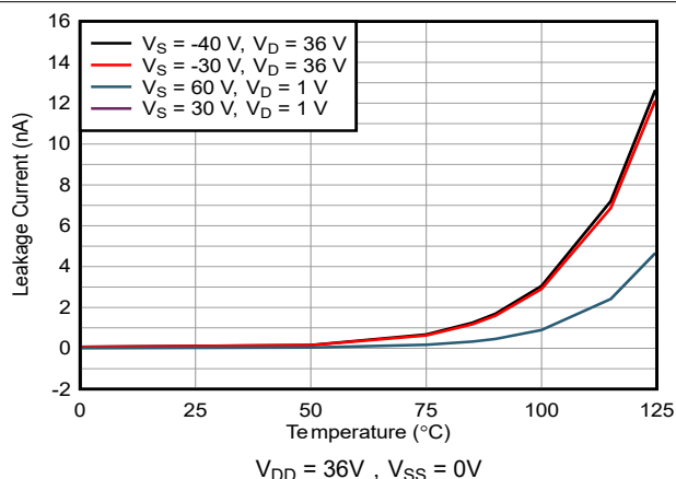
图 6-23. I_{D(FA)} 过压漏电流与温度的关系
