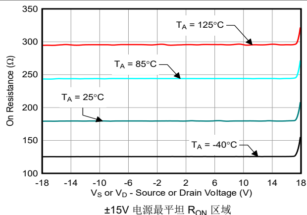
图 6-4. 导通电阻与源极或漏极电压之间的关系
