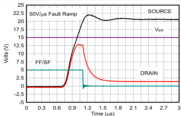
图 6-35. 漏极输出响应 - 正过压
