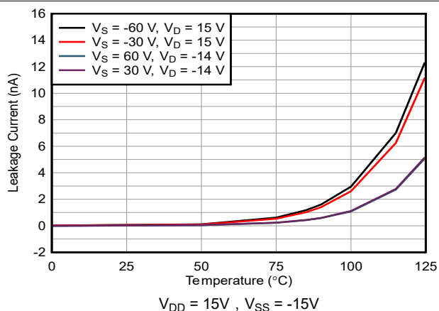
图 6-20. I_{D(FA)} 过压漏电流与温度的关系
