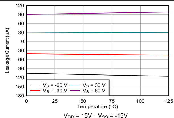
图 6-24. I_{S(FA)} 过压漏电流与温度的关系
