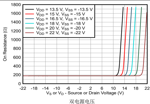
图 6-1. 导通电阻与源极或漏极电压之间的关系
