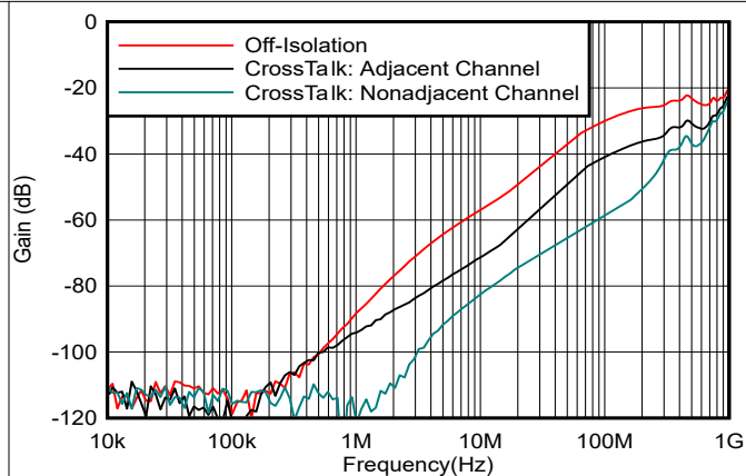
图 6-32. 关断隔离和串扰与频率间的关系
