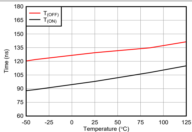
图 5-20. T_{\text{ON (EN)}} and T_{\text{OFF (EN)}} vs Temperature
