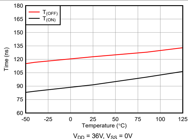
图 5-21. T_{\text{ON (EN)}} and T_{\text{OFF (EN)}} vs Temperature
