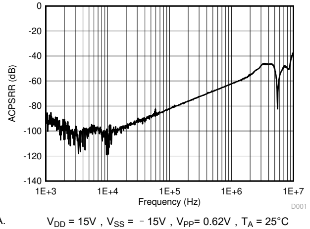
图 6-14. ACPSRR 与频率间的关系
