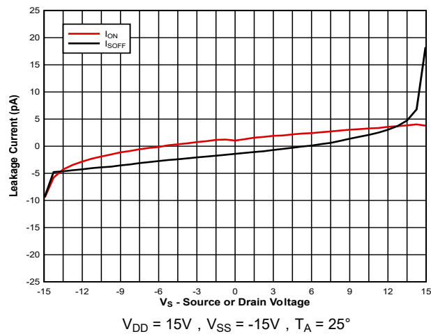
图 5-5. 漏电流与偏置电压间的关系
