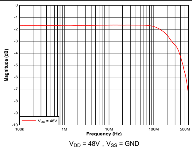
图 5-8. 48V 带宽与频率间的关系
