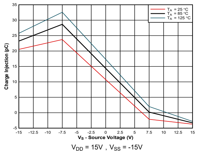
图 5-6. 电荷注入与源极电压间的关系
