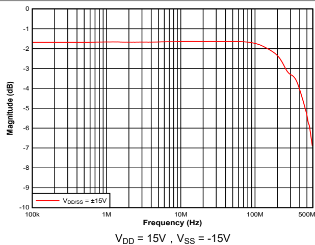
图 5-7. \pm 15\text{V} 带宽与频率间的关系
