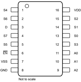
图 6-2. TMUX4051-Q1 DYY 封装，16 引脚 SOT-23-THIN (顶视图)
