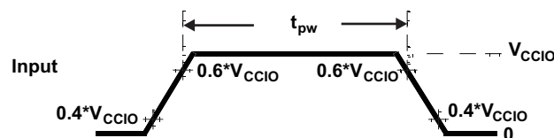
图 7-17. FlexRay Inputs
