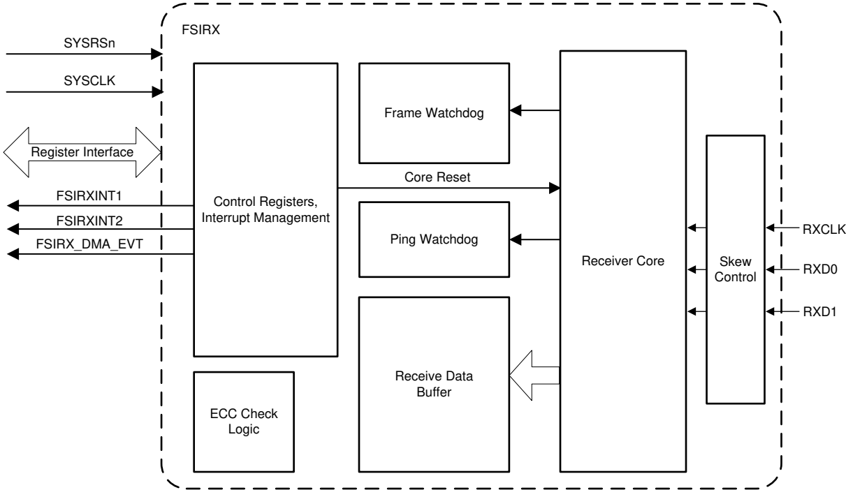
图 6-91. FSIRX 方框图
