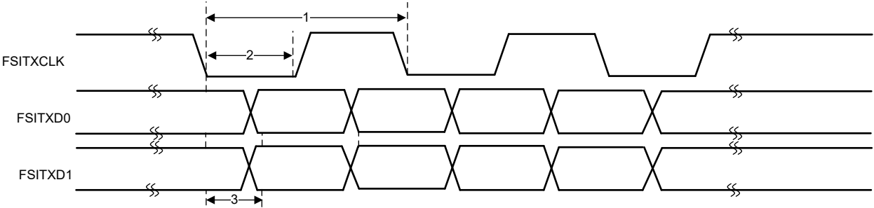
图 6-89. FSITX 时序
