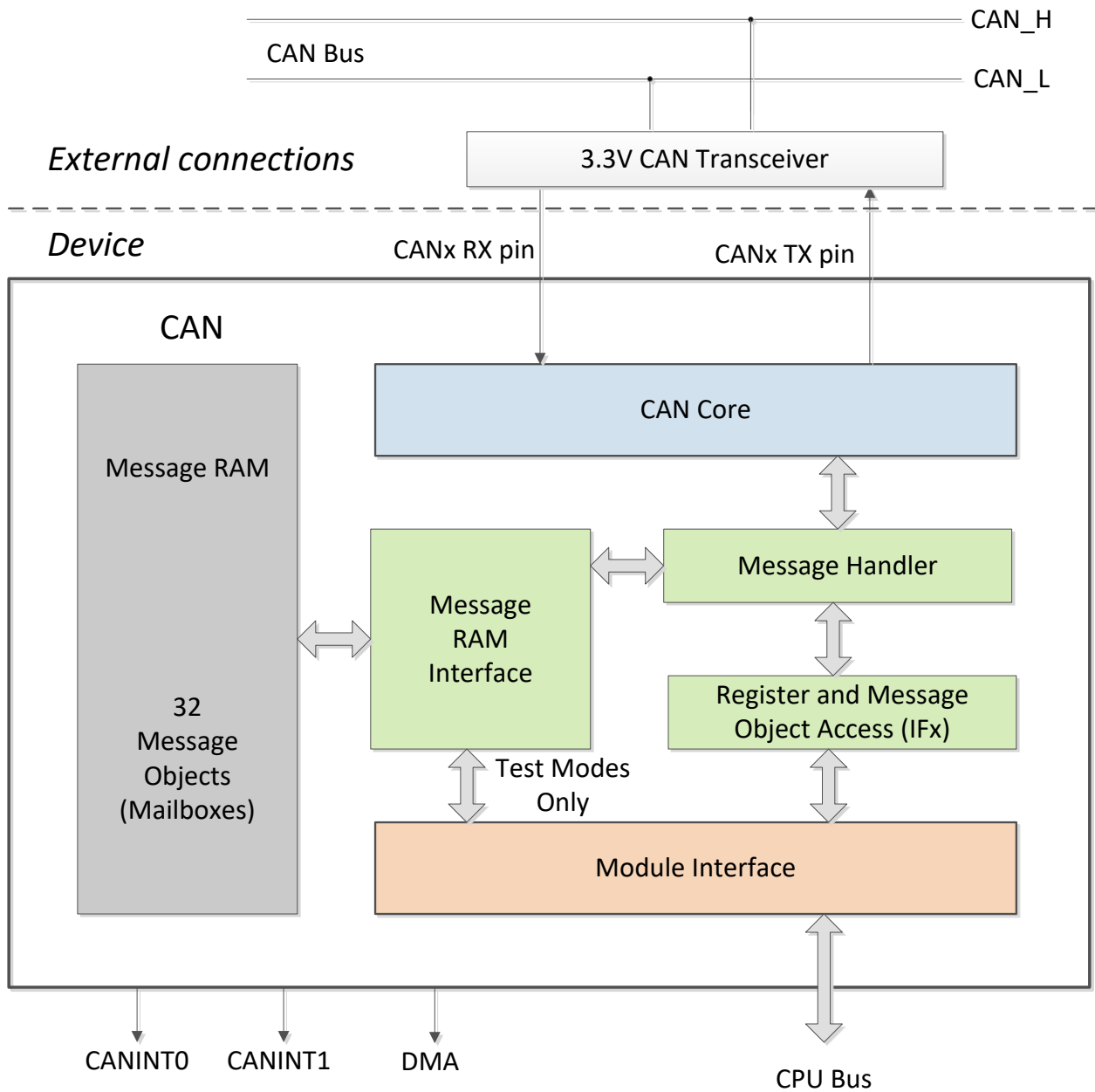
图 6-85. CAN 方框图
