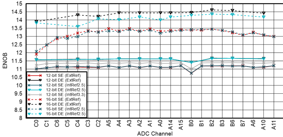
图 6-53. 100 引脚 PZP 的每通道 ENOB
