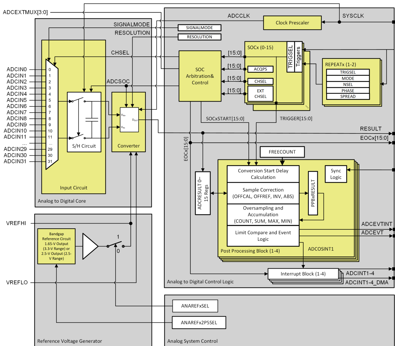
图 6-49. ADC 模块方框图
