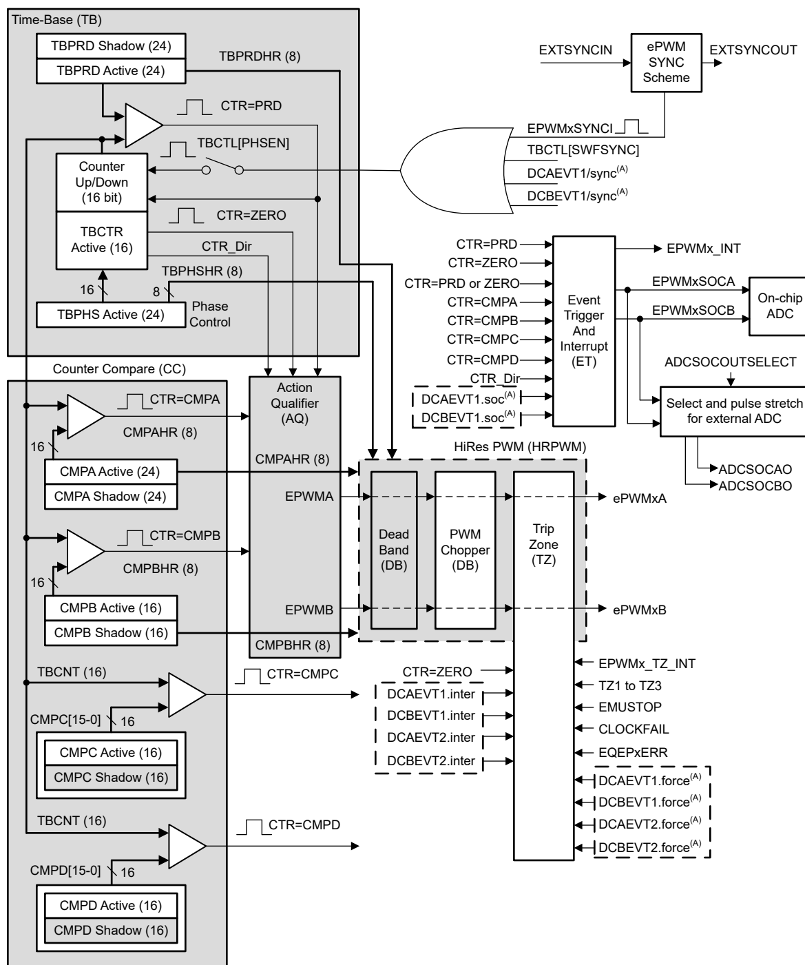
图 6-56. ePWM 子模块和关键内部信号互连
