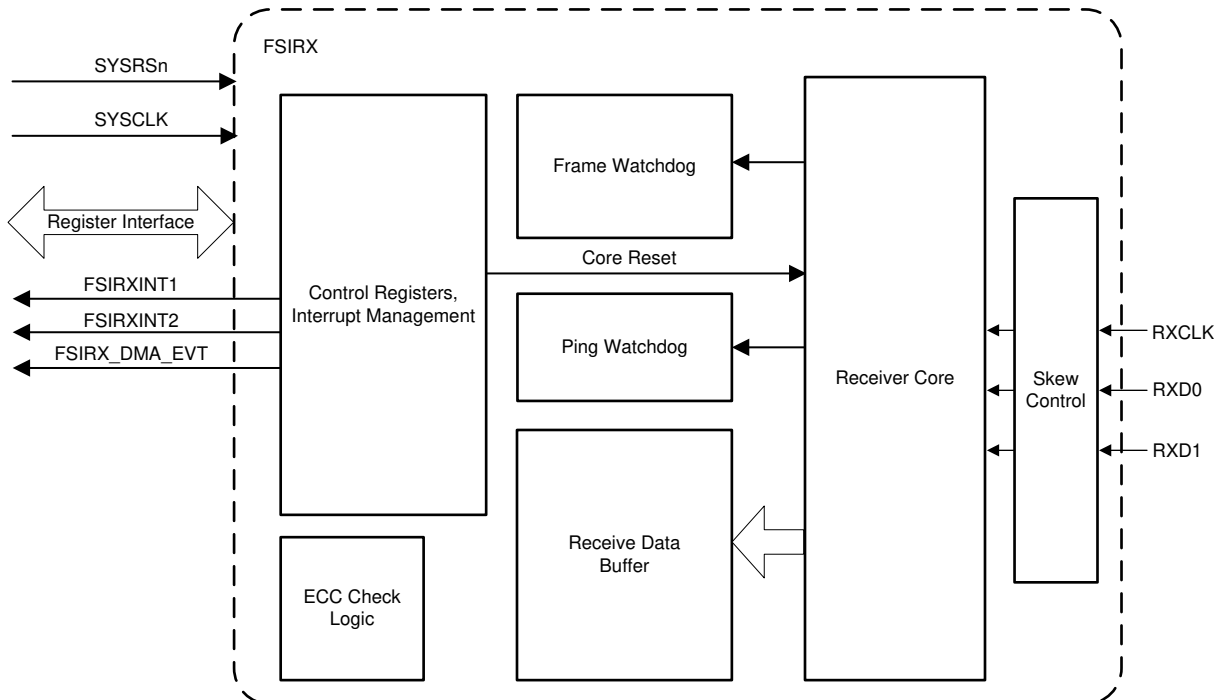
图 6-79. FSIRX 方框图
