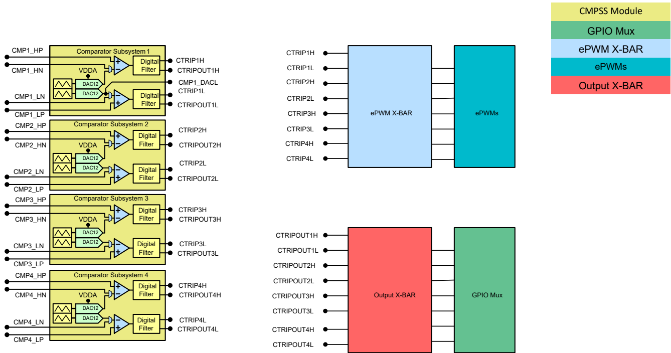
图 6-48. CMPSS 连接
