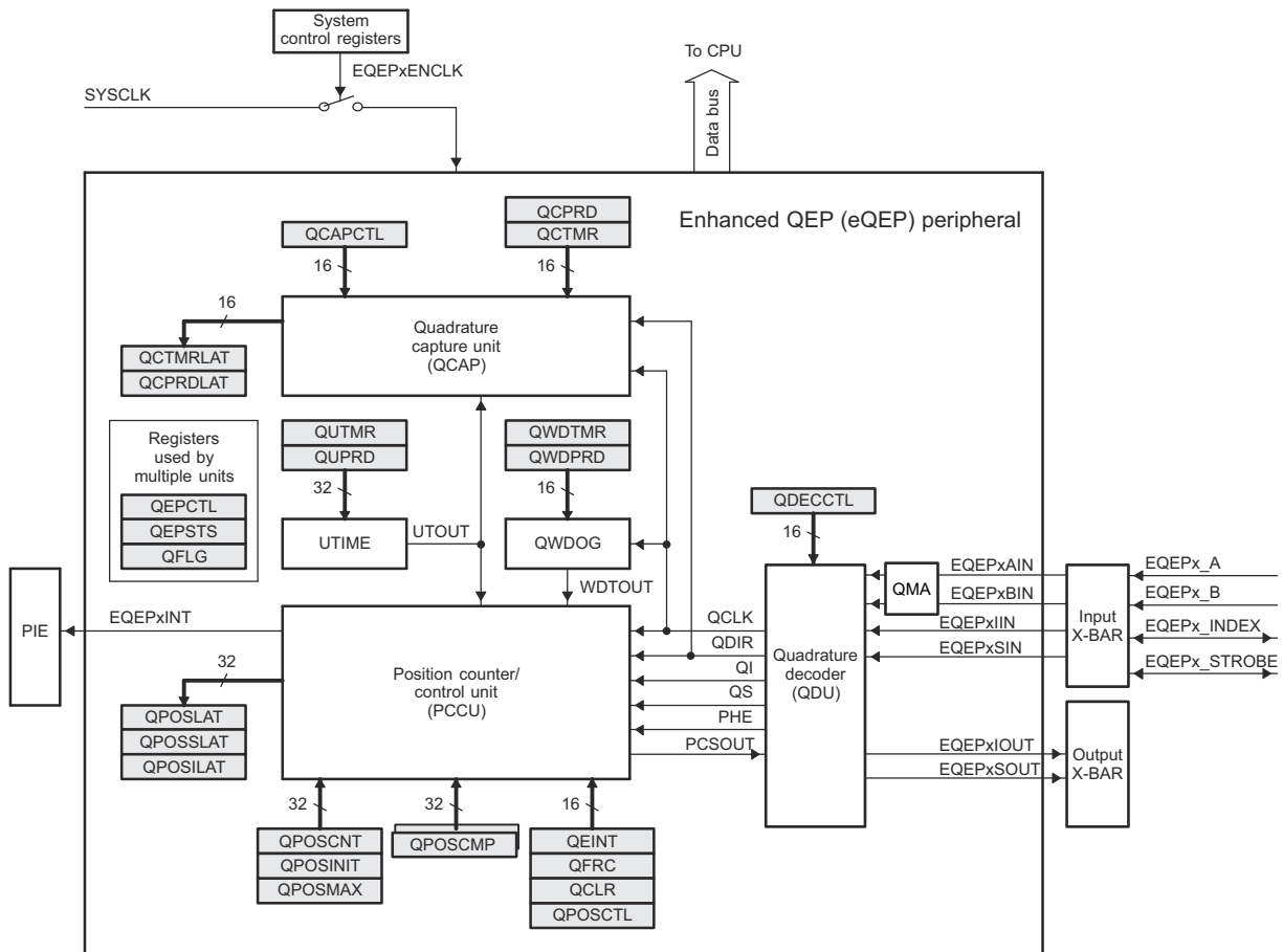
图 6-65. eQEP 方框图
