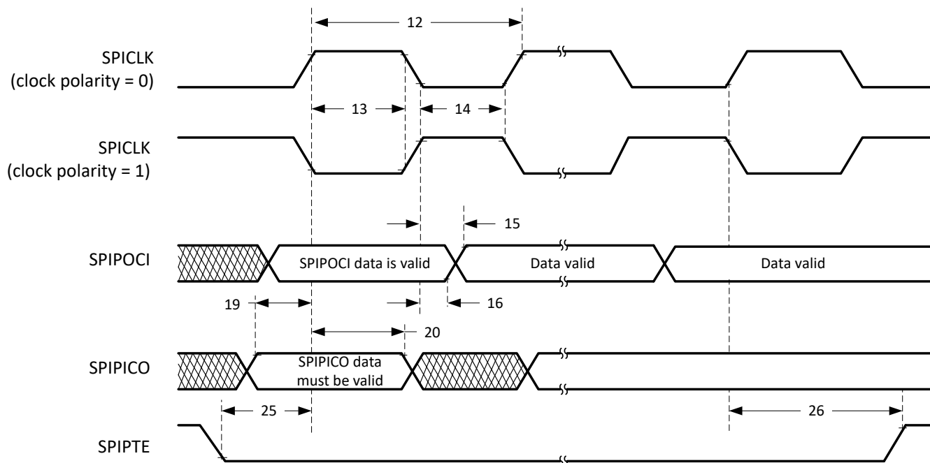
图 6-77. SPI 外设模式外部时序 (时钟相位 = 1)
