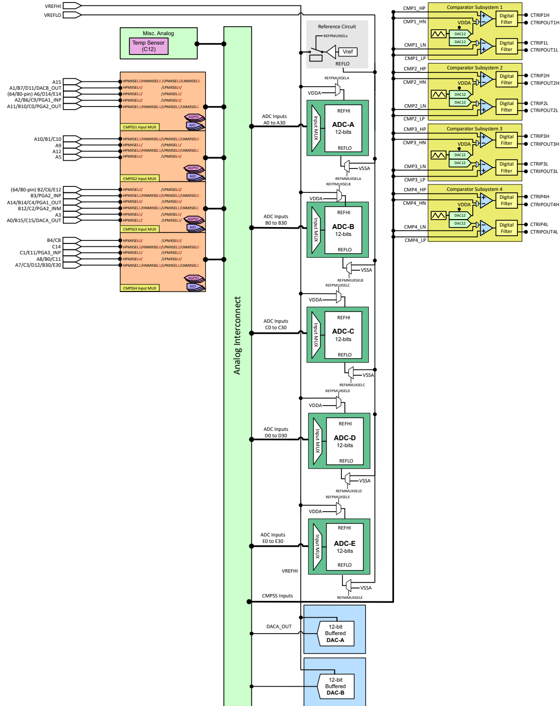
图 6-34. 模拟子系统方框图 ( 80/64/56 引脚封装 )
