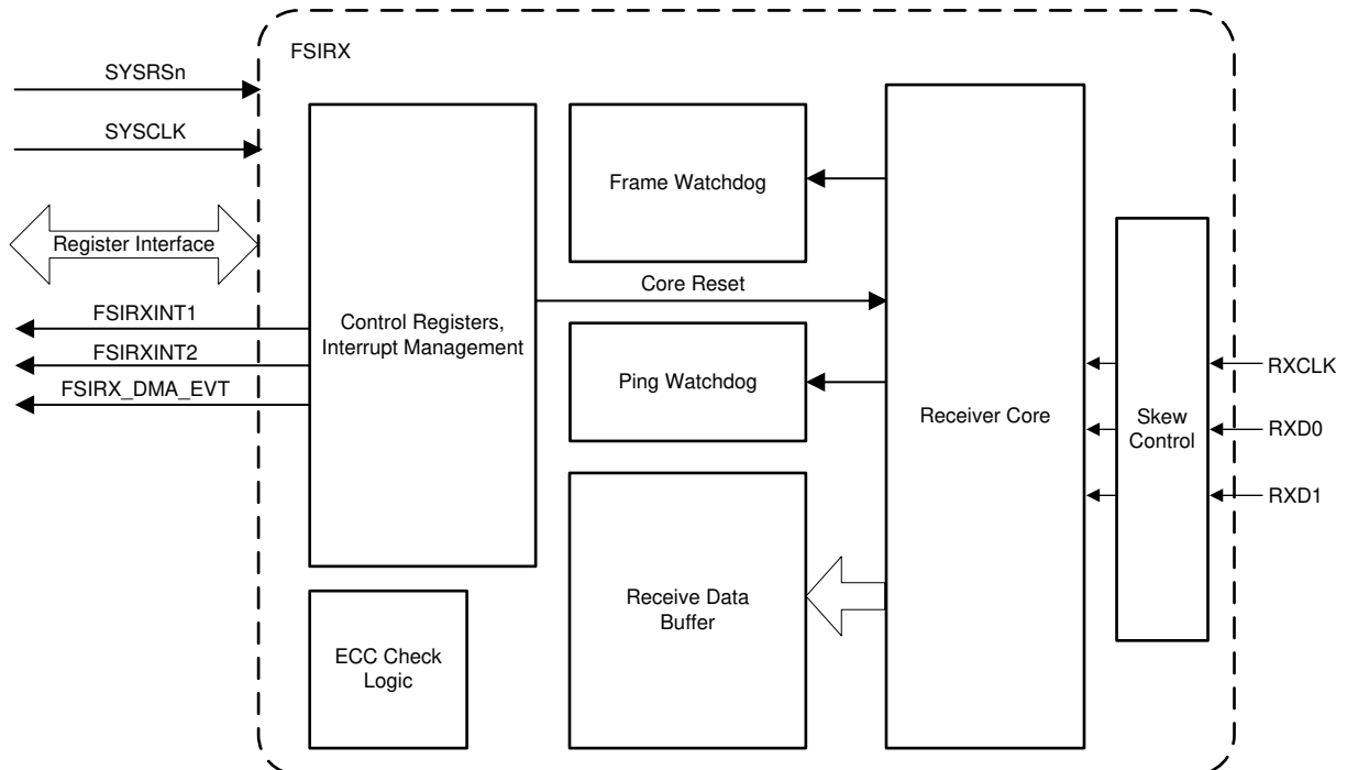
图 6-83. FSIRX 方框图
