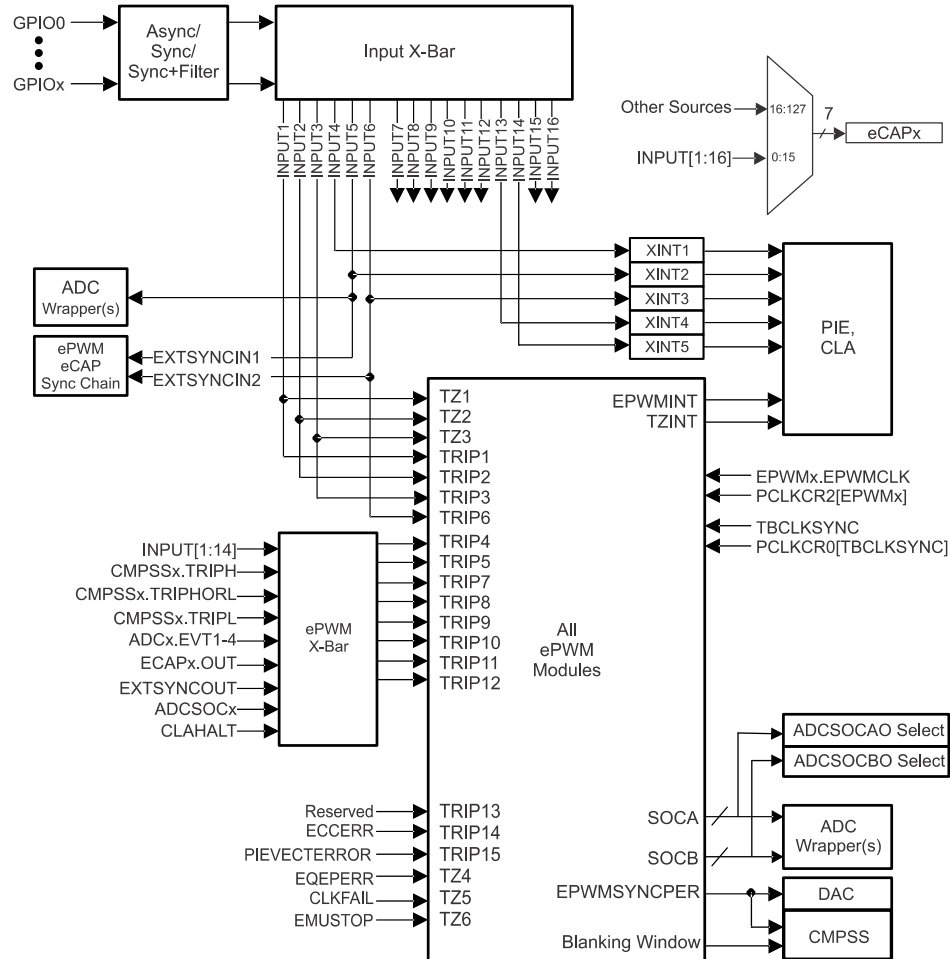
图 6-59. ePWM 跳变输入连接
