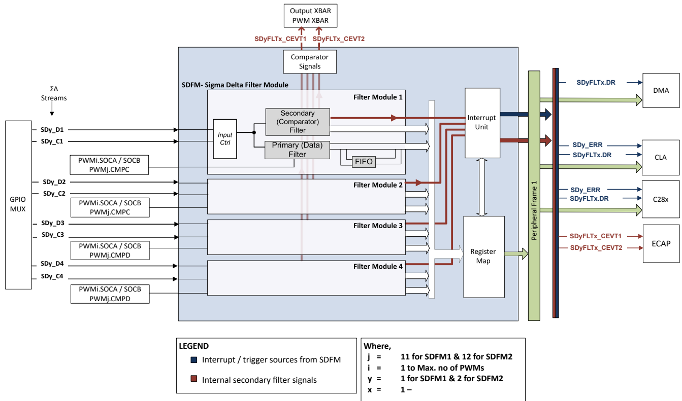
图 6-66. \Sigma - \Delta 滤波器模块 (SDFM) 方框图
