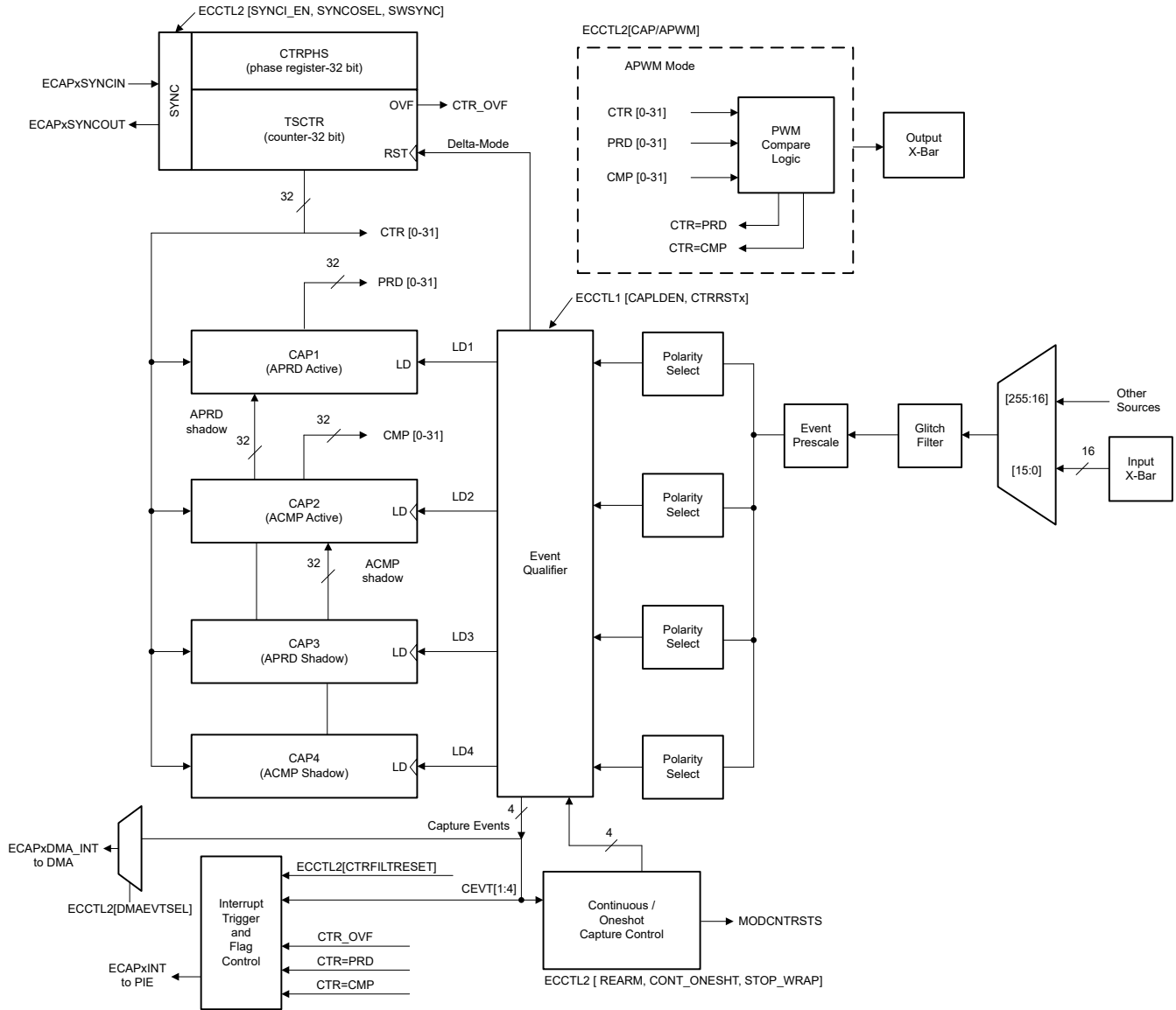
图 6-63. eCAP 方框图
