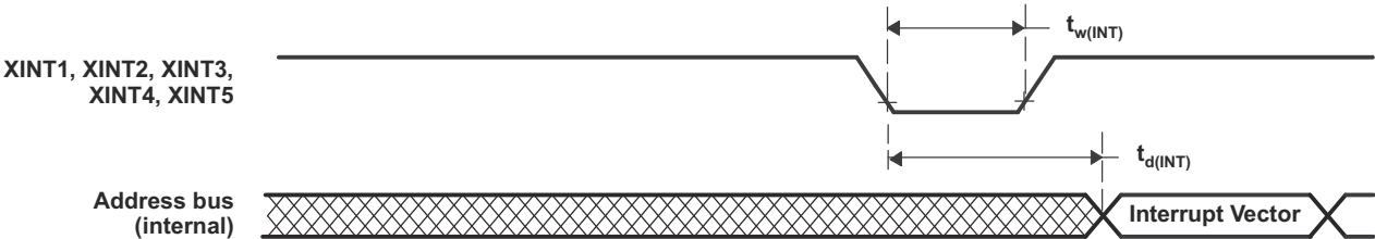
图 6-30. 外部中断时序
