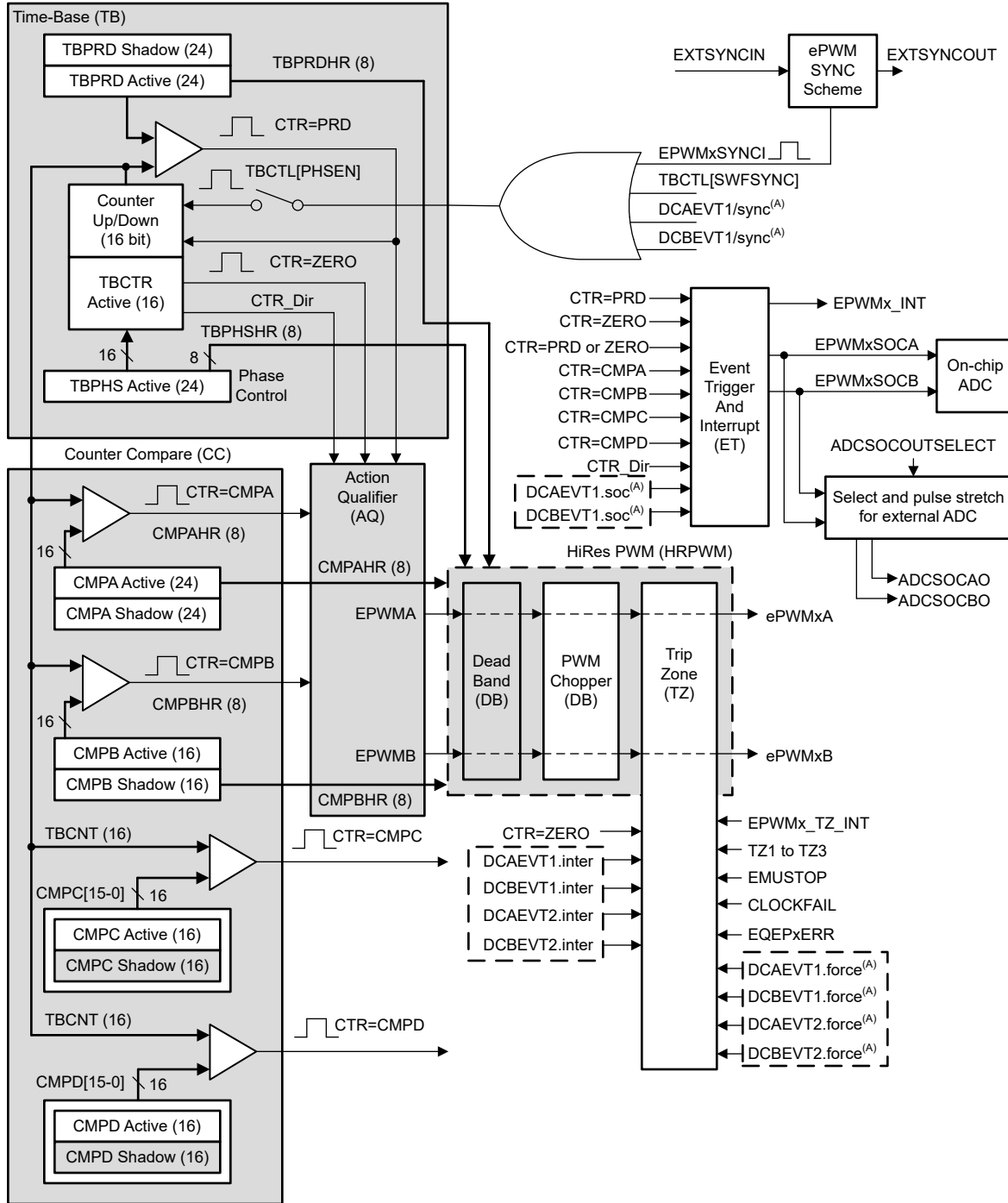
图 6-58. ePWM 子模块和关键内部信号互连
