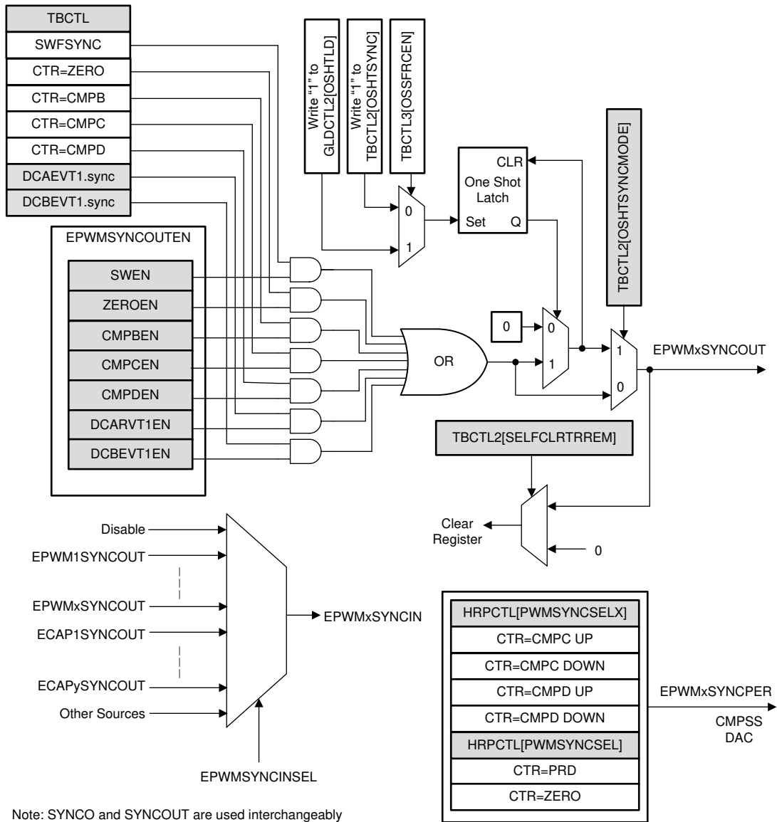
图 6-60. 同步链架构
