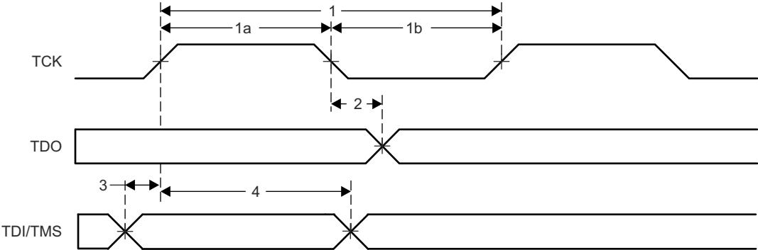
图 6-24. JTAG 时序
