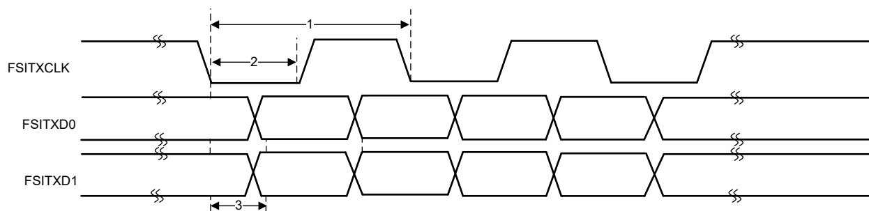
图 6-81. FSITX 时序
