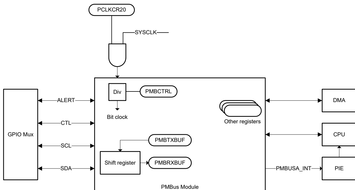
图 6-71. PMBus 方框图
