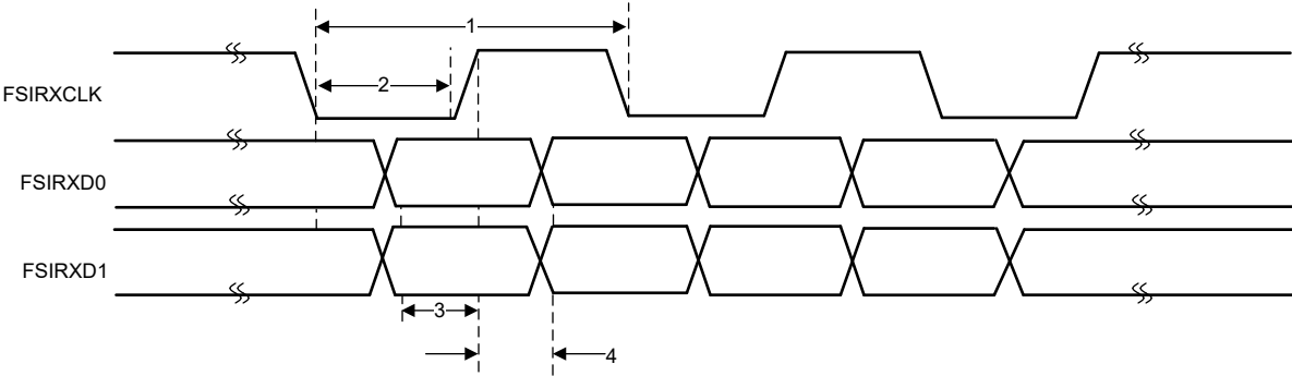
图 6-84. FSIRX 时序
