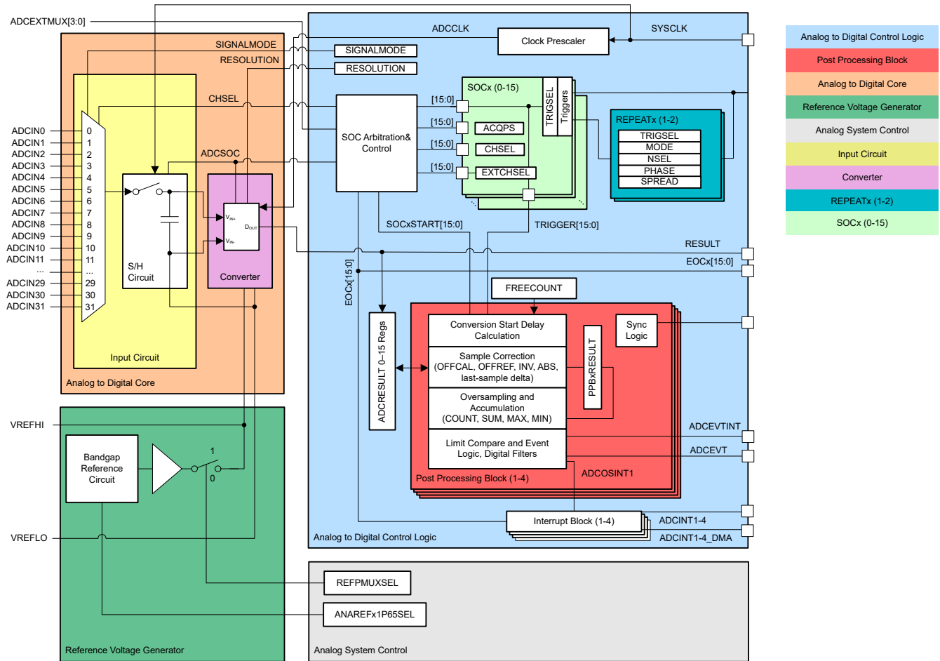
图 6-37. ADC 模块方框图
