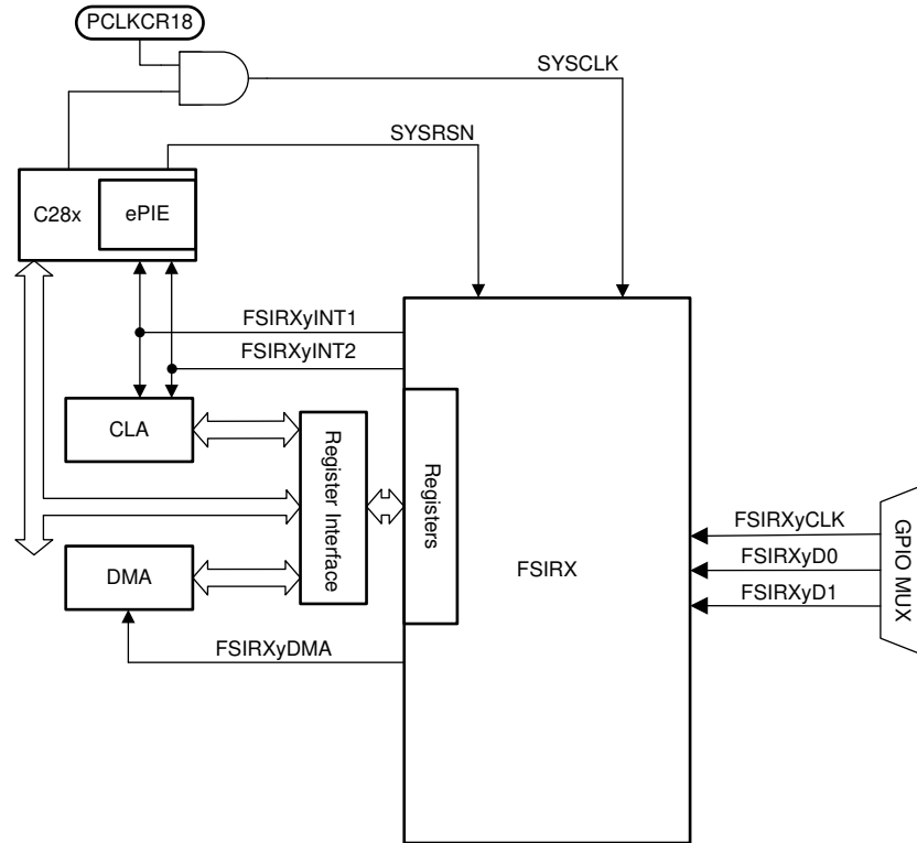
图 6-82. FSIRX CPU 接口
