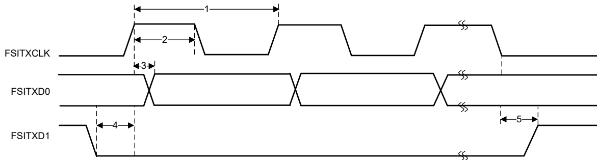
图 6-85. FSITX SPI 信令模式时序
