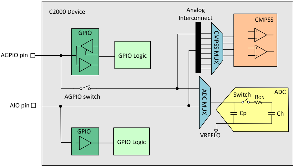
图 5-8. 具有 AGPIO 实现方式的模拟子系统方框图
