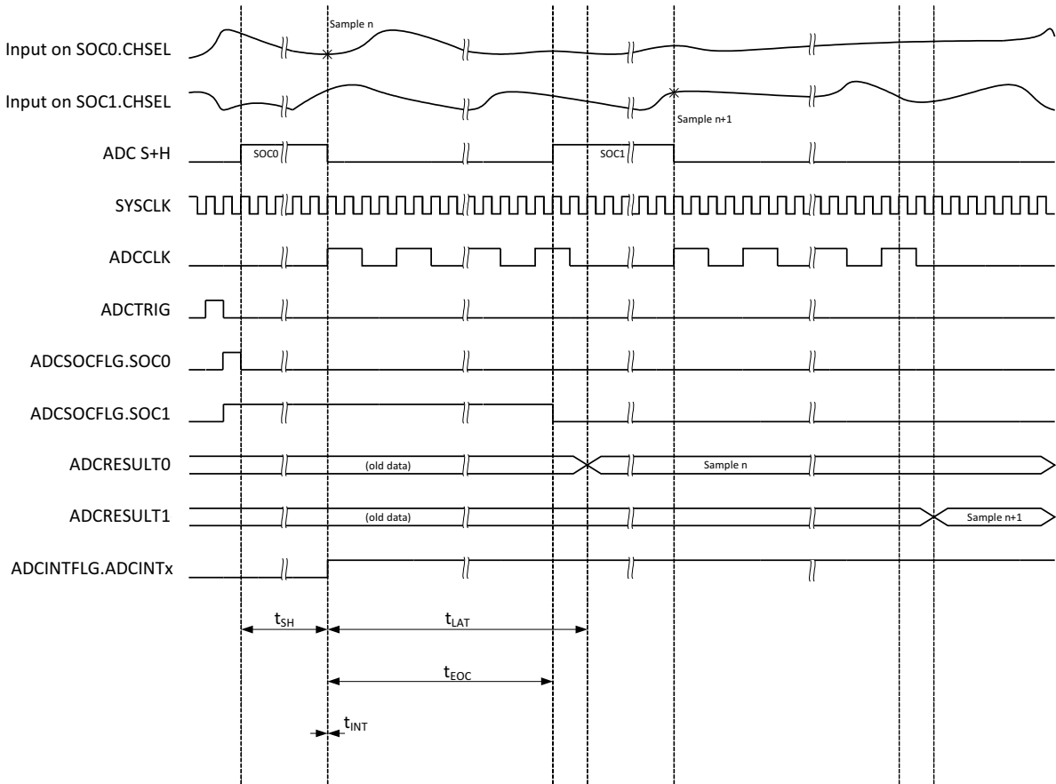
图 6-46. 提前中断模式下 12 位模式的 ADC 时序
