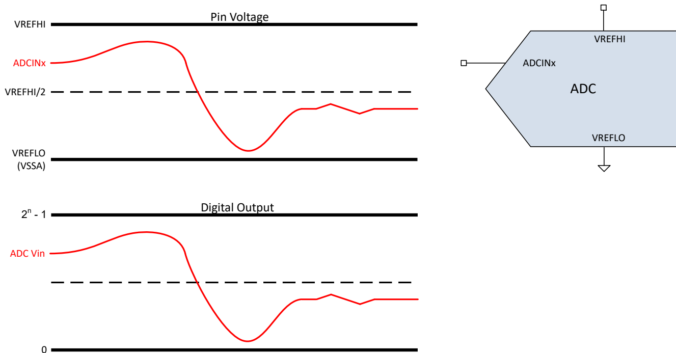
图 6-38. 单端信号模式
