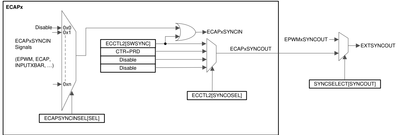
图 6-64. eCAP 同步方案
