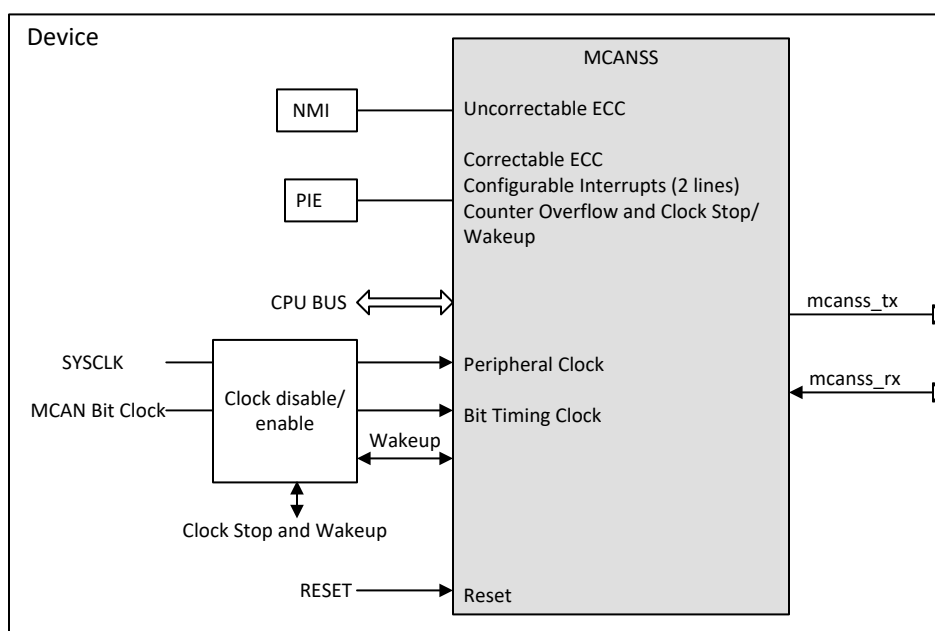
图 6-68. MCAN 模块概述
