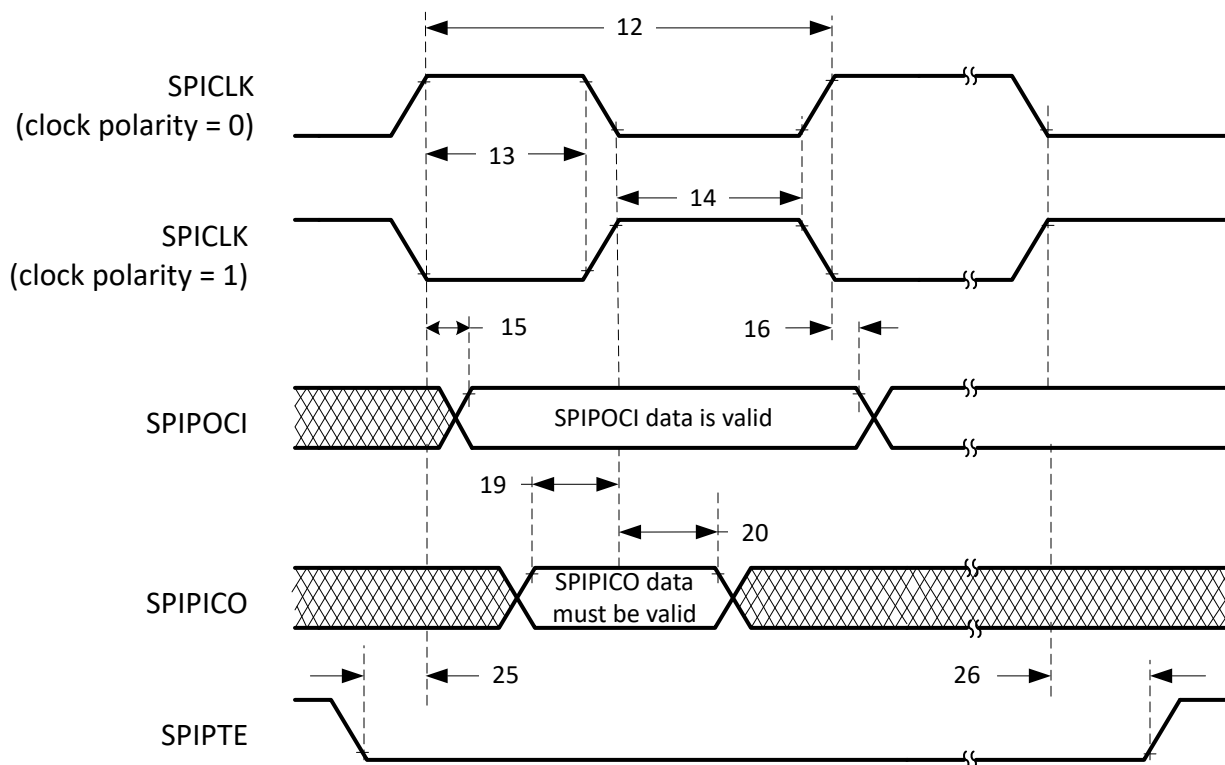
图 6-76. SPI 外设模式外部时序 (时钟相位 = 0)
