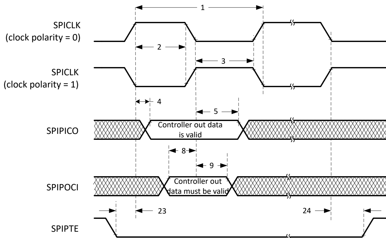
图 6-74. SPI 控制器模式外部时序 (时钟相位 = 0)
