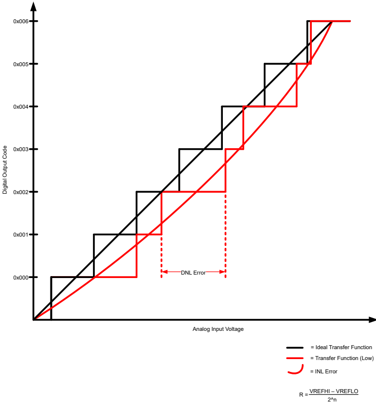
图 6-39. ADC INL 和 DNL
