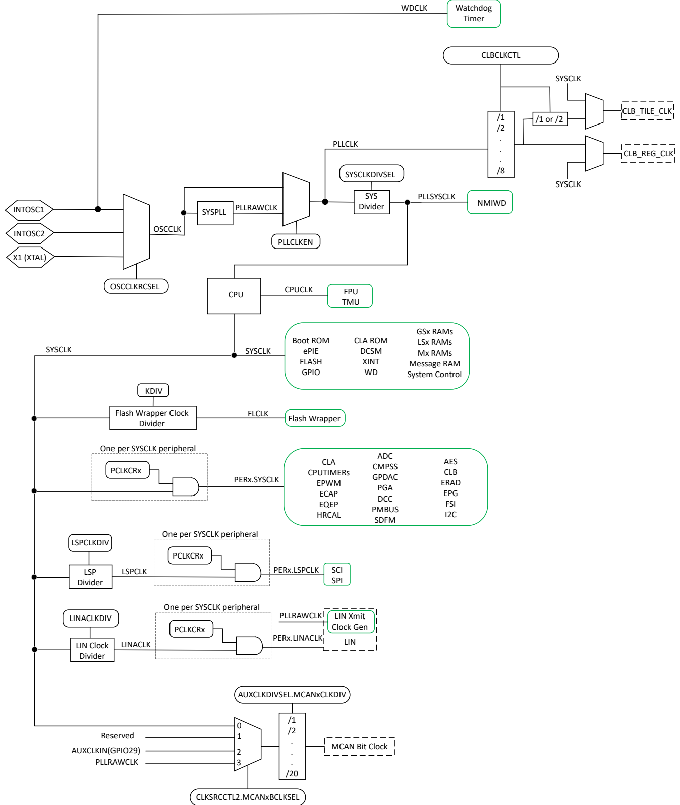
图 6-11. 计时系统
