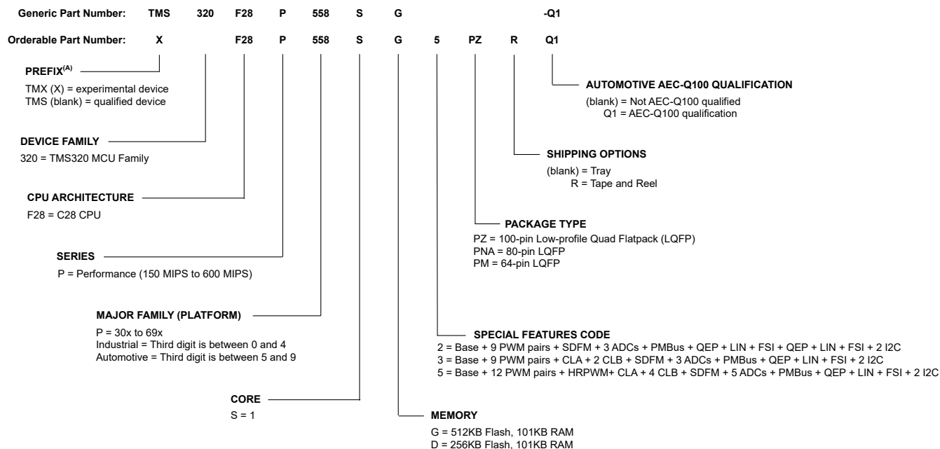
图 9-1. 器件命名规则 P558
