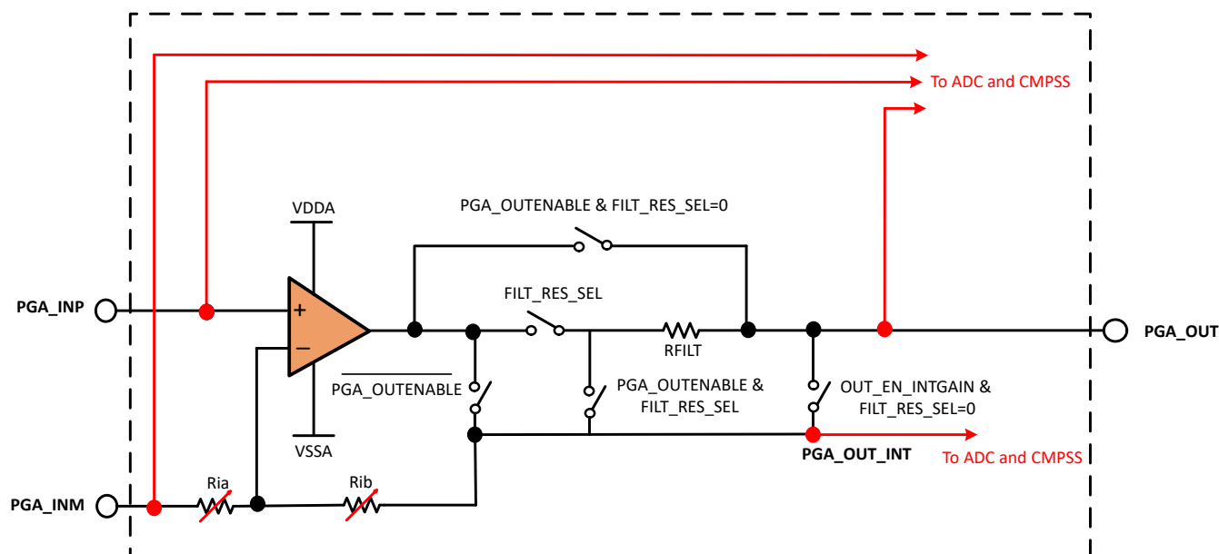
图 6-57. PGA 方框图
