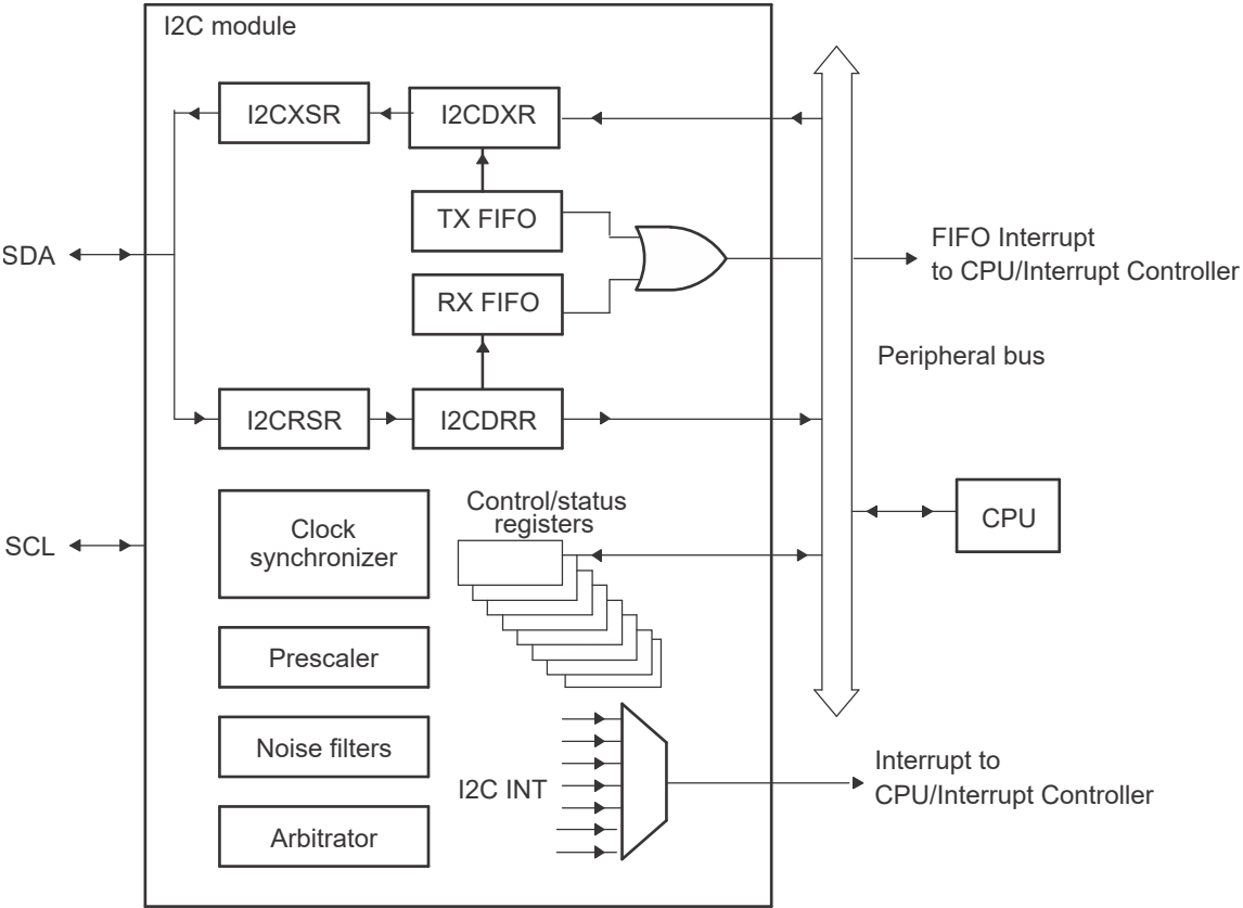
图 6-69. I2C 外设模块接口
