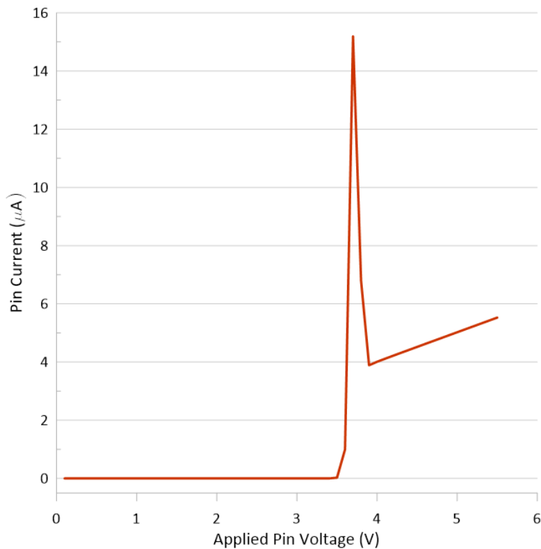
图 6-3. 漏电流与输入电压间的关系 ( 器件已通电 )
