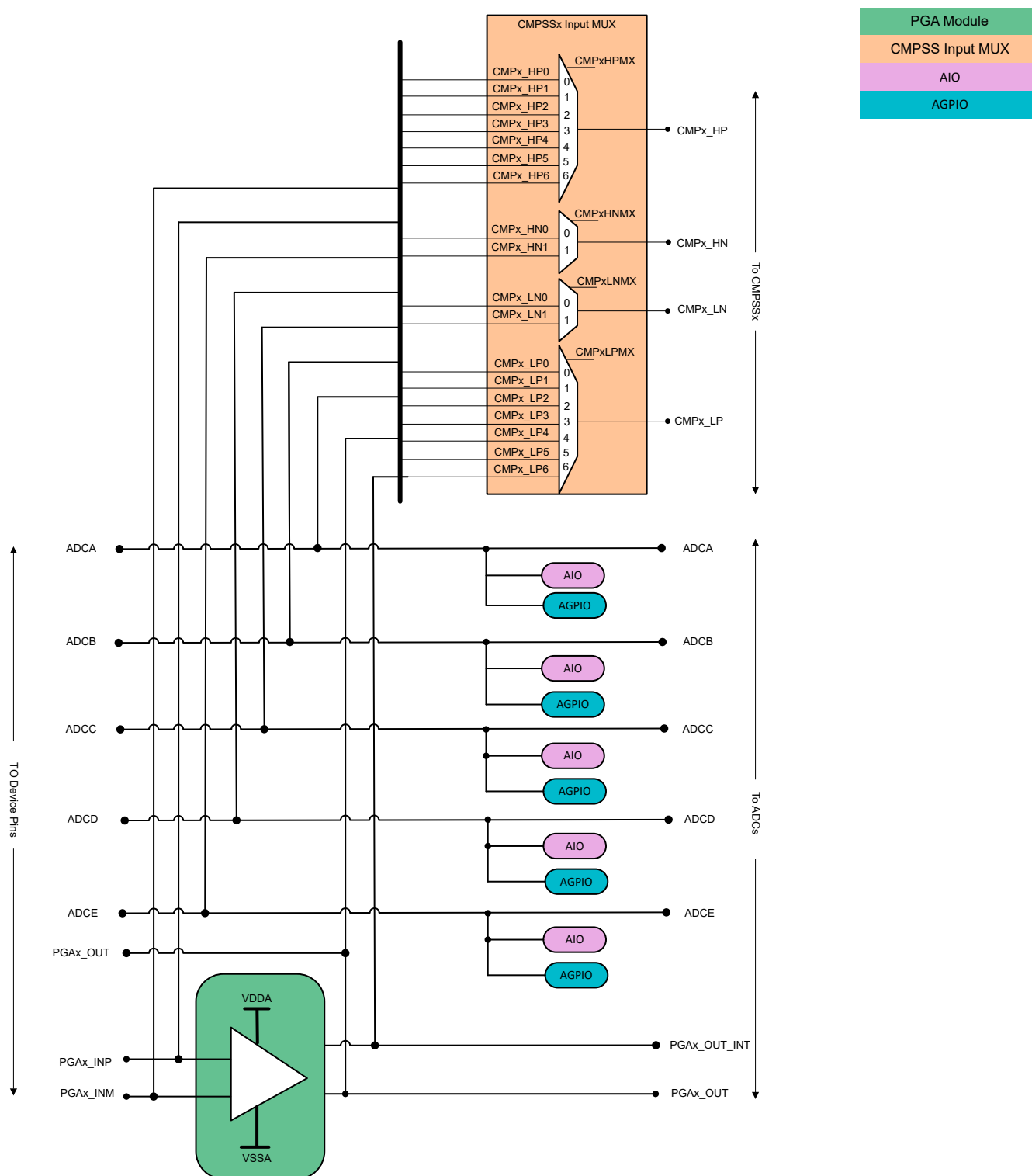
图 6-36. 模拟组连接
