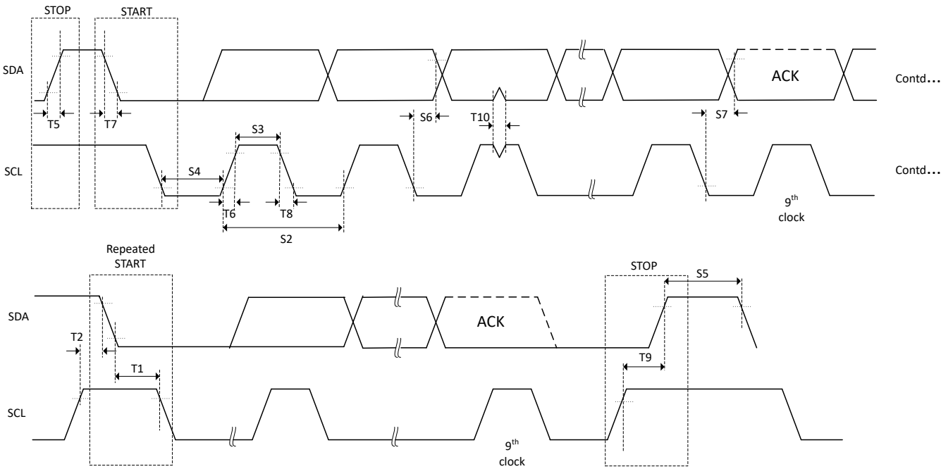
图 6-70. I2C 时序图
