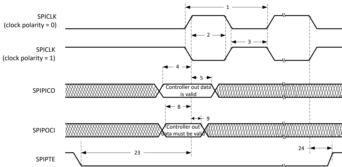
图 6-74. SPI 控制器模式外部时序 (时钟相位 = 0)
