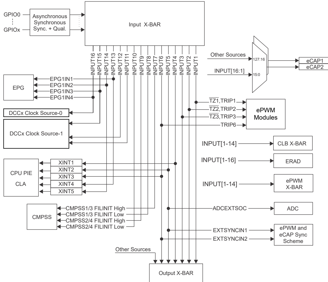
图 5-9. 输入 X-BAR
