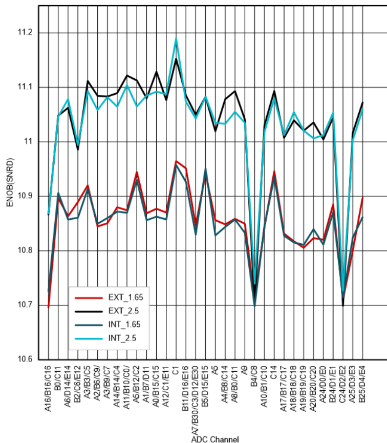
图 6-40. 100 引脚 PZ 的每通道 ENOB
