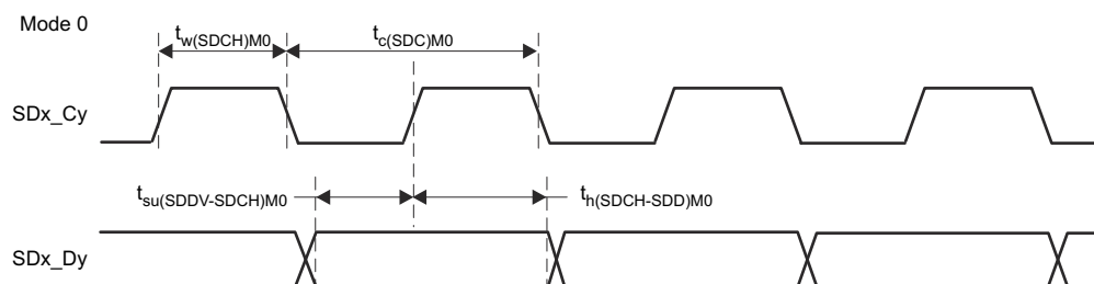
图 6-67. SDFM 时序图 - 模式 0
