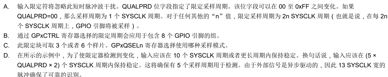
图 6-27. 采样模式
