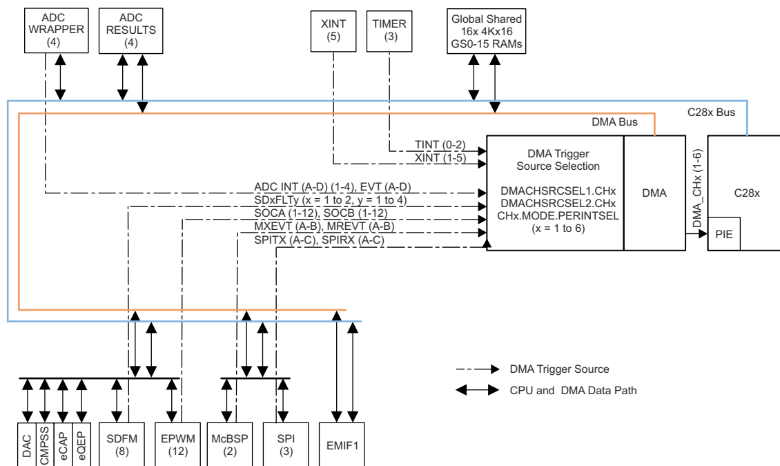
图 7-3. DMA 方框图
