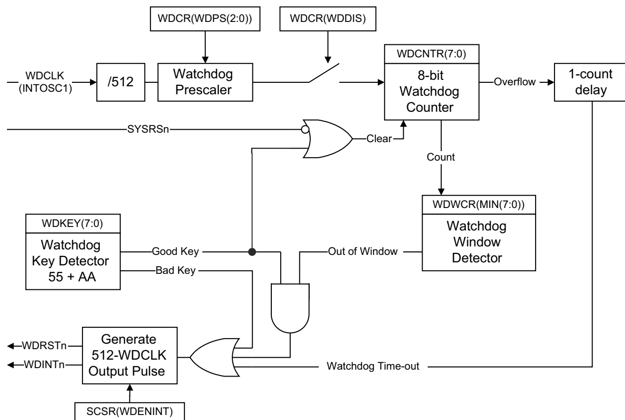
图 7-5. 窗口看门狗
